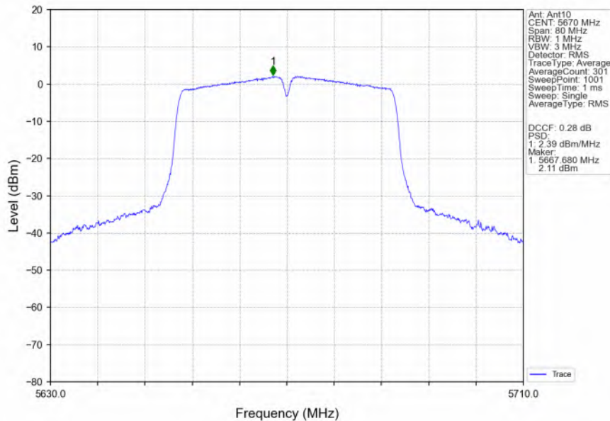
802.11n(HT40)_HCH_5670MHz_Ant10_NTNV
