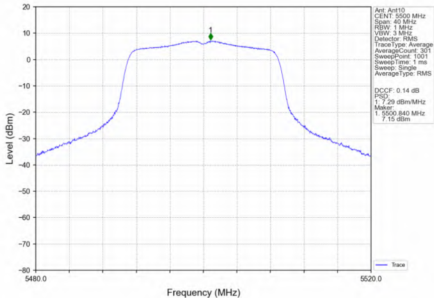
802.11ac(VHT20)_LCH_5500MHz_Ant10_NTNV
