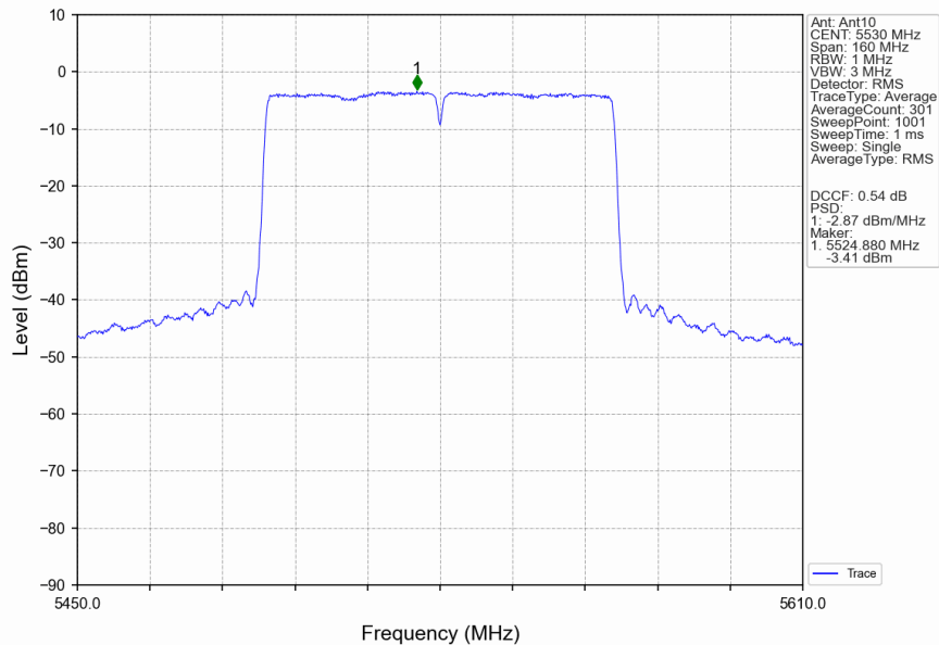
802.11ac(VHT80)_LCH_5530MHz_Ant10_NTNV
