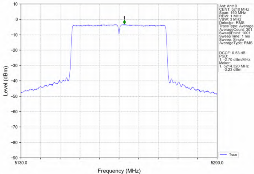
802.11ac(VHT80)_MCH_5210MHz_Ant10_NTNV
