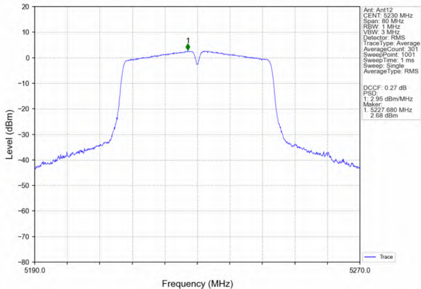
802.11n(HT40)_HCH_5230MHz_Ant12_NTNV
