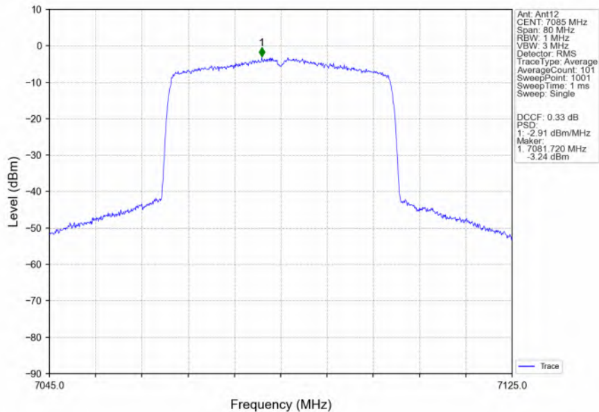
802.11ax(HEW40)_HCH_7085MHz_RU484_Left_Ant12_NTNV
