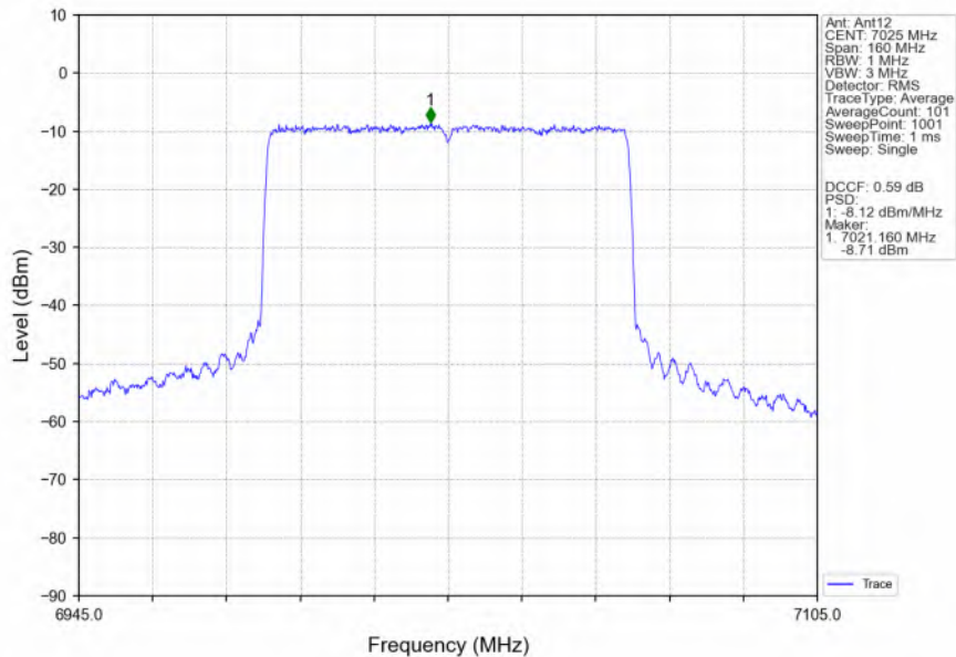
802.11ax(HEW80)_HCH_7025MHz_RU996_Left_Ant12_NTNV
