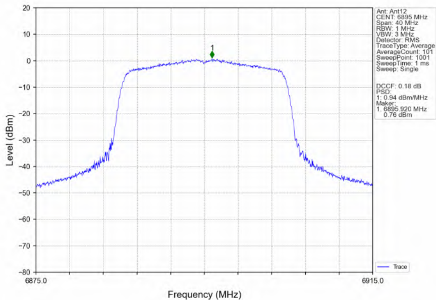
802.11ax(HEW20)_LCH_6895MHz_RU242_Left_Ant12_NTNV
