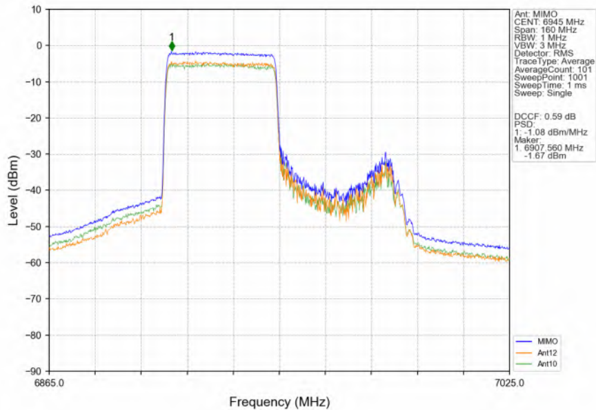
802.11ax(HEW80)_LCH_6945MHz_RU996_Left_Ant12_NTNV
