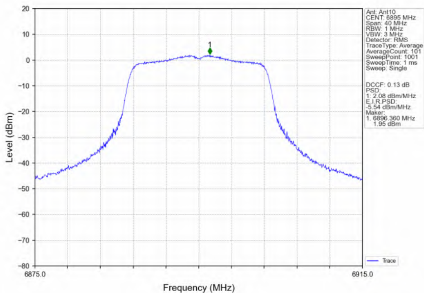
802.11a_LCH_6895MHz_Ant10_NTNV
