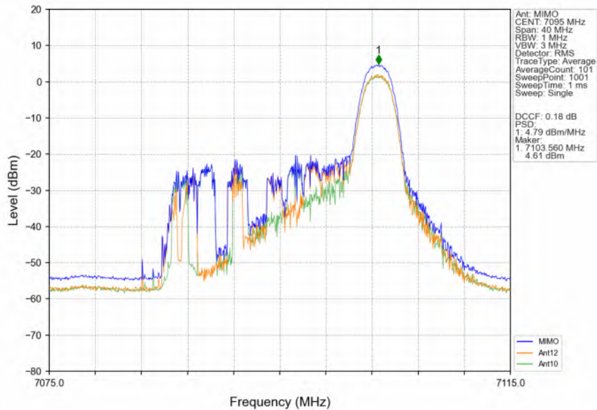
802.11ax(HEW20)_HCH_7095MHz_RU52_Right_Ant12_NTNV
