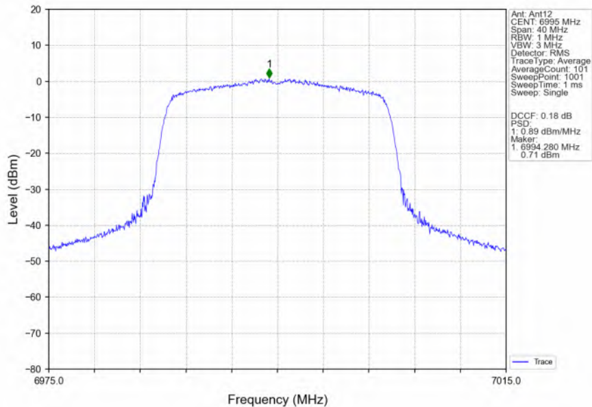
802.11ax(HEW20)_MCH_6995MHz_RU242_Left_Ant12_NTNV
