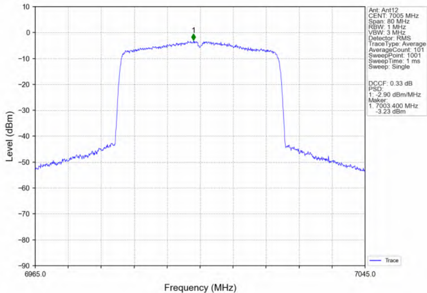
802.11ax(HEW40)_MCH_7005MHz_RU484_Left_Ant12_NTNV
