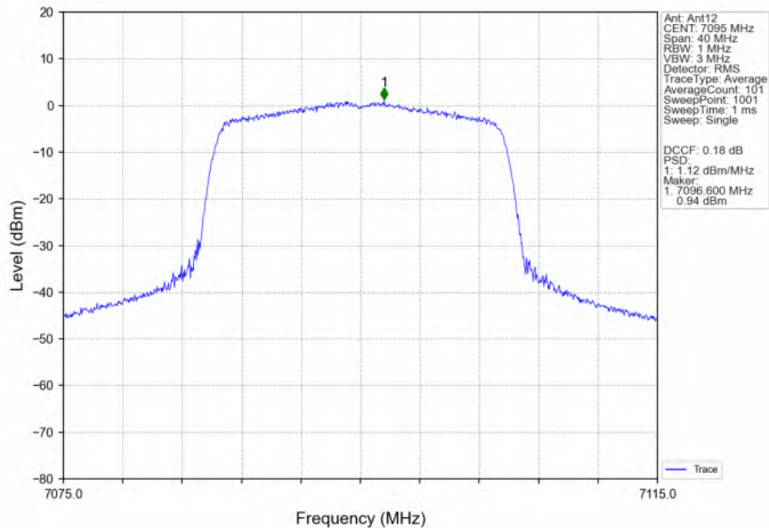
802.11ax(HEW20)_HCH_7095MHz_RU242_Left_Ant12_NTNV
