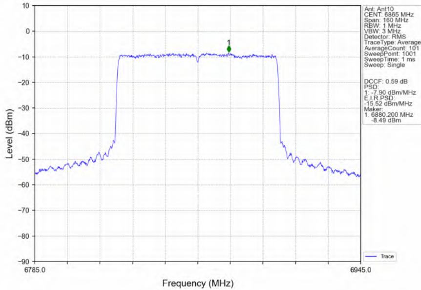
802.11ax(HEW80)_HCH_6865MHz_RU996_Left_MIMO_NTNV
