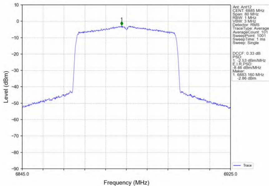
802.11ax(HEW40)_HCH_6885MHz_RU484_Left_Ant12_NTNV
