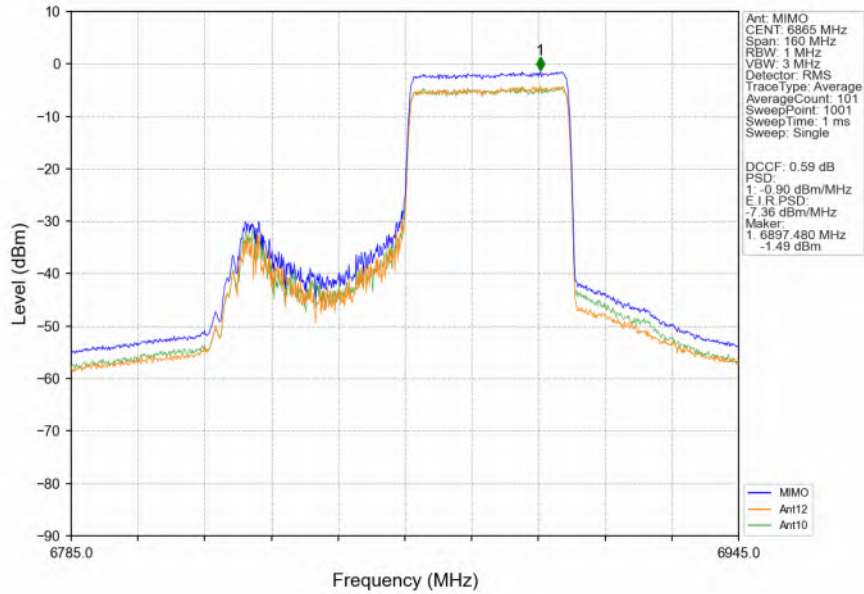
802.11ax(HEW80)_HCH_6865MHz_RU996_Left_Ant12_NTNV
