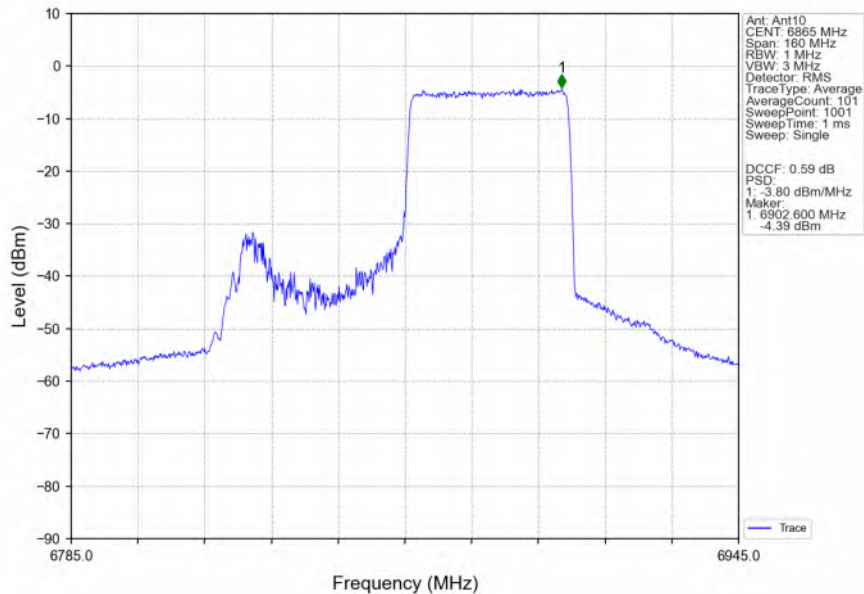
802.11ax(HEW80)_HCH_6865MHz_RU484_Right_Ant10_NTNV
