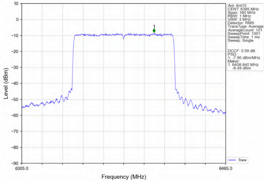
802.11ax(HEW80)_HCH_6385MHz_RU996_Left_MIMO_NTNV
