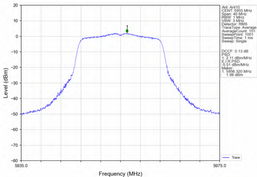
802.11a_LCH_5955MHz_Ant10_NTNV
