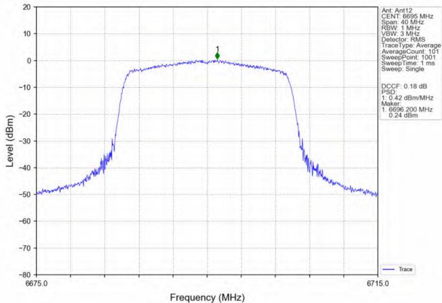
802.11ax(HEW20)_MCH_6695MHz_RU242_Left_Ant12_NTNV
