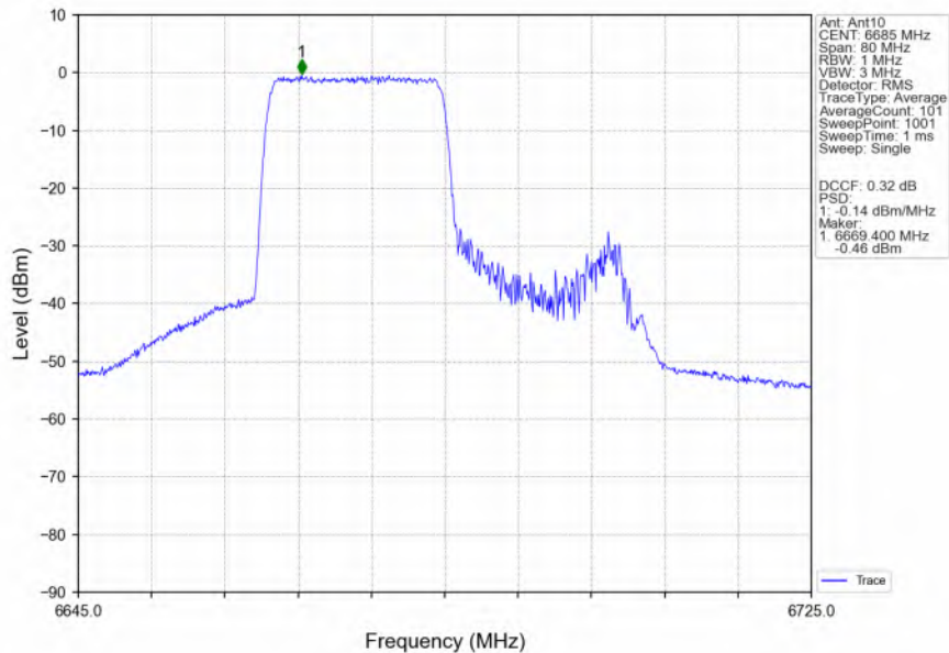
802.11ax(HEW40)_MCH_6685MHz_RU242_Left_Ant10_NTNV
