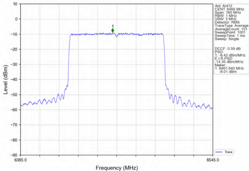
802.11ax(HEW80)_LCH_6465MHz_RU996_Left_Ant12_NTNV
