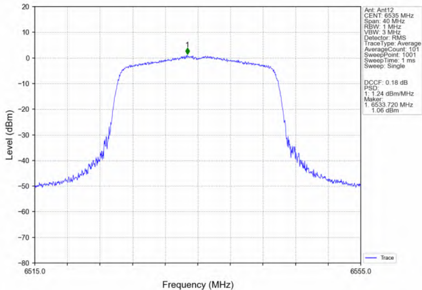
802.11ax(HEW20)_LCH_6535MHz_RU242_Left_Ant12_NTNV
