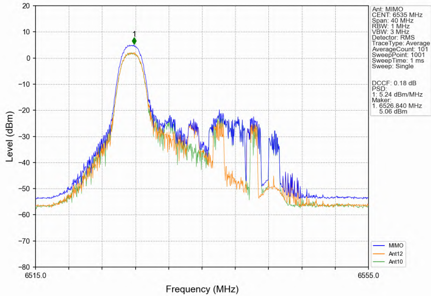
802.11ax(HEW20)_LCH_6535MHz_RU52_Left_Ant12_NTNV
