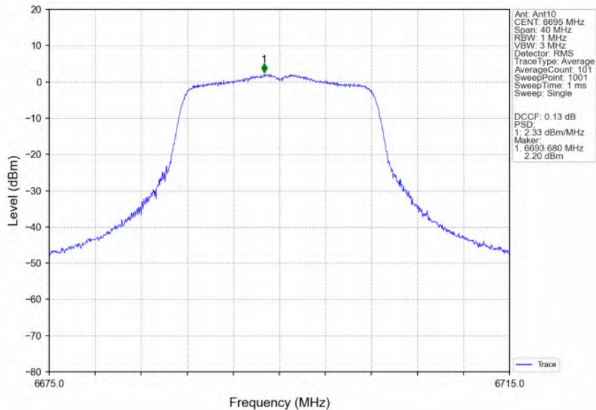
802.11a_MCH_6695MHz_Ant10_NTNV
