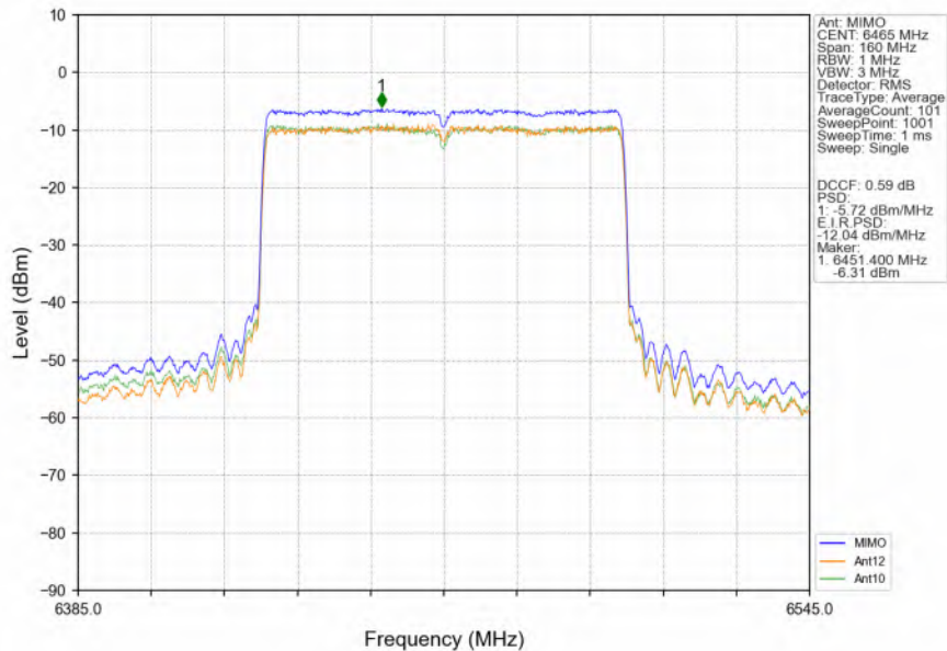
802.11ax(HEW80)_LCH_6465MHz_RU996_Left_MIMO_NTNV
