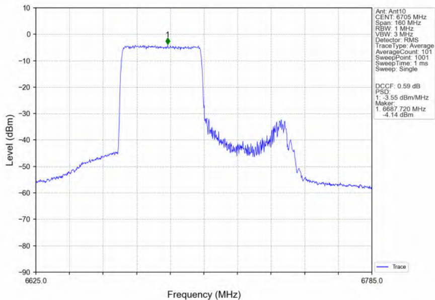
802.11ax(HEW80)_MCH_6705MHz_RU484_Left_Ant10_NTNV
