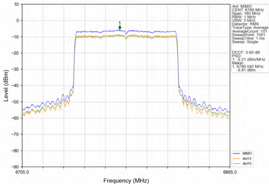
802.11ax(HEW80)_HCH_6785MHz_RU996_Left_MIMO_NTNV
