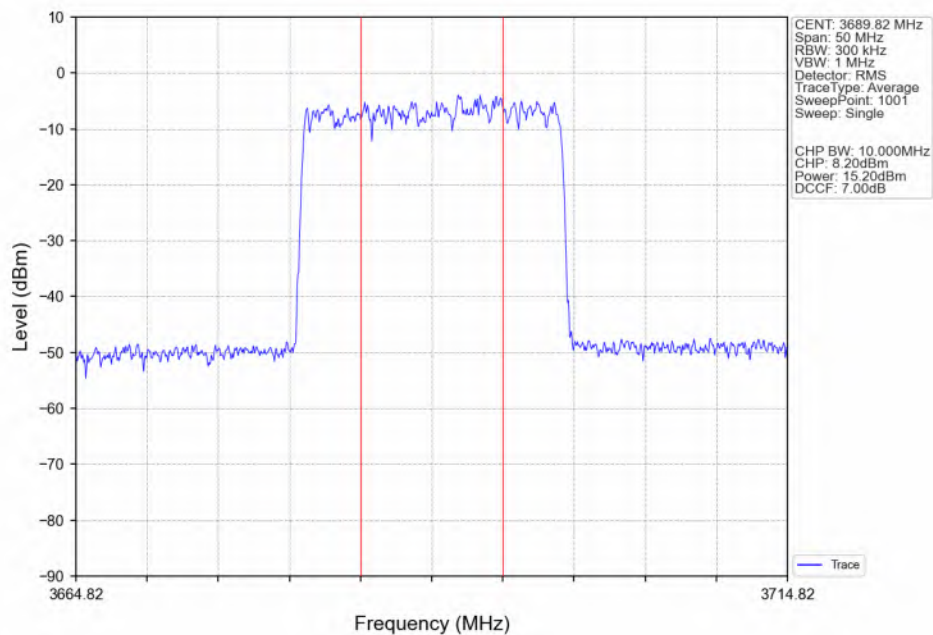
n48_30kHz_SISO_NTNV_20MHz_DFT-s-OFDM_256_QAM_3690MHz_Inner_Full_Ant4
