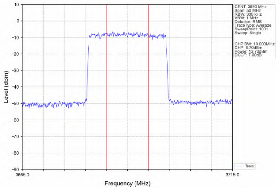
n48_30kHz_SISO_NTNV_20MHz_CP-OFDM_256_QAM_3690MHz_Inner_Full_Ant4
