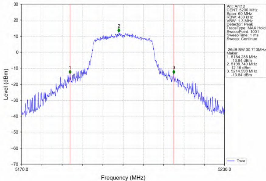
802.11n(HT20)_MCH_5200MHz_Ant12_NTNV
