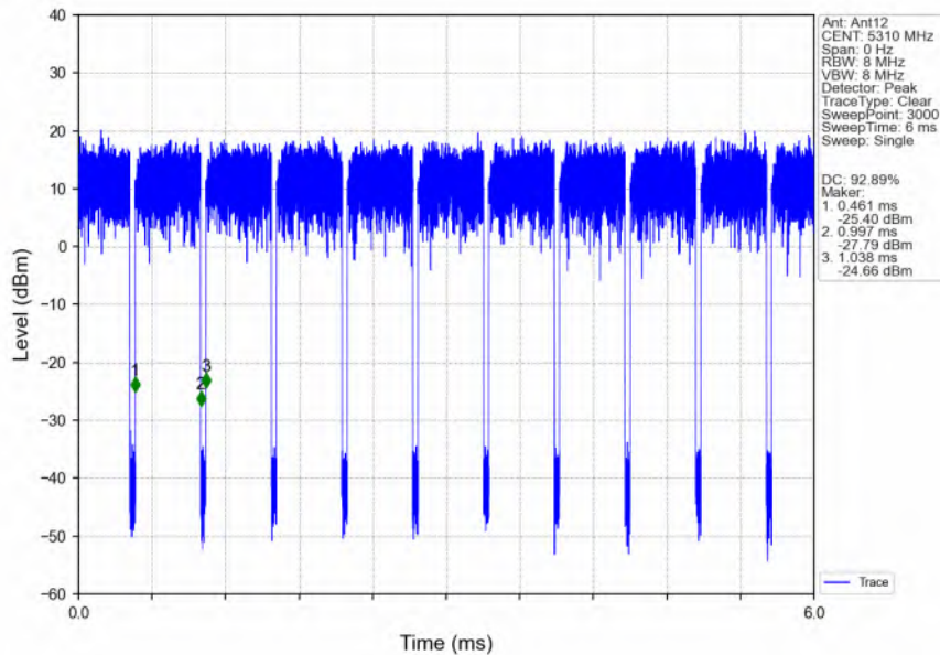
802.11ax(HEW40)_HCH_5310MHz_RU484_Left_Ant12_NTNV
