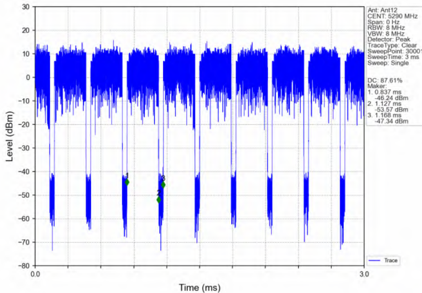
802.11ax(HEW80)_MCH_5290MHz_RU996_Left_Ant12_NTNV
