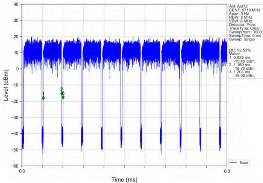
802.11ax(HEW40)_HCH_5710MHz_RU484_Left_Ant12_NTNV
