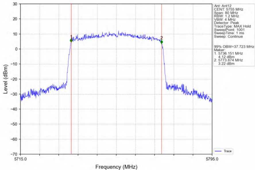
802.11ax(HEW40)_LCH_5755MHz_RU484_Left_Ant12_NTNV
