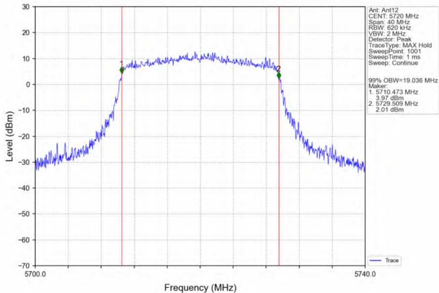
802.11ax(HEW20)_HCH_5720MHz_RU242_Left_Ant12_NTNV
