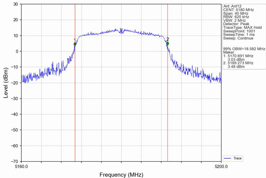
802.11n(HT20)_LCH_5180MHz_Ant12_NTNV
