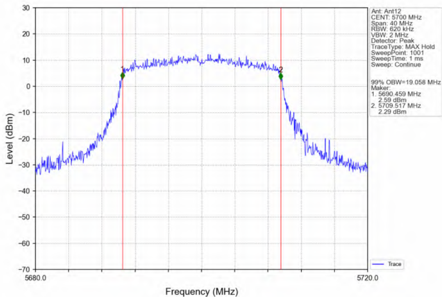
802.11ax(HEW20)_HCH_5700MHz_RU242_Left_Ant12_NTNV
