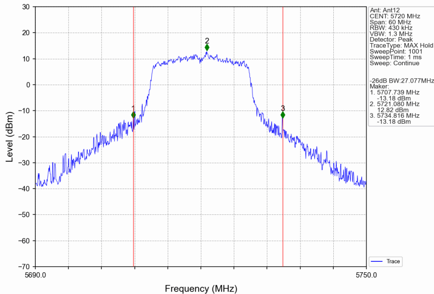
802.11n(HT20)_HCH_5720MHz_Ant12_NTNV
