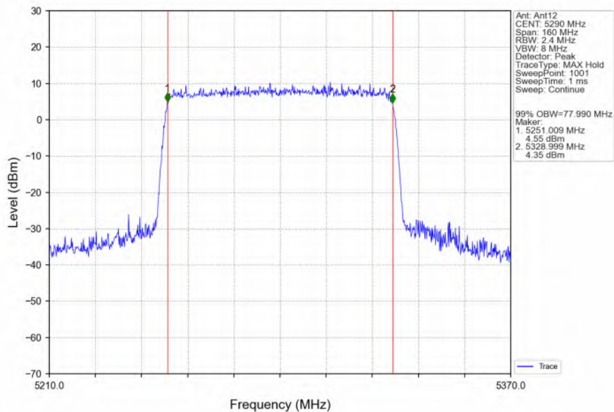
802.11ax(HEW80)_MCH_5290MHz_RU996_Left_Ant12_NTNV
