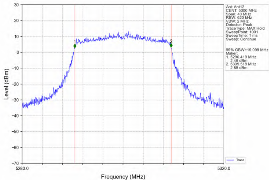
802.11ax(HEW20)_MCH_5300MHz_RU242_Left_Ant12_NTNV
