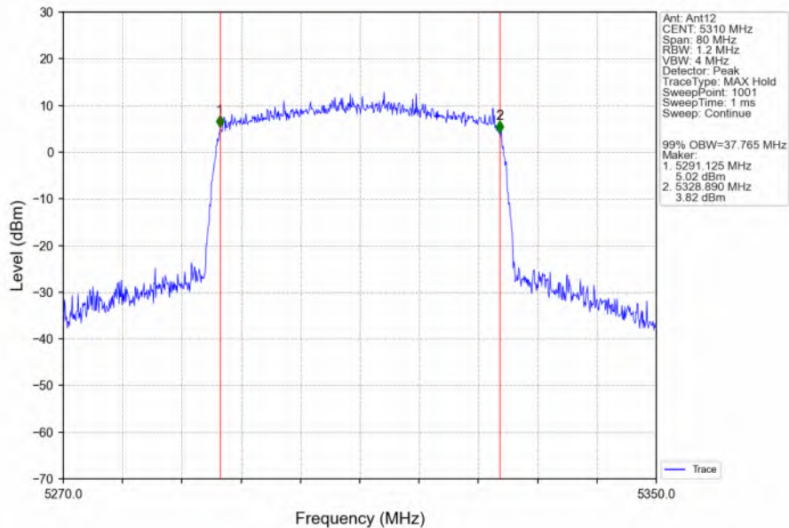
802.11ax(HEW40)_HCH_5310MHz_RU484_Left_Ant12_NTNV
