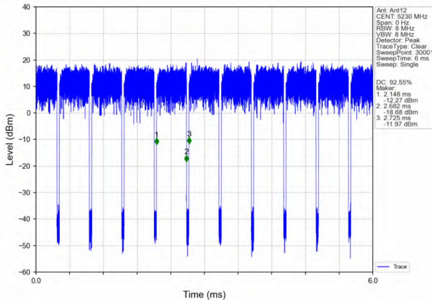
802.11ax(HEW40)_HCH_5230MHz_RU484_Left_Ant12_NTNV
