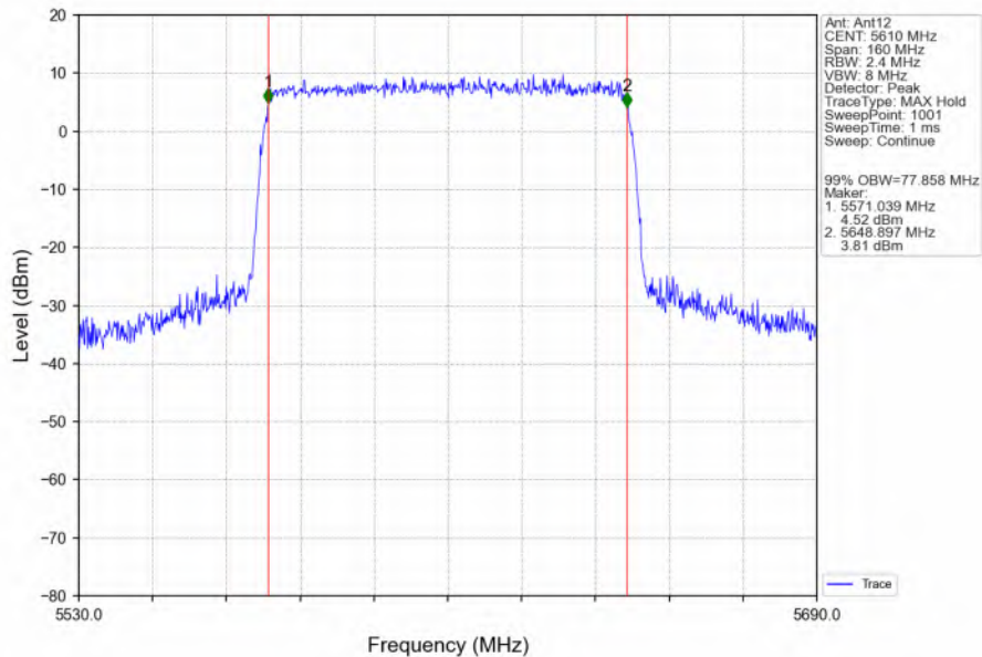
802.11ax(HEW80)_HCH_5610MHz_RU996_Left_Ant12_NTNV
