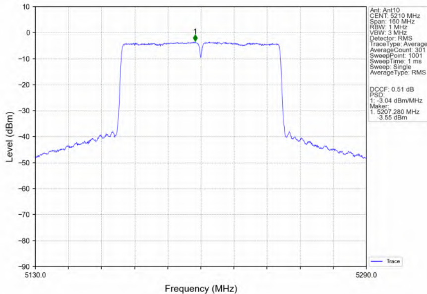
802.11ac(VHT80)_MCH_5210MHz_Ant10_NTNV
