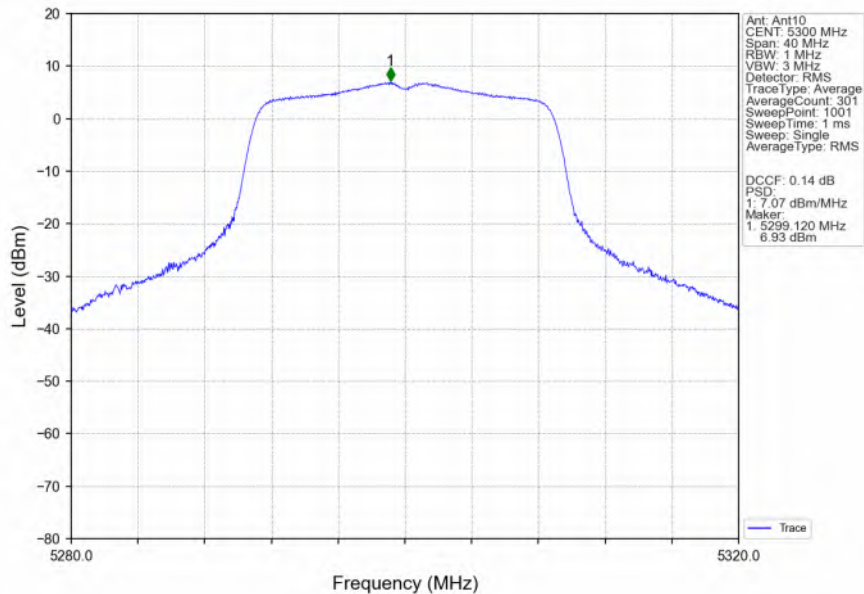
802.11n(HT20)_MCH_5300MHz_Ant10_NTNV
