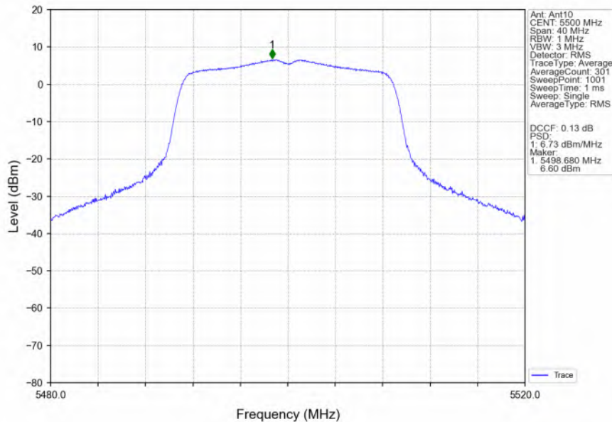
802.11ac(VHT20)_LCH_5500MHz_Ant10_NTNV
