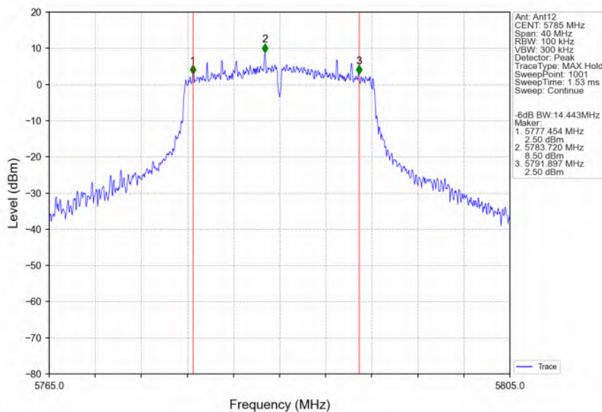
802.11a_MCH_5785MHz_Ant12_NTNV
