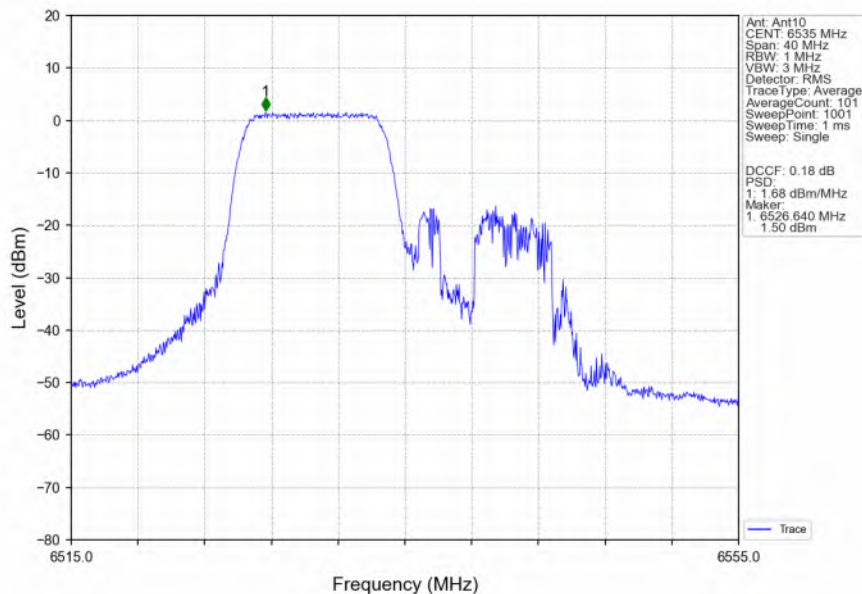
802.11ax(HEW20) LCH 6535MHz RU106 Left_Ant10 NTN
