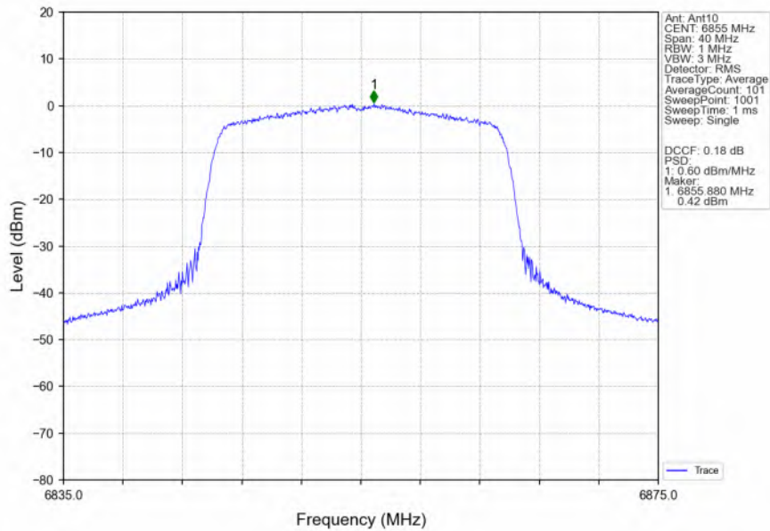
802.11ax(HEW20) HCH 6855MHz RU242 Left MIMO NTNW
