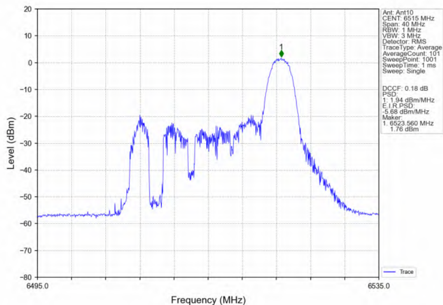
802.11ax(HEW20) HCH 6515MHz RU26 Right Ant10 NTNV
