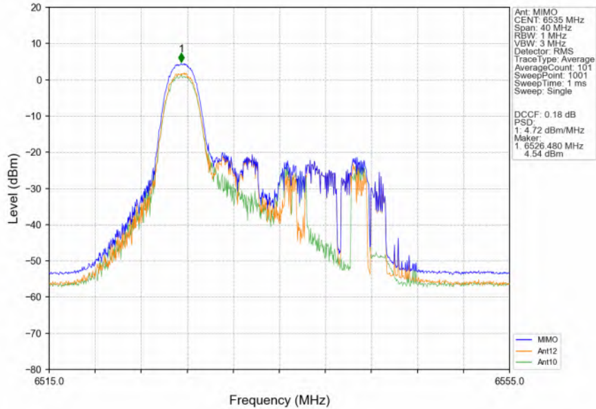
802.11ax(HEW20)_LCH_6535MHz_RU52_Left_Ant12_NTNV
