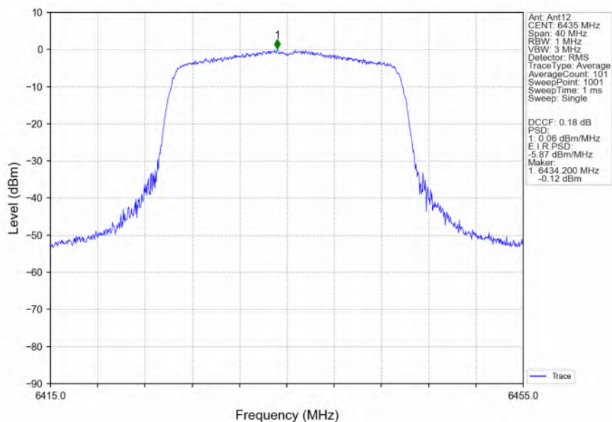
802.11ax(HEW20) LCH 6435MHz RU242 Left Ant12 NTN
