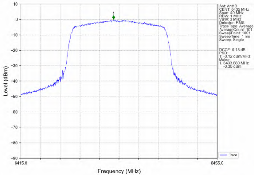
802.11ax(HEW20) LCH 6435MHz RU242 Left MIMO NTN
