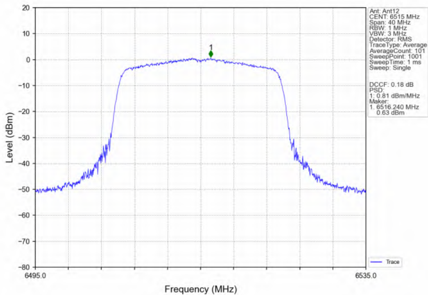
802.11ax(HEW20) HCH 6515MHz RU242 Left Ant12 NTN
