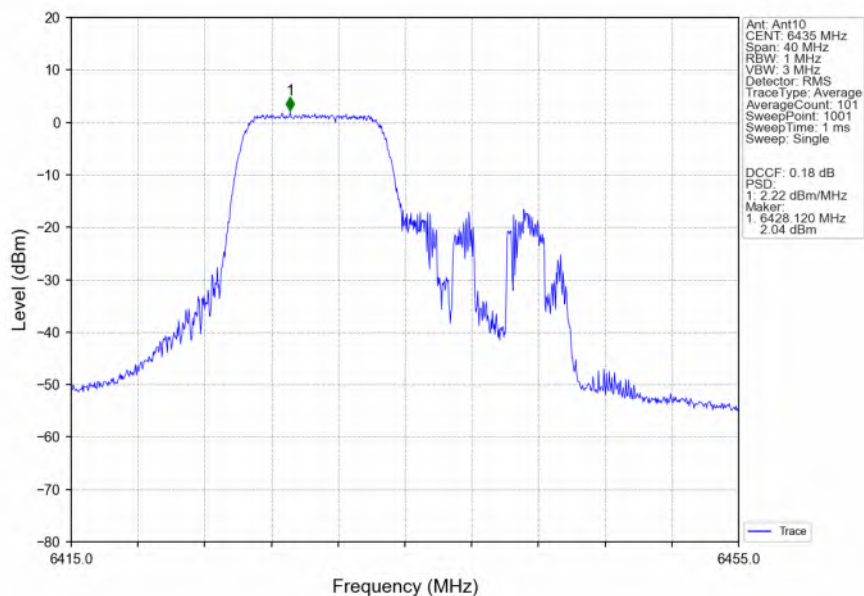
802.11ax(HEW20) LCH 6435MHz RU106 Left_Ant10 NTNW
