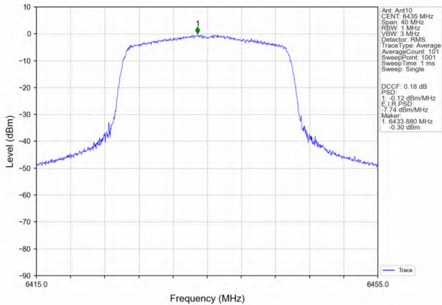
802.11ax(HEW20) LCH 6435MHz RU242 Left MIMO NTNv
