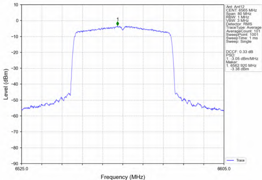
802.11ax(HEW40) LCH 6565MHz RU484 Left Ant12 NTNW
