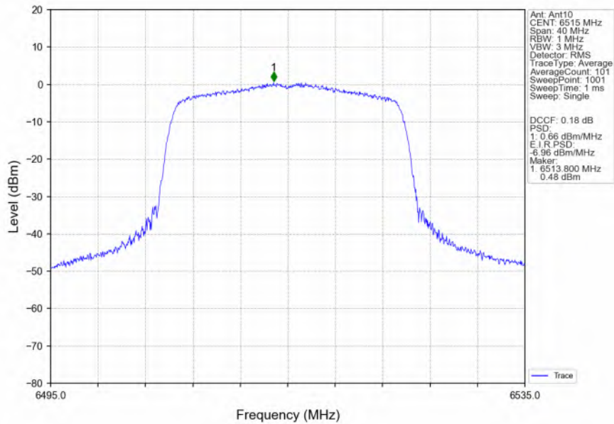
802.11ax(HEW20) HCH 6515MHz RU242 Left MIMO NTN
