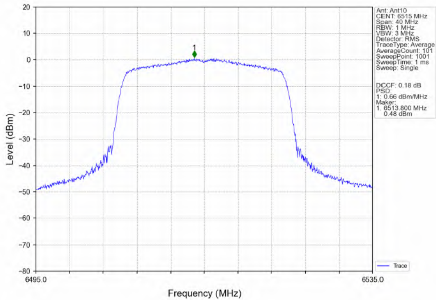
802.11ax(HEW20) HCH 6515MHz RU242 Left MIMO NTNW
