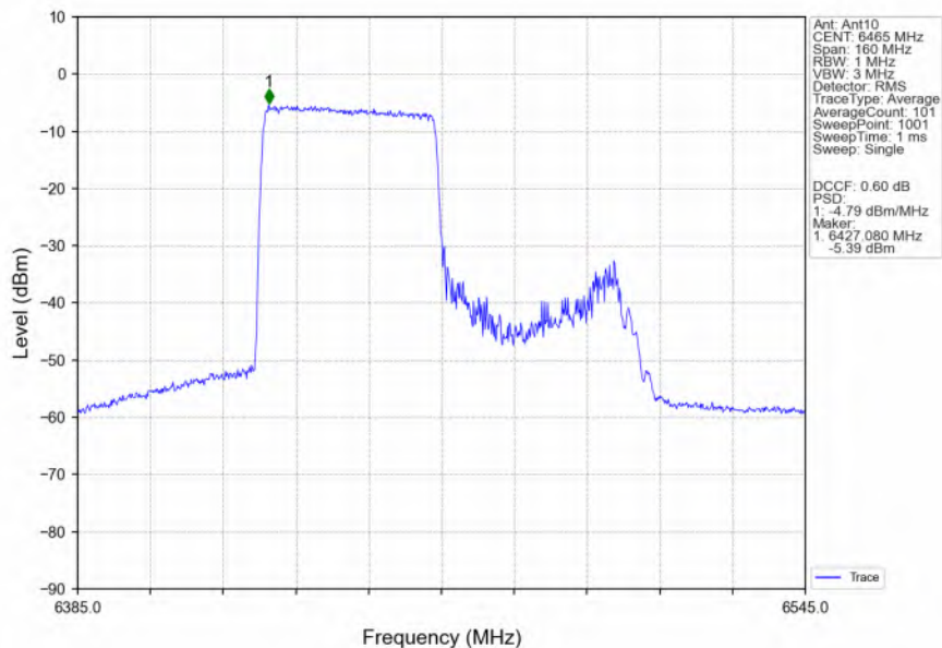
802.11ax(HEW80) LCH 6465MHz RU484 Left_Ant10 NTNW
