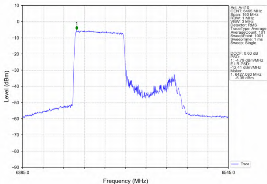
802.11ax(HEW80) LCH 6465MHz RU484 Left Ant10 NTN
