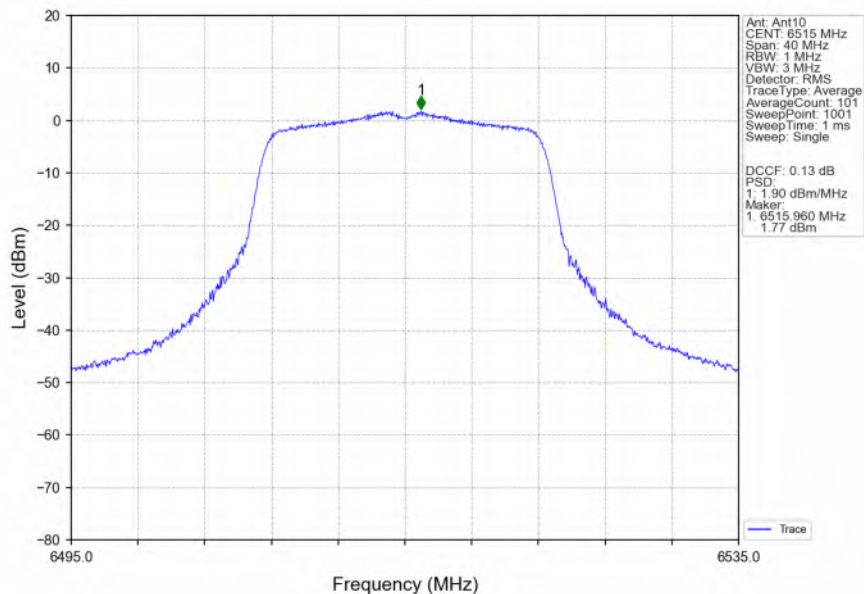
802.11a_HCH_6515MHz_Ant10_NTNV
