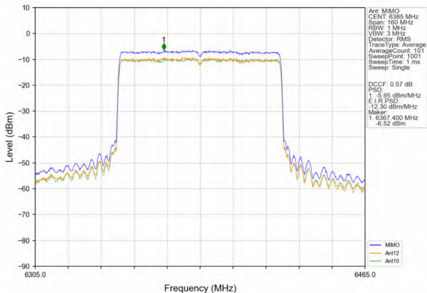
802.11ax(HEW80) HCH 6385MHz RU996 Left MIMO NTN
