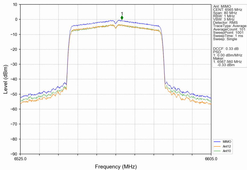
802.11ax(HEW40) LCH 6565MHz RU484 Left MIMO NTNv
