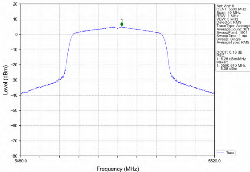
802.11ax(HEW20)_LCH_5500MHz_RU242_Left_Ant10_NTNV
