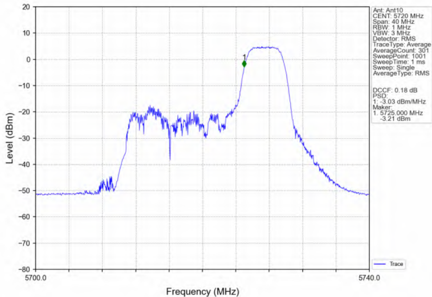
802.11ax(HEW20)_HCH_5720MHz_RU52_Right_Ant10_NTNV
