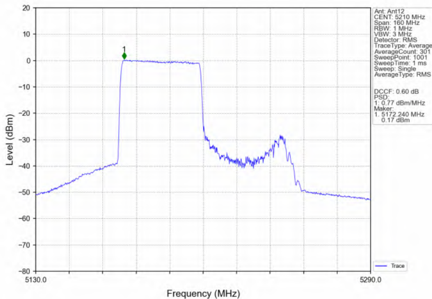
802.11ax(HEW80)_MCH_5210MHz_RU484_Left_Ant12_NTNV
