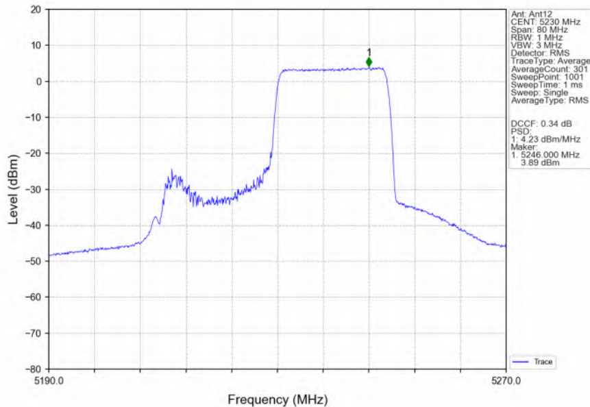
802.11ax(HEW40)_HCH_5230MHz_RU242_Right_Ant12_NTNV
