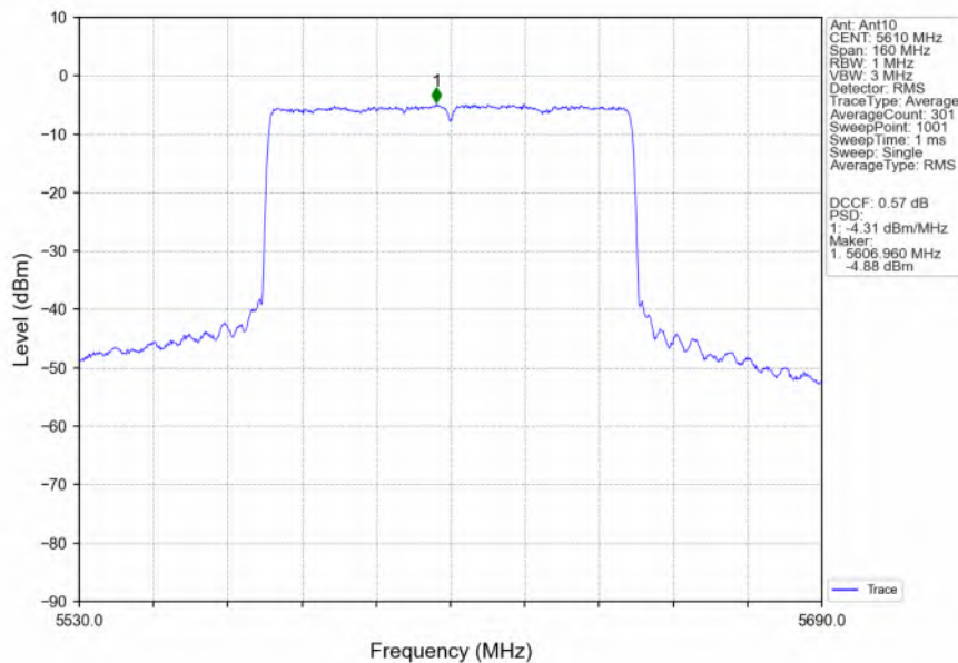
802.11ax(HEW80)_HCH_5610MHz_RU996_Left_Ant10_NTNV
