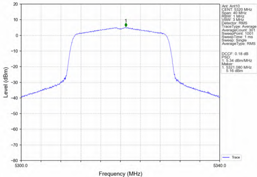
802.11ax(HEW20)_HCH_5320MHz_RU242_Left_Ant10_NTNV
