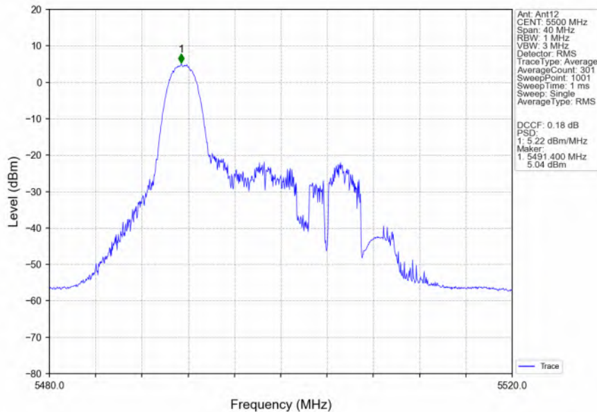
802.11ax(HEW20)_LCH_5500MHz_RU26_Left_Ant12_NTNV
