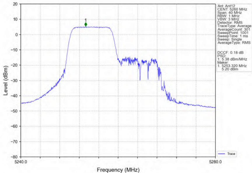
802.11ax(HEW20)_LCH_5260MHz_RU106_Left_Ant12_NTNV
