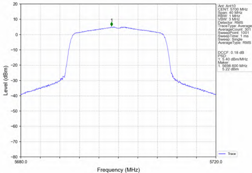
802.11ax(HEW20)_HCH_5700MHz_RU242_Left_Ant10_NTNV
