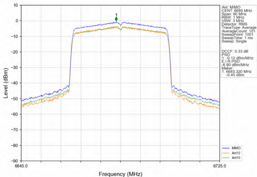
802.11ax(HEW40) MCH_6685MHz RU484 Left MIMO NTN
