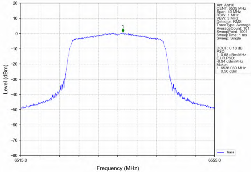
802.11ax(HEW20) LCH 6535MHz RU242 Left MIMO NTN
