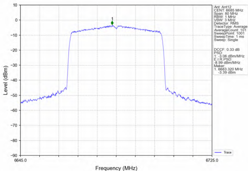
802.11ax(HEW40) MCH_6685MHz RU484 Left Ant12 NTN
