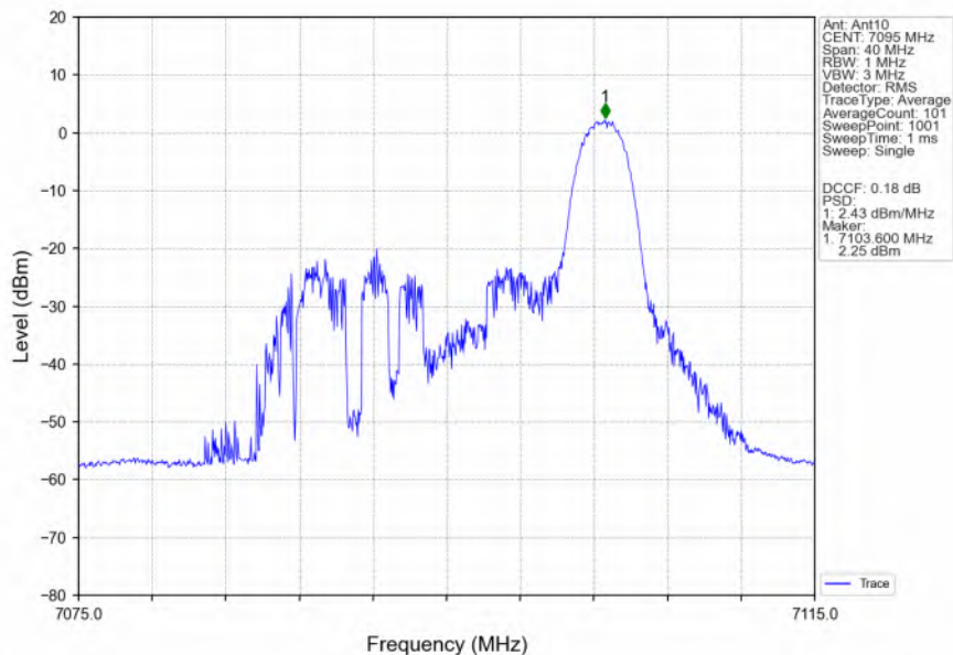
802.11ax(HEW20) HCH 7095MHz RU26 Right Ant10 NTNV
