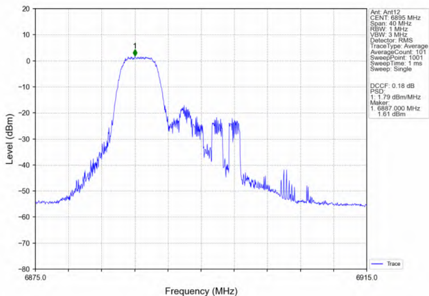
802.11ax(HEW20)_LCH_6895MHz_RU52_Left_Ant12_NTNV
