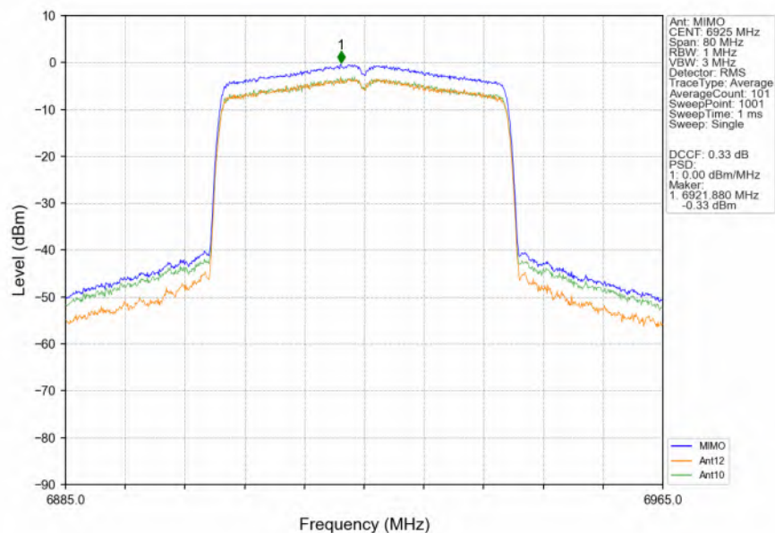
802.11ax(HEW40) LCH 6925MHz RU484 Left MIMO NTN
