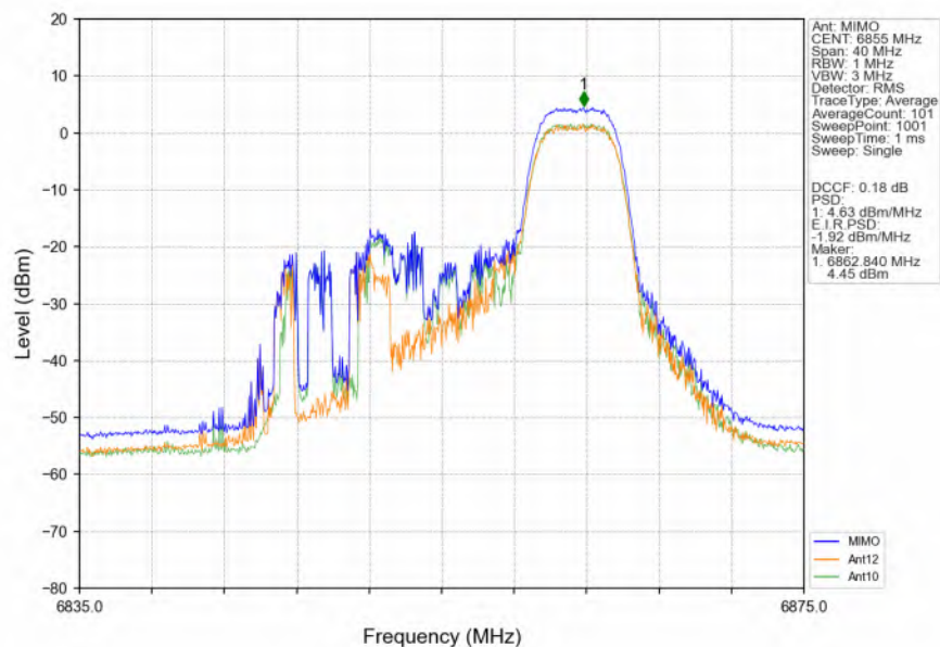
802.11ax(HEW20) HCH 6855MHz RU52 Right MIMO NTN
