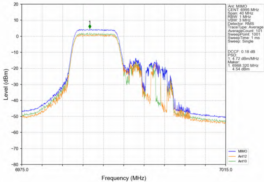
802.11ax(HEW20) MCH_6995MHz RU242 Left Ant12 NTNW
