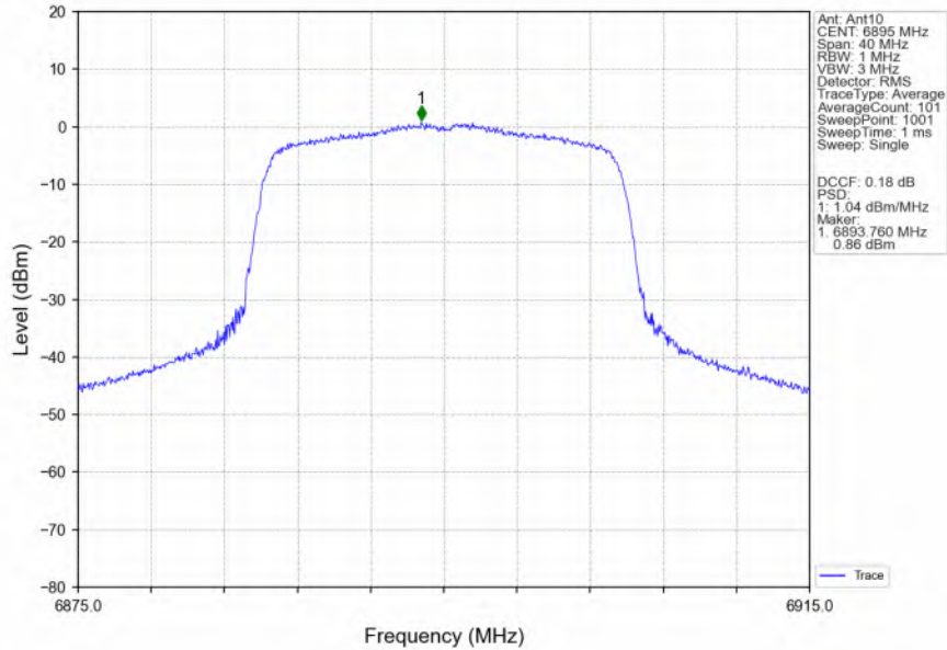
802.11ax(HEW20) LCH 6895MHz RU242 Left MIMO NTNW
