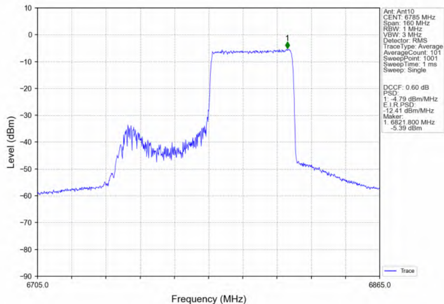
802.11ax(HEW80) HCH 6785MHz RU484 Right Ant10 NTN
