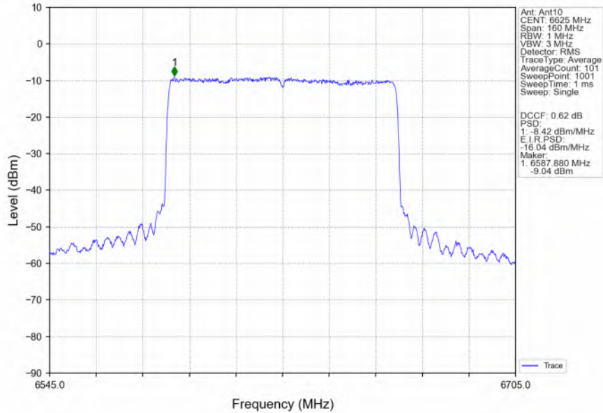
802.11ax(HEW80) LCH 6625MHz RU996 Left MIMO NTN
