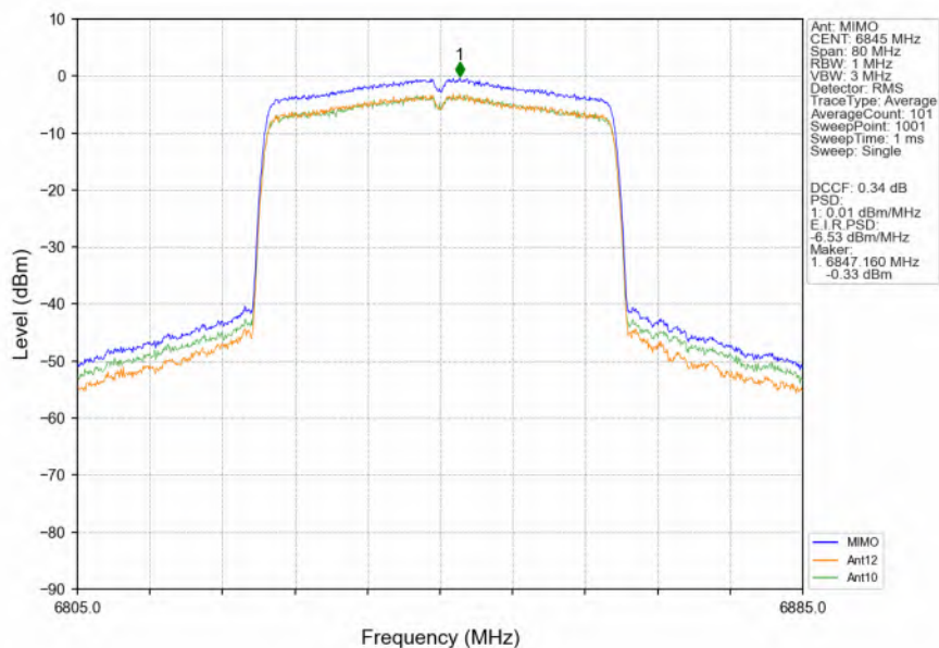
802.11ax(HEW40) HCH 6845MHz RU484 Left MIMO NTNW
