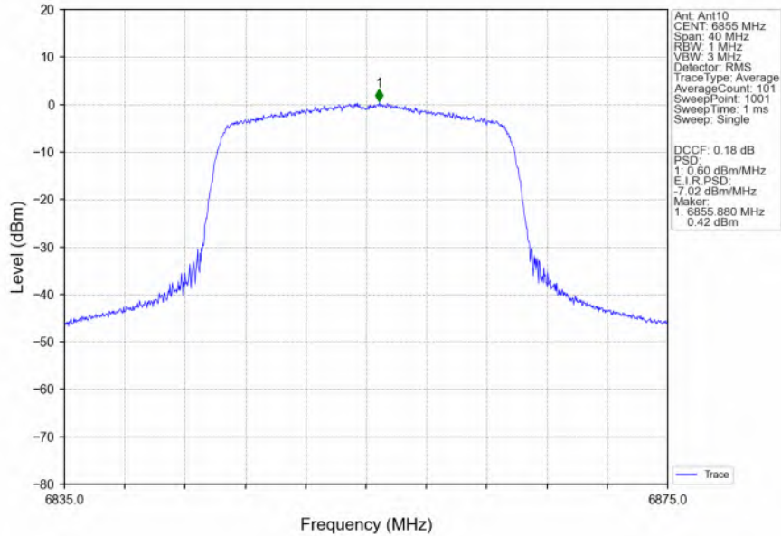
802.11ax(HEW20) HCH 6855MHz RU242 Left MIMO NTN
