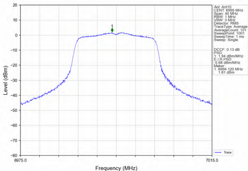
802.11a_MCH_6995MHz_Ant10_NTNV
