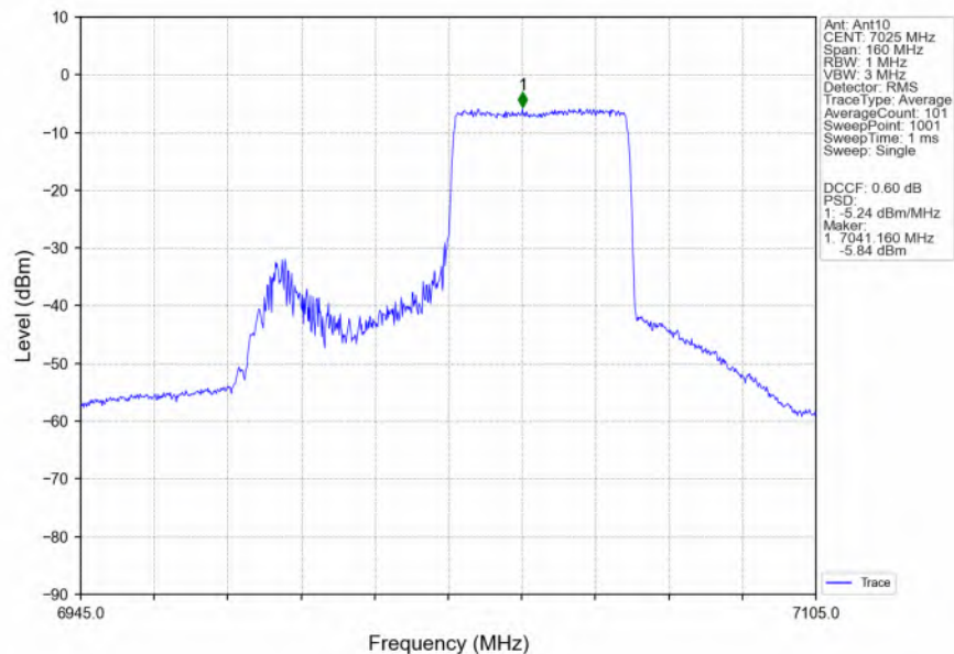
802.11ax(HEW80) HCH 7025MHz RU484 Right Ant10 NTN7
