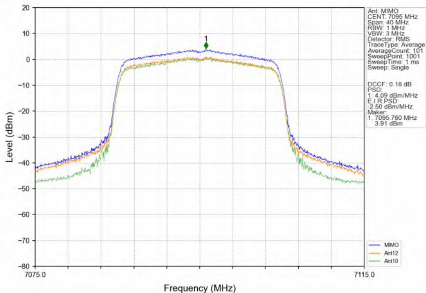
802.11ax(HEW20) HCH 7095MHz RU242 Left MIMO NTN
