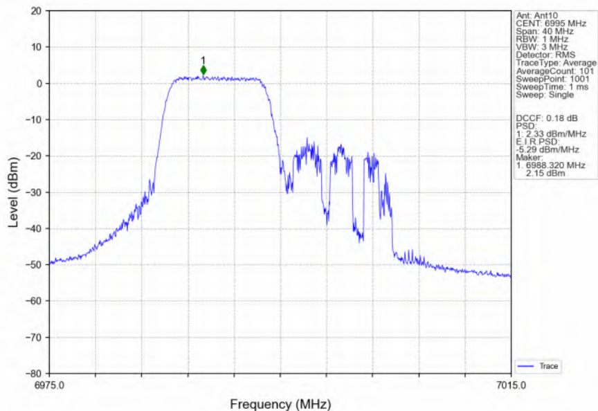
802.11ax(HEW20) MCH_6995MHz RU106 Left_Ant10 NTN
