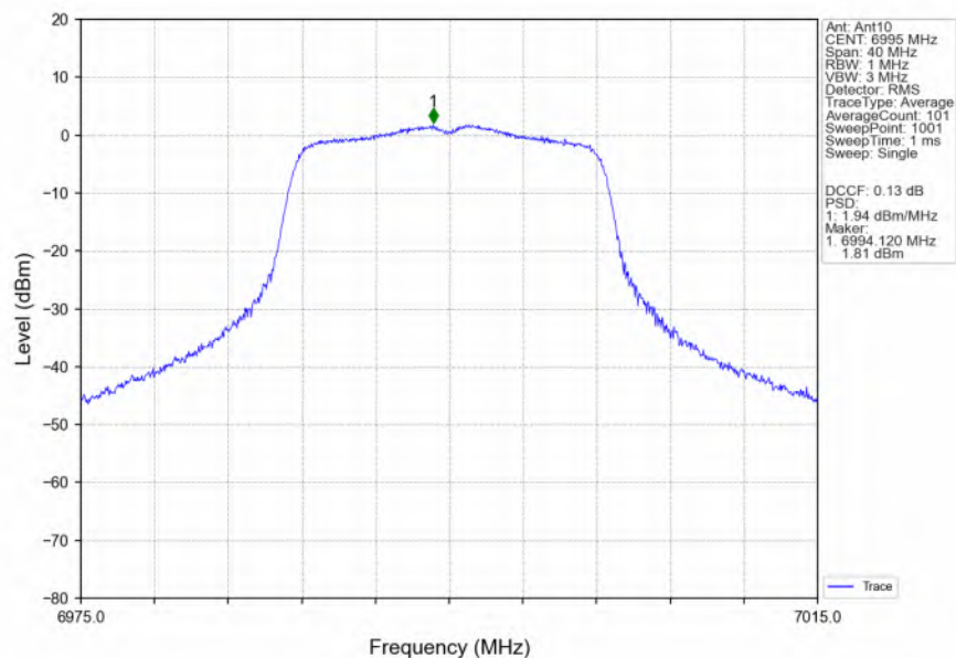
802.11a_MCH_6995MHz_Ant10_NTNV
