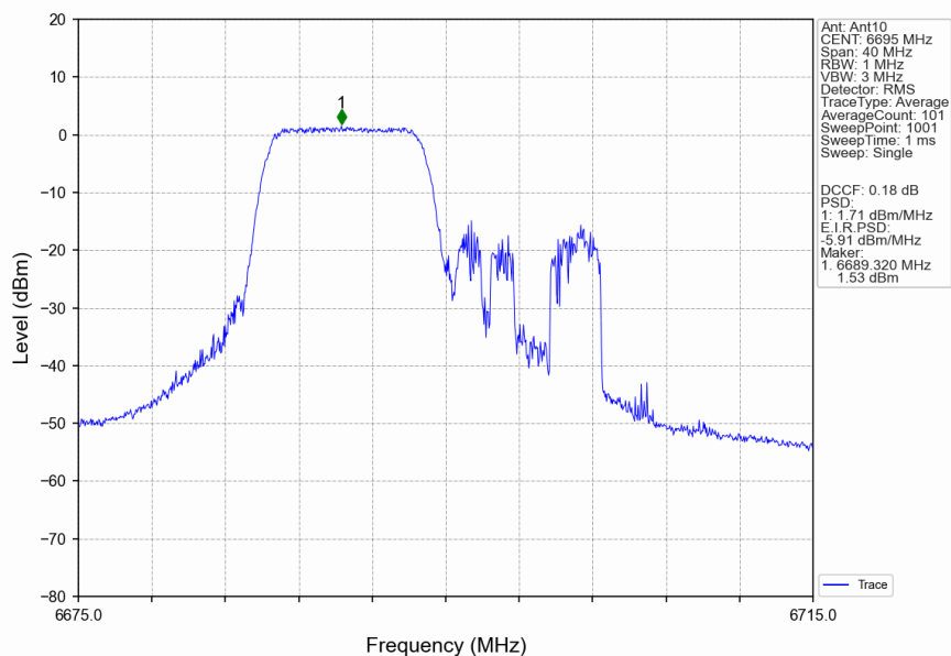
802.11ax(HEW20) MCH_6695MHz RU106 Left_Ant10 NTN
