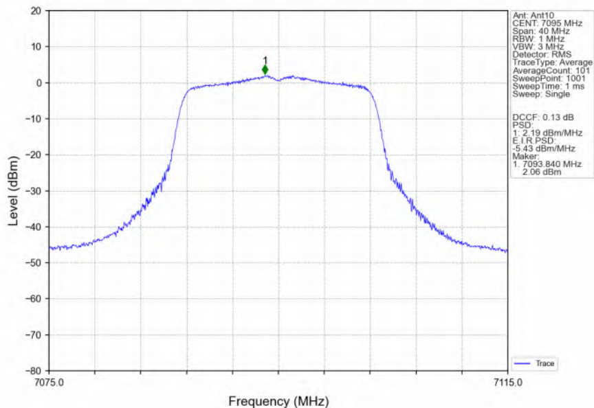
802.11a_HCH_7095MHz_Ant10_NTNV
