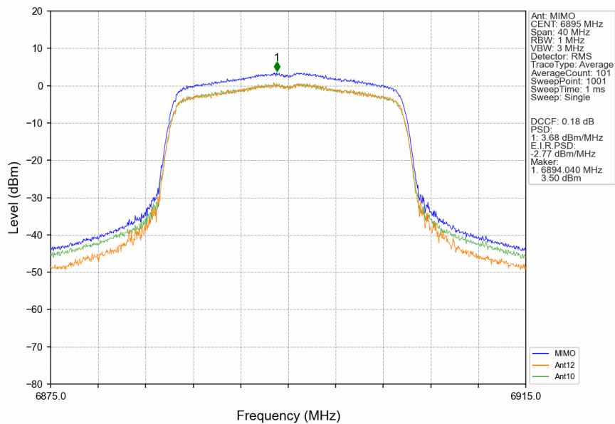
802.11ax(HEW20) LCH 6895MHz RU242 Left MIMO NTN
