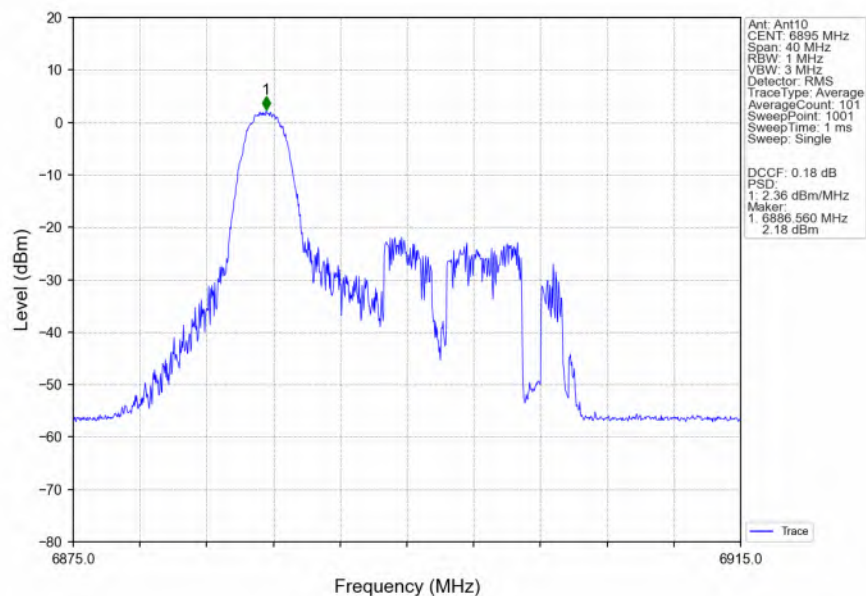
802.11ax(HEW20)_LCH_6895MHz_RU26_Left_Ant10_NTNV
