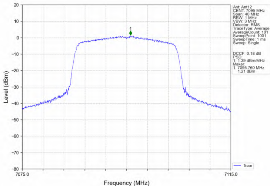
802.11ax(HEW20) HCH 7095MHz RU242 Left Ant12 NTN
