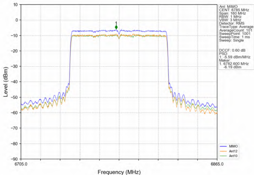
802.11ax(HEW80) HCH 6785MHz RU996 Left MIMO NTNW
