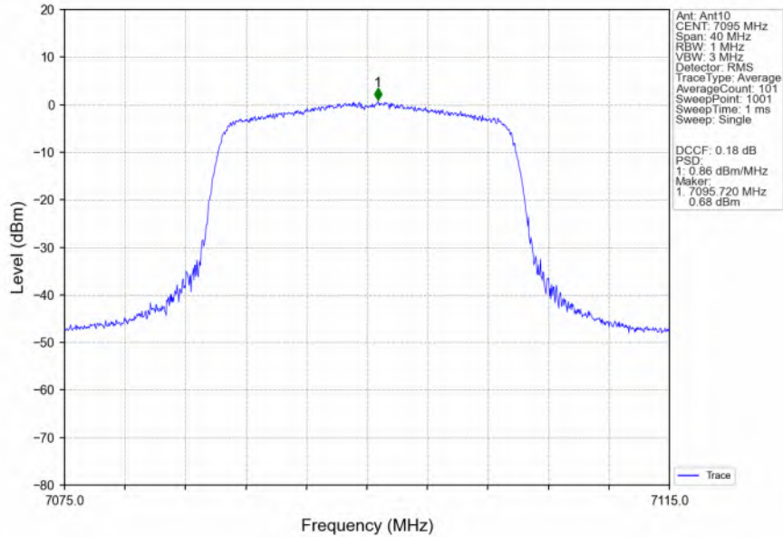
802.11ax(HEW20) HCH 7095MHz RU242 Left MIMO NTNW
