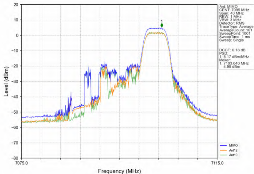
802.11ax(HEW20) HCH 7095MHz RU52 Right MIMO NTN
