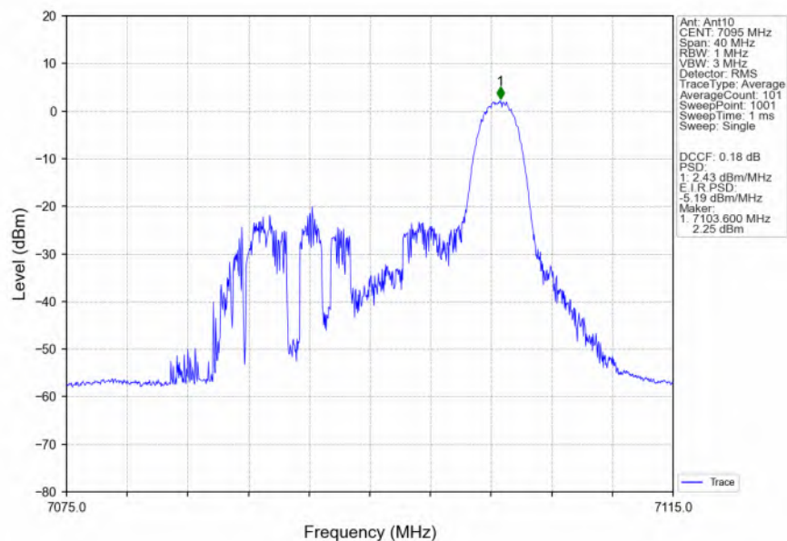
802.11ax(HEW20) HCH 7095MHz RU26 Right Ant10 NTN
