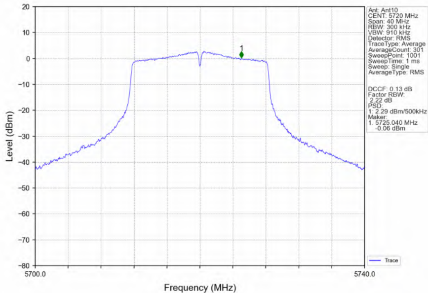
802.11a_HCH_5720MHz_Ant10_NTNV
