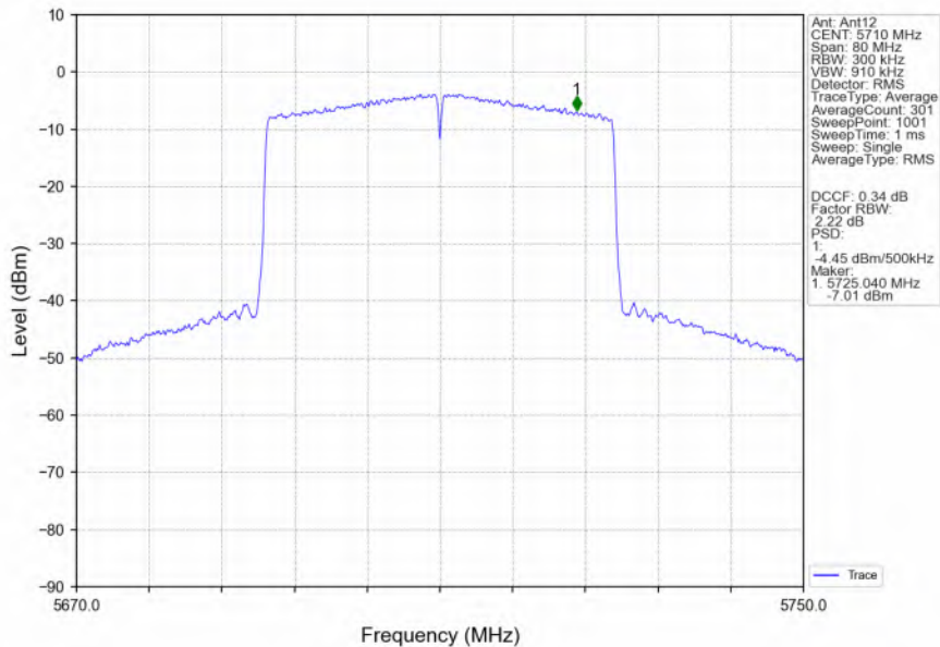
802.11ax(HEW40)_HCH_5710MHz_RU484_Left_Ant12_NTNV
