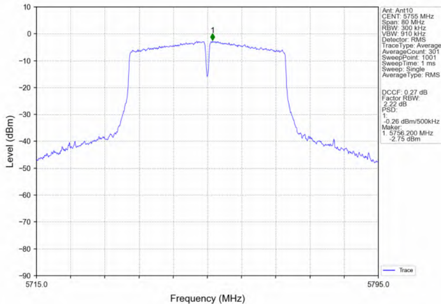
802.11n(HT40)_LCH_5755MHz_Ant10_NTNV
