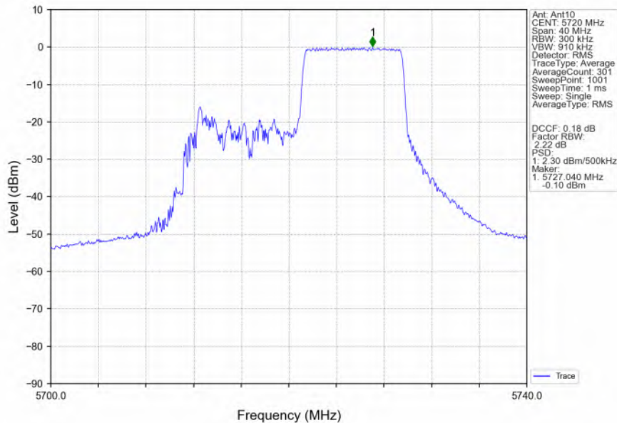
802.11ax(HEW20)_HCH_5720MHz_RU106_Right_Ant10_NTNV
