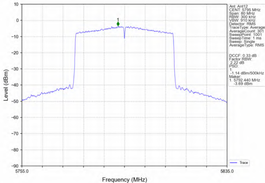
802.11ax(HEW40)_HCH_5795MHz_RU484_Left_Ant12_NTNV
