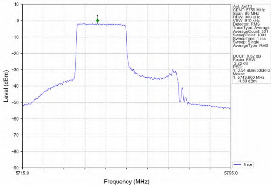
802.11ax(HEW40)_LCH_5755MHz_RU242_Left_Ant10_NTNV
