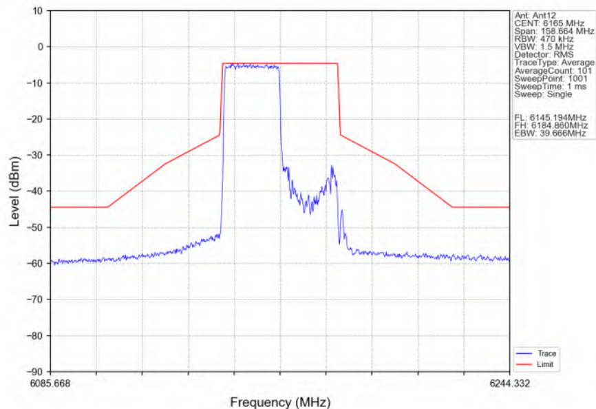
802.11ax(HEW40) MCH 6165MHz RU242 Left Ant12 NTN
