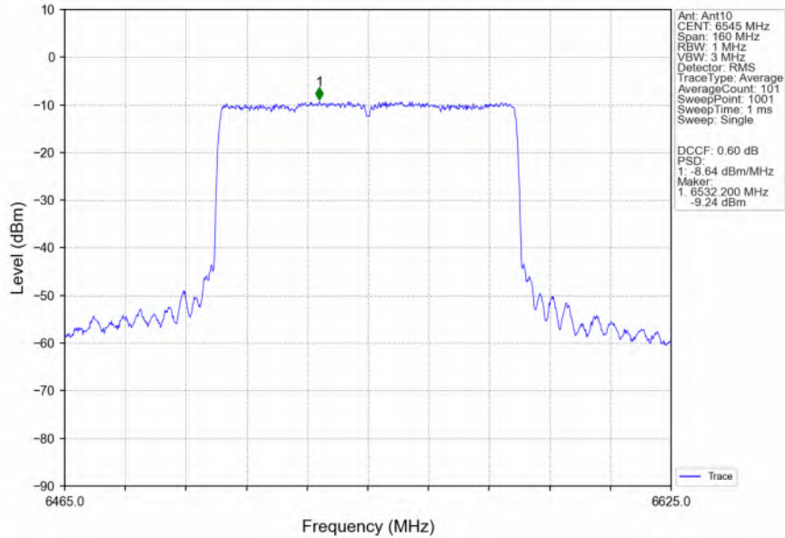
802.11ax(HEW80) HCH 6545MHz RU996 Left MIMO NTNW
