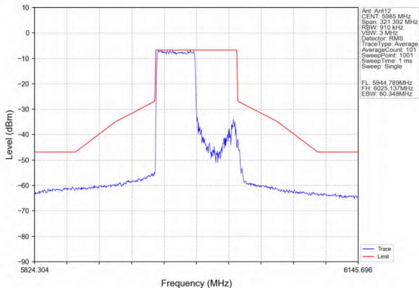
802.11ax(HEW80) LCH 5985MHz RU484 Left Ant12 NTNV
