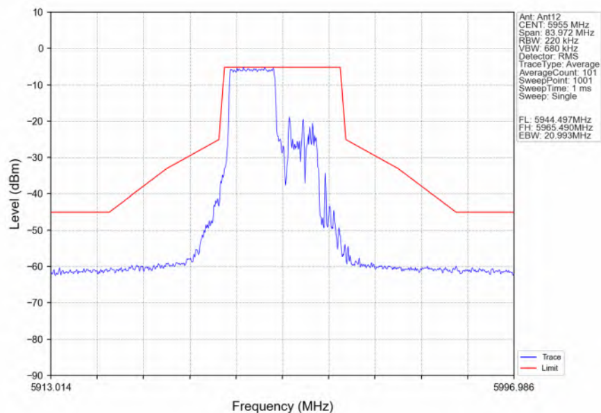
802.11ax(HEW20)_LCH_5955MHz_RU106_Left_Ant12_NTNV
