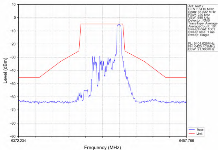
802.11ax(HEW20) HCH 6415MHz RU26 Right Ant12 NTNV
