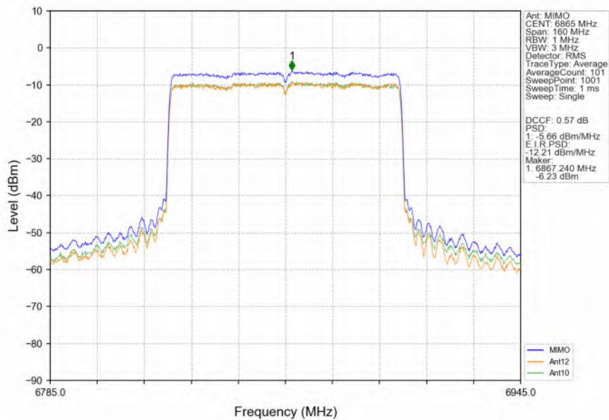
802.11ax(HEW80) HCH 6865MHz RU996 Left MIMO NTN
