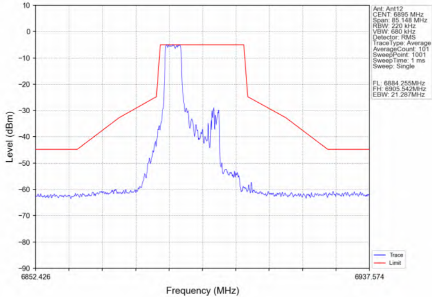
802.11ax(HEW20)_LCH_6895MHz_RU106_Left_Ant12_NTNV
