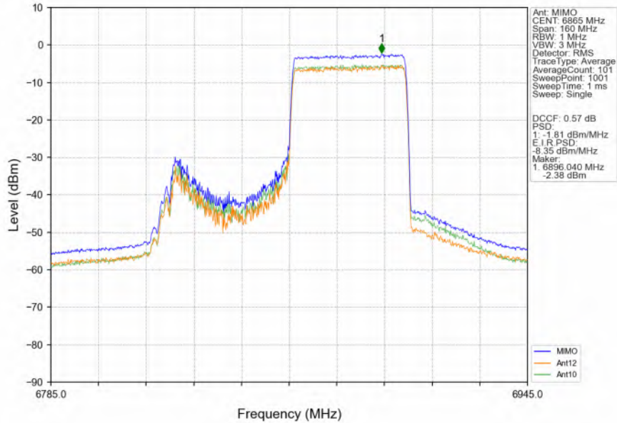
802.11ax(HEW80) HCH 6865MHz RU996 Left Ant12 NTN
