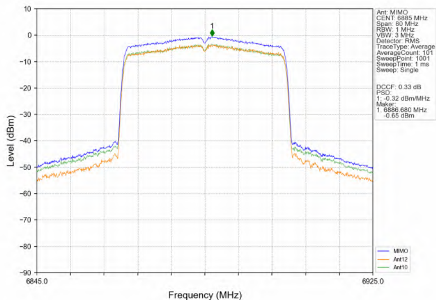
802.11ax(HEW40) HCH 6885MHz RU484 Left MIMO NTNW
