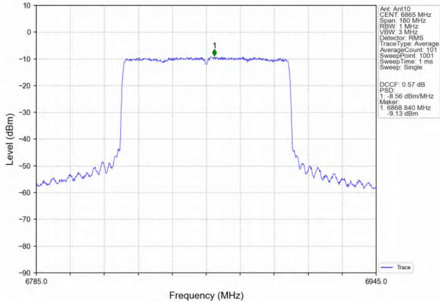
802.11ax(HEW80) HCH 6865MHz RU996 Left MIMO NTNW
