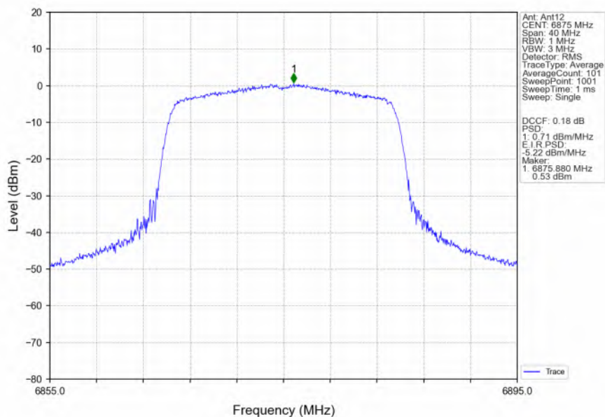
802.11ax(HEW20) HCH 6875MHz RU242 Left Ant12 NTN
