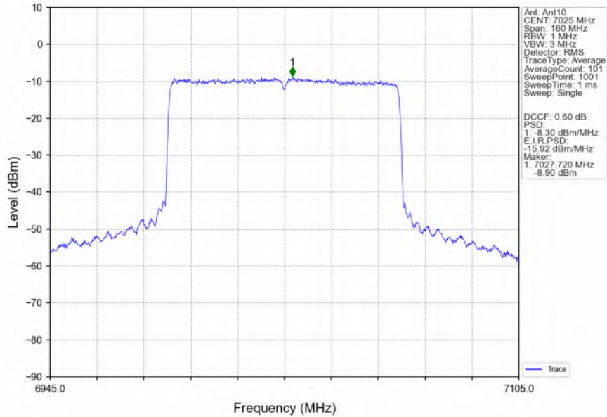
802.11ax(HEW80) HCH 7025MHz RU996 Left MIMO NTNW
