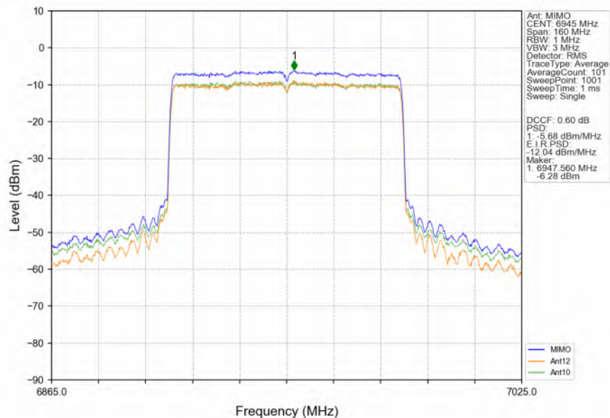
802.11ax(HEW80) LCH 6945MHz RU996 Left MIMO NTNv
