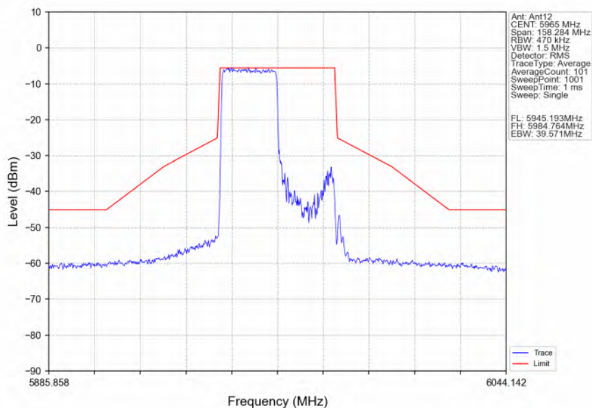
802.11ax(HEW40) LCH 5965MHz RU242 Left Ant12 NTNv
