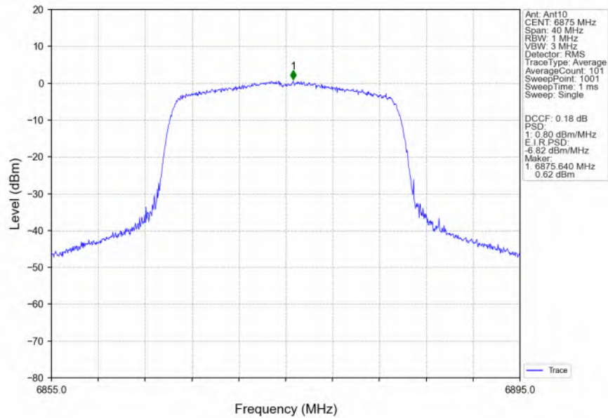
802.11ax(HEW20) HCH 6875MHz RU242 Left MIMO NTN
