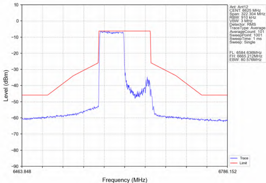
802.11ax(HEW80) LCH 6625MHz RU484 Left Ant12 NTNV
