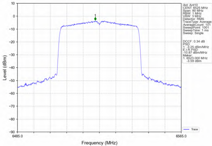
802.11ax(HEW40) HCH 6525MHz RU484 Left MIMO NTN
