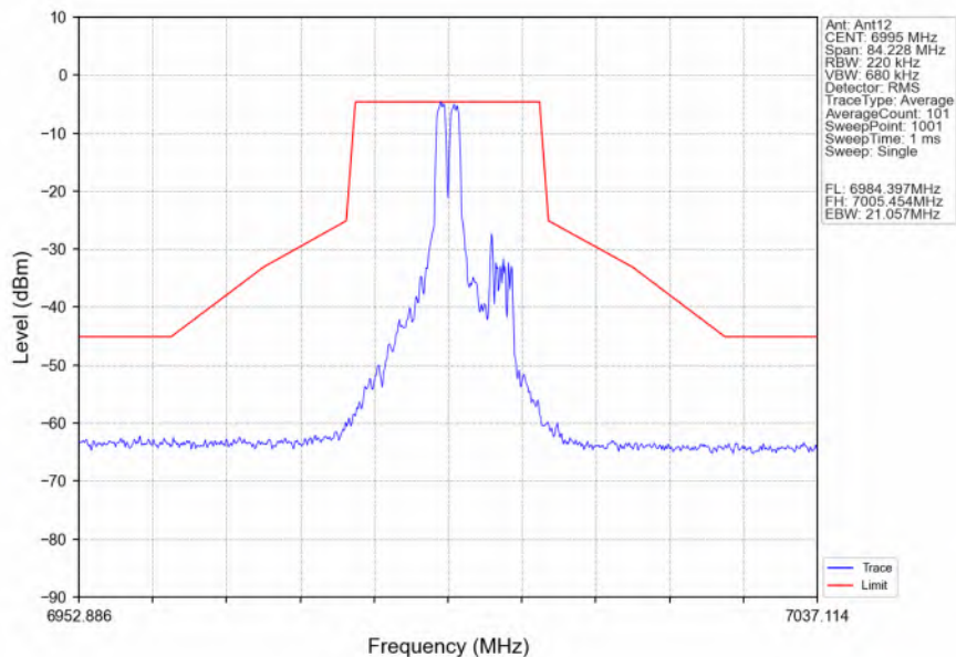
802.11ax(HEW20) MCH 6995MHz RU26 Mid Ant12 NTN
