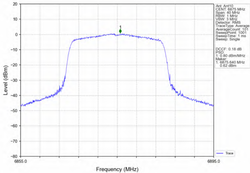
802.11ax(HEW20) HCH 6875MHz RU242 Left MIMO NTNW
