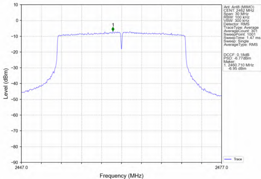
802.11ax(HEW20)_HCH_2462MHz_RU242_Left_Ant8 (MIMO)_NTNV
