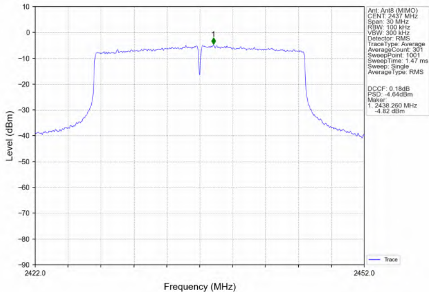
802.11ax(HEW20)_MCH_2437MHz_RU242_Left_Ant8 (MIMO)_NTNV
