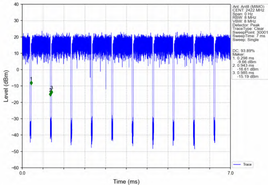
802.11n(HT40)_LCH_2422MHz_Ant8 (MIMO)_NTNV
