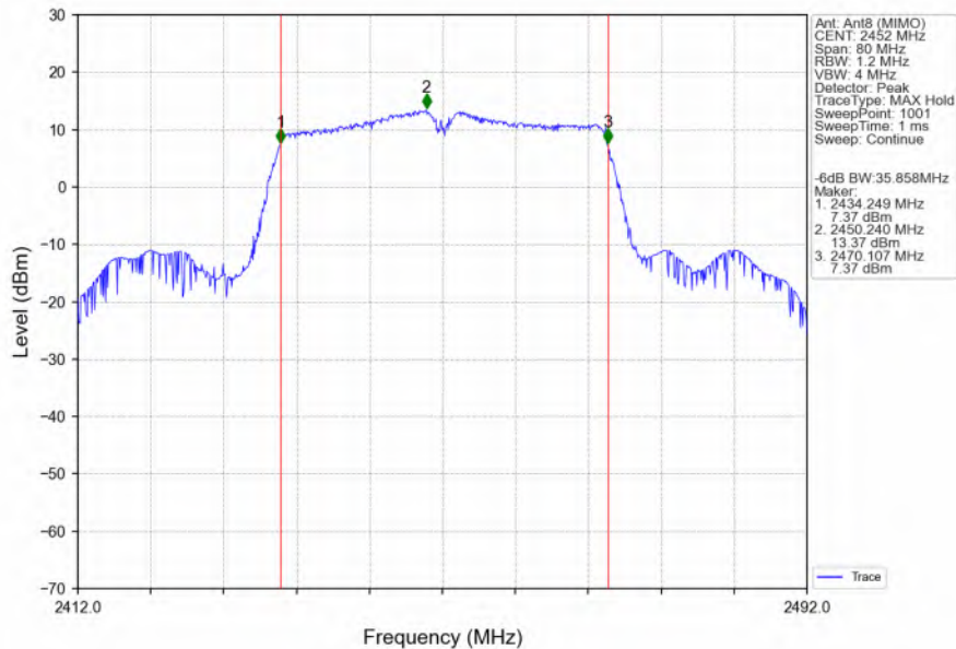
802.11n(HT40)_HCH_2452MHz_Ant8 (MIMO)_NTNV
