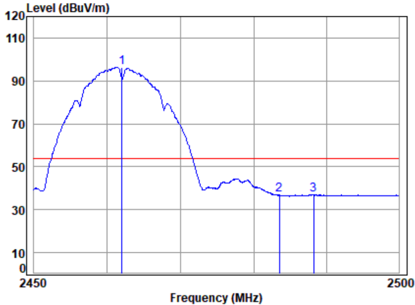
11b_TX_CH_11_Horizontal
