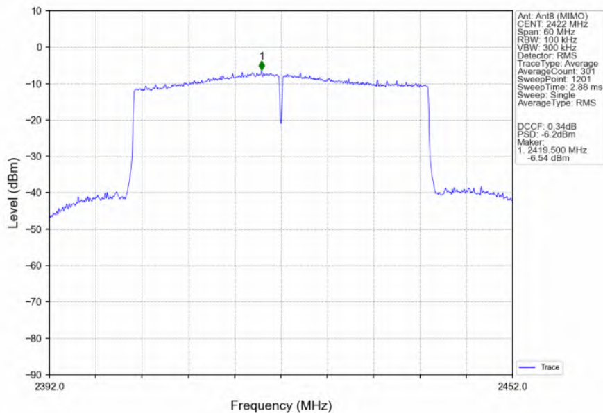
802.11ax(HEW40)_LCH_2422MHz_RU484_Left_Ant8 (MIMO)_NTNV
