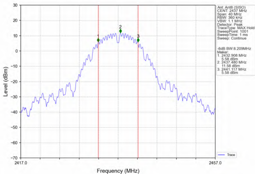
802.11b_MCH_2437MHz_Ant8 (SISO)_NTNV
