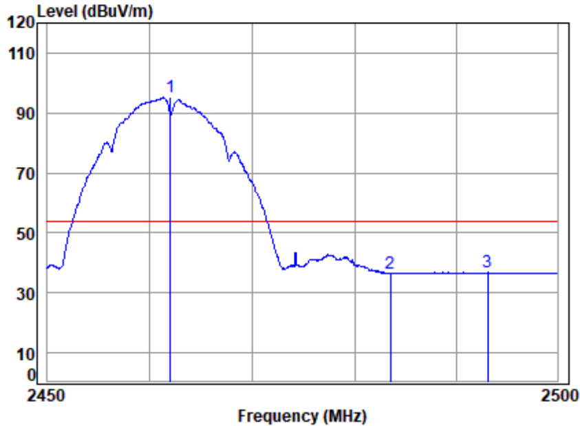
11b_TX_CH_11_Vertical
