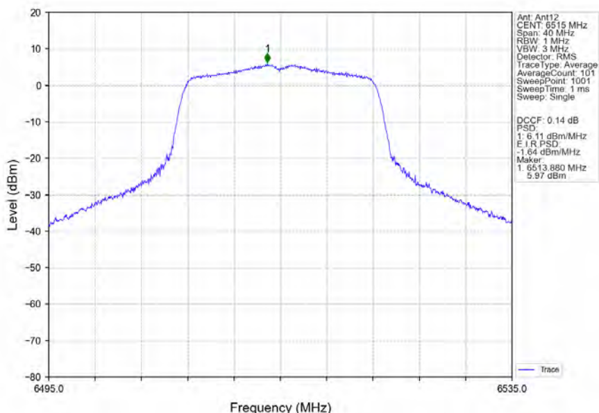
802.11a_HCH_6515MHz_Ant12_NTNV
