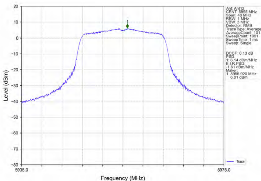
802.11a_LCH_5955MHz_Ant12_NTNV
