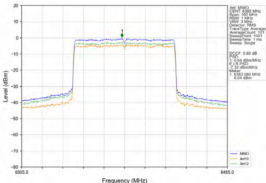
802.11ax(HEW80)_HCH_6385MHz_SU_/_MIMO_NTNV
