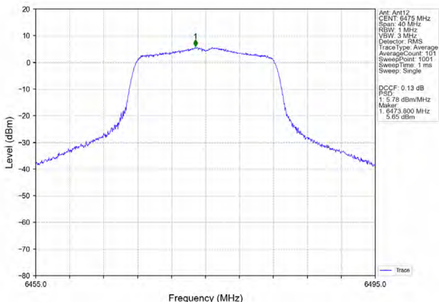
802.11a_MCH_6475MHz_Ant12_NTNV
