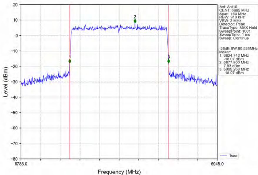
802.11ax(HEW80)_HCH_6865MHz_SU_/_Ant10_NTNV
