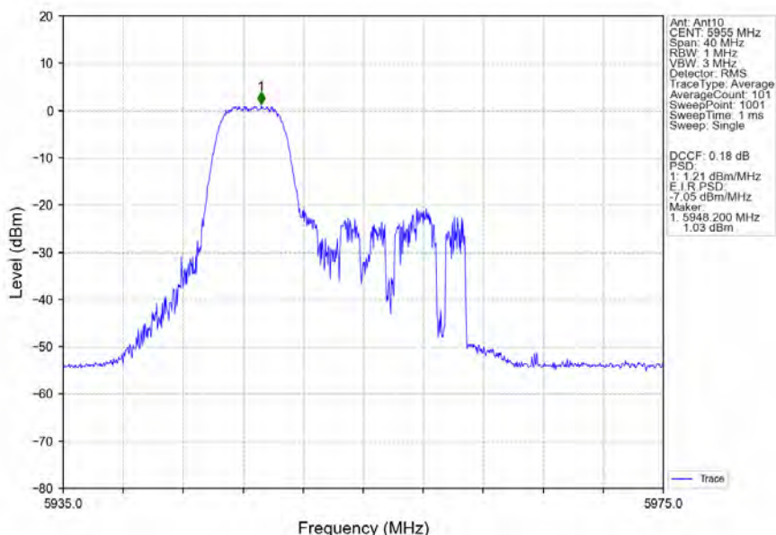
802.11ax(HEW20)_LCH_5955MHz_RU52_Left_Ant10_NTNV
