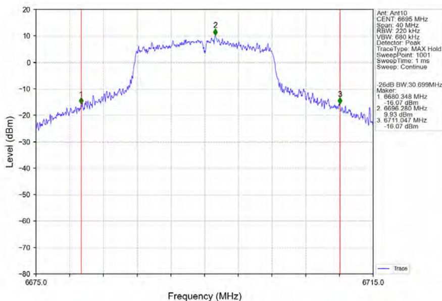
802.11a_MCH_6695MHz_Ant10_NTNV
