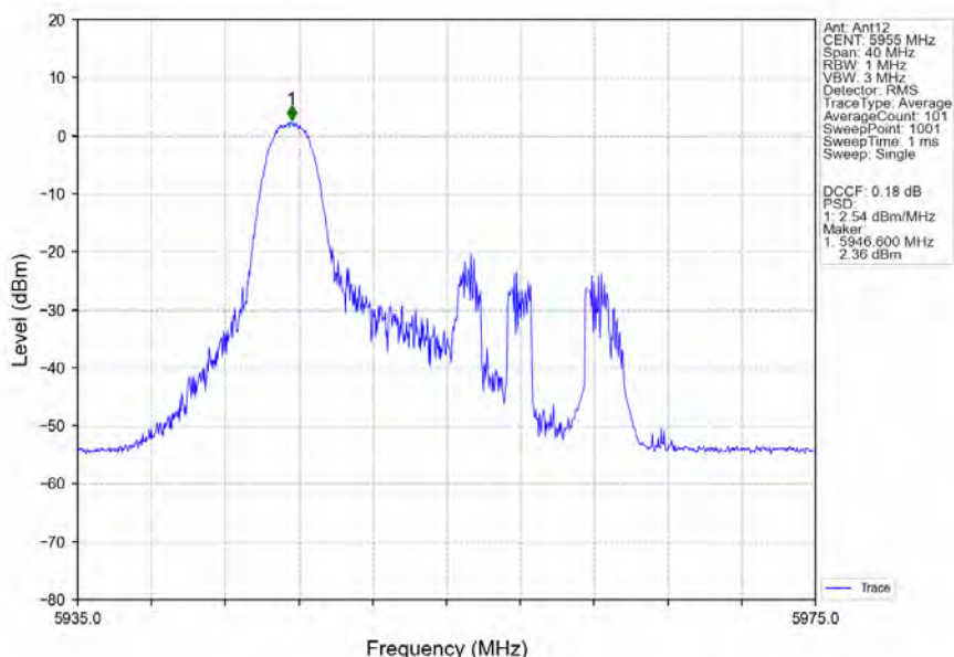
802.11ax(HEW20)_LCH_5955MHz_RU26_Left_Ant12_NTNV
