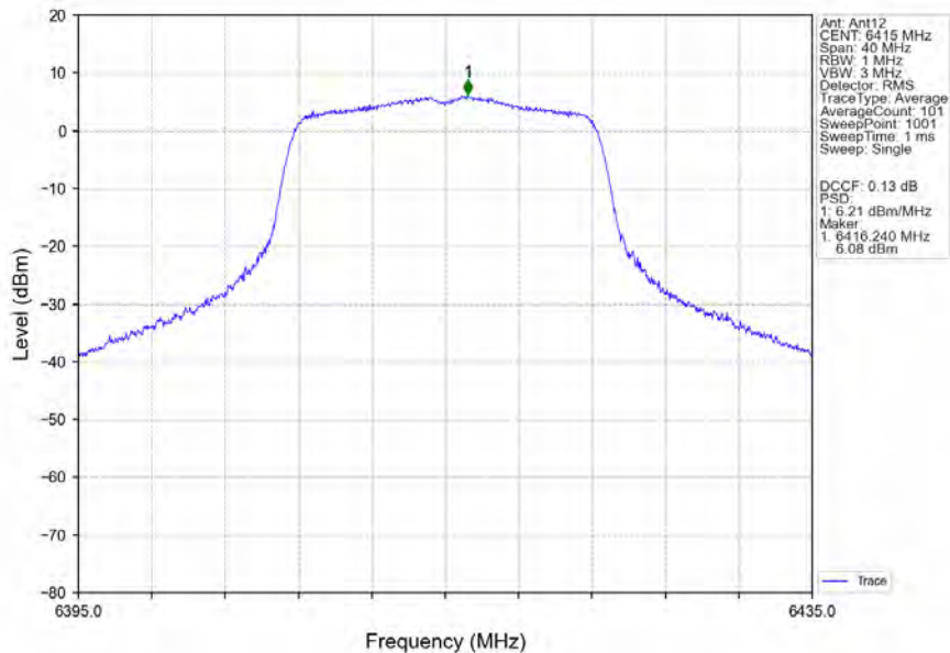
802.11a_HCH_6415MHz_Ant12_NTNV
