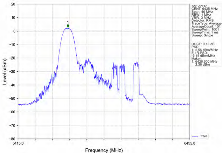
802.11ax(HEW20)_LCH_6435MHz_RU26_Left_Ant12_NTNV
