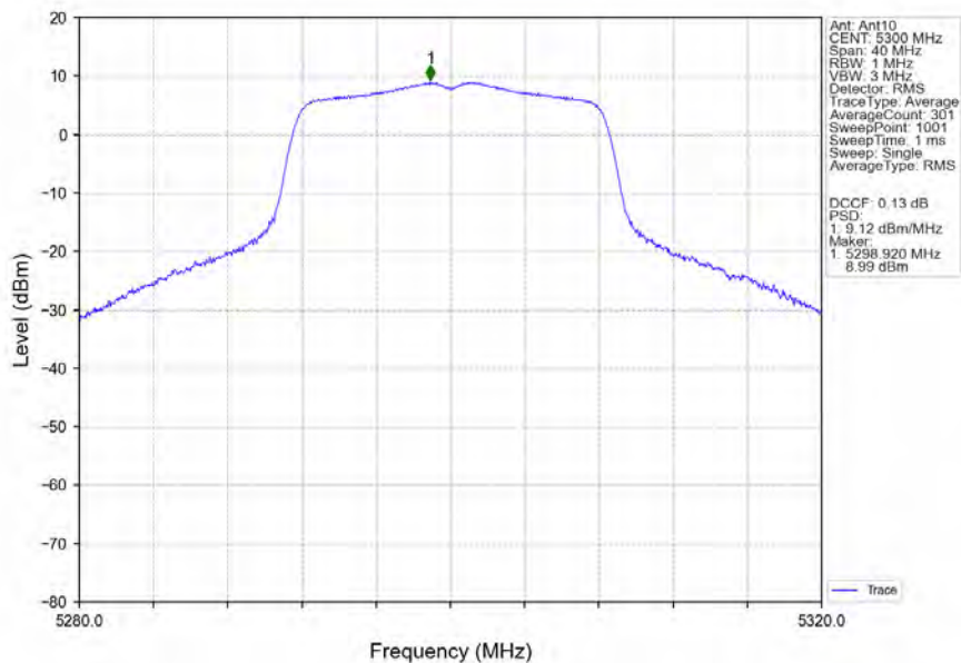
802.11a_MCH_5300MHz_Ant10_NTNV
