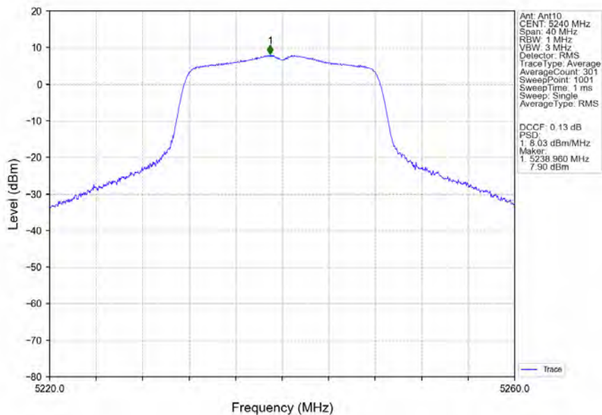
802.11a_HCH_5240MHz_Ant10_NTNV
