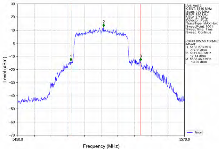
802.11ax(HEW40)_LCH_5510MHz_RU484_Left_Ant12_NTNV
