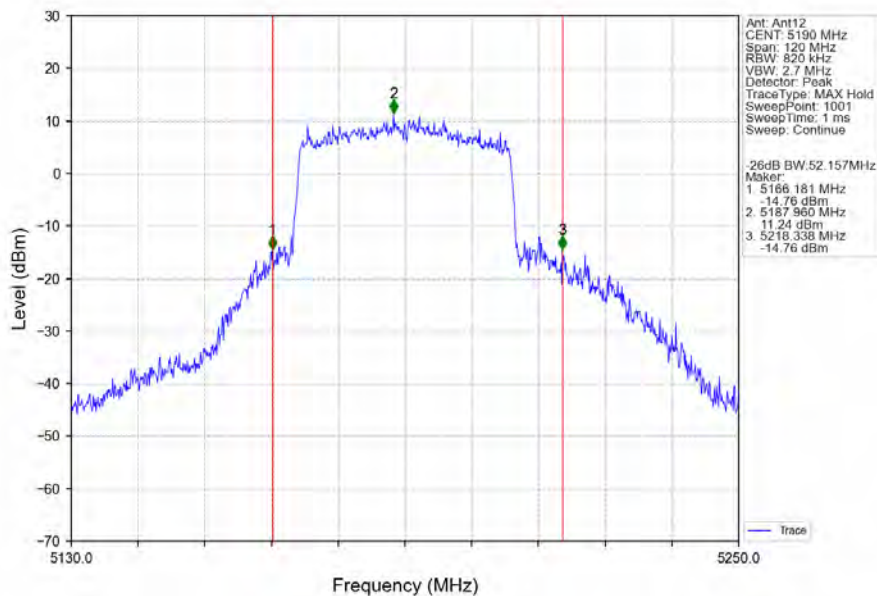
802.11ax(HEW40)_LCH_5190MHz_RU484_Left_Ant12_NTNV
