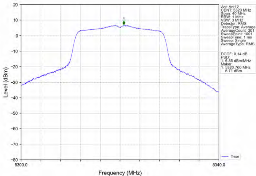
802.11n(HT20)_HCH_5320MHz_Ant12_NTNV
