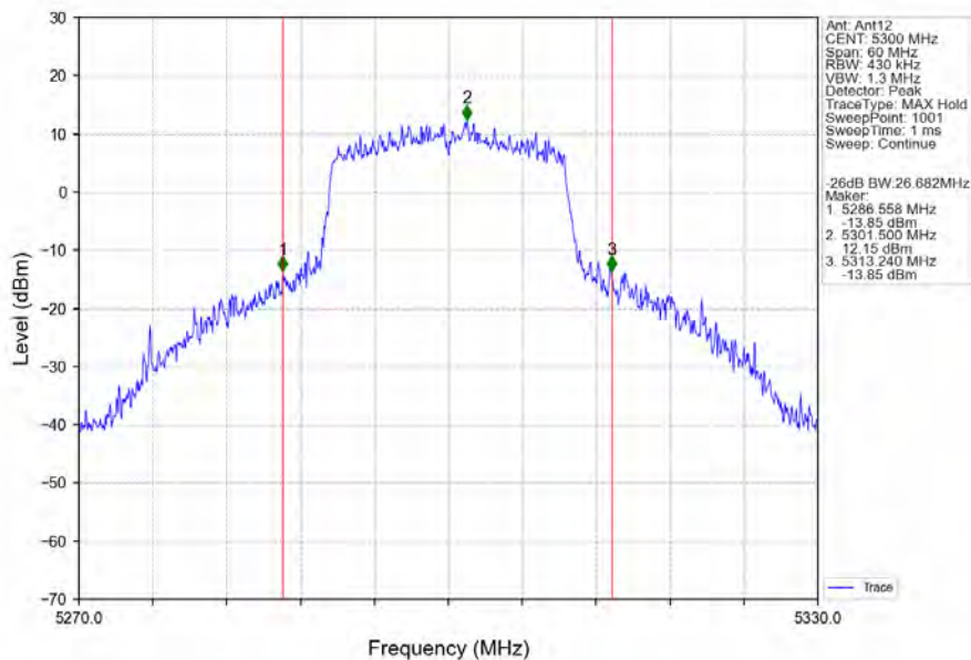
802.11ax(HEW20)_MCH_5300MHz_RU242_Left_Ant12_NTNV
