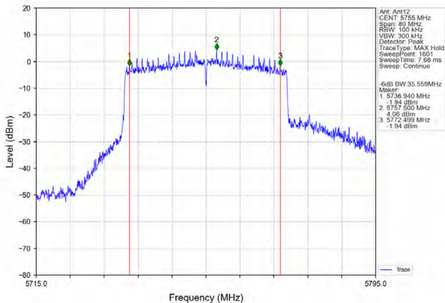
802.11ax(HEW40)_LCH_5755MHz_RU484_Left_Ant12_NTNV
