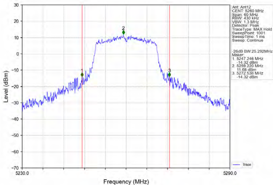
802.11n(HT20)_LCH_5260MHz_Ant12_NTNV
