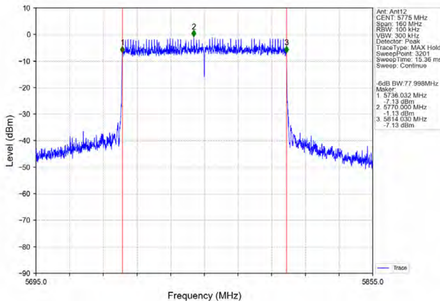
802.11ax(HEW80)_MCH_5775MHz_RU996_Left_Ant12_NTNV
