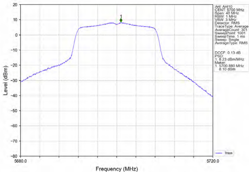
802.11a_HCH_5700MHz_Ant10_NTNV
