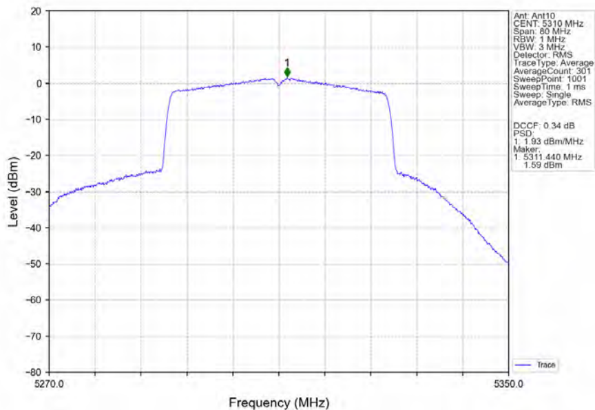
802.11ax(HEW40)_HCH_5310MHz_RU484_Left_Ant10_NTNV
