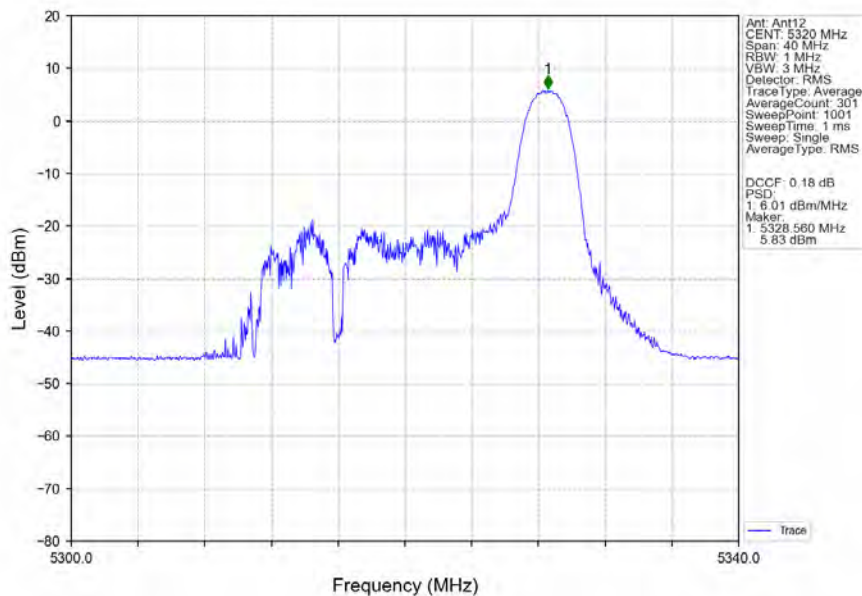
802.11ax(HEW20)_HCH_5320MHz_RU26_Right_Ant12_NTNV
