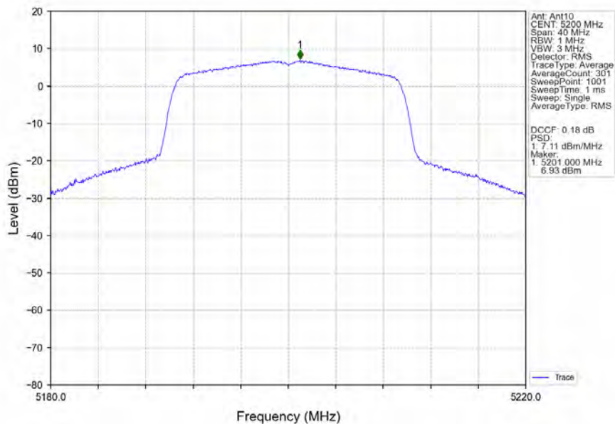
802.11ax(HEW20)_MCH_5200MHz_RU242_Left_Ant10_NTNV
