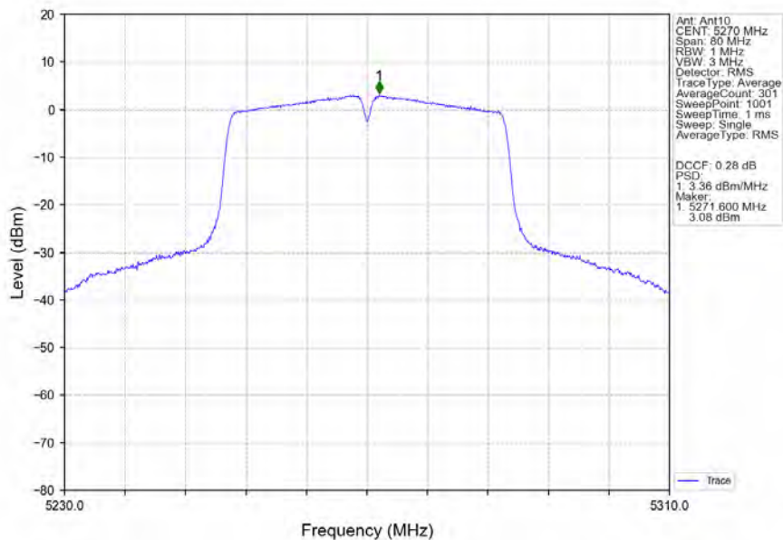
802.11ac(VHT40)_LCH_5270MHz_Ant10_NTNV
