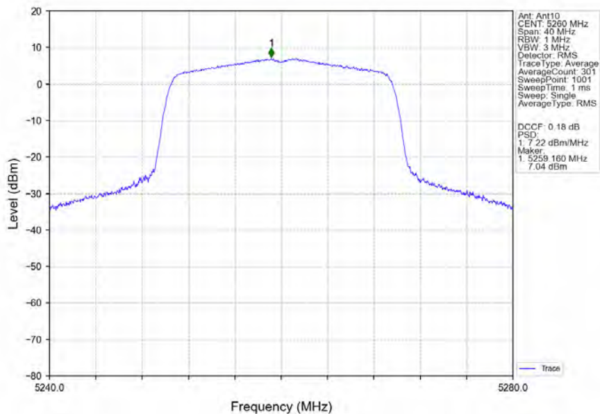
802.11ax(HEW20)_LCH_5260MHz_RU242_Left_Ant10_NTNV
