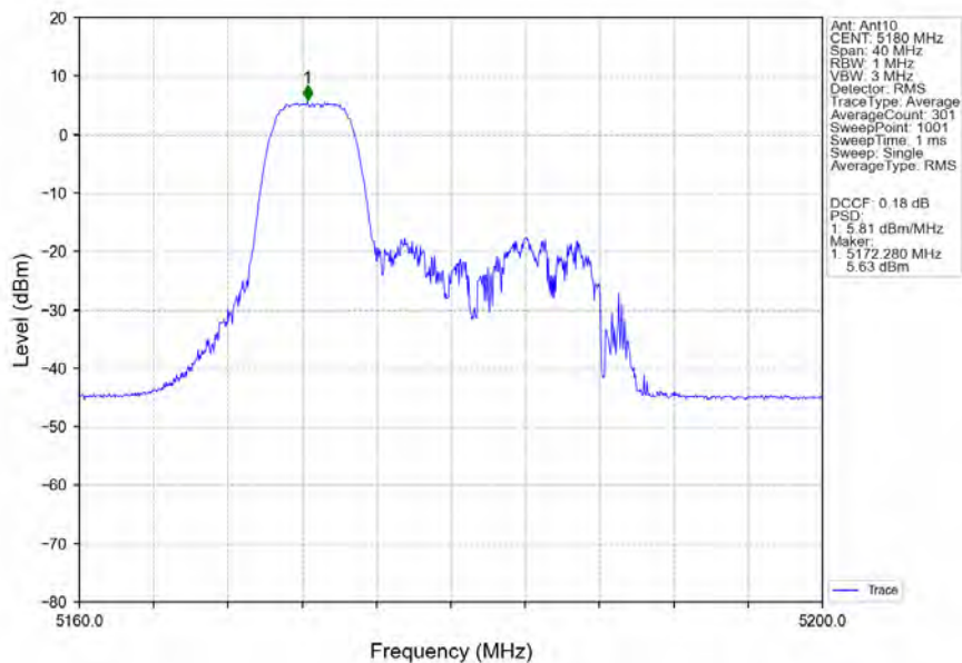
802.11ax(HEW20)_LCH_5180MHz_RU52_Left_Ant10_NTNV
