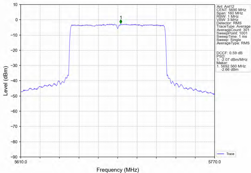
802.11ax(HEW80)_HCH_5690MHz_RU996_Left_Ant12_NTNV
