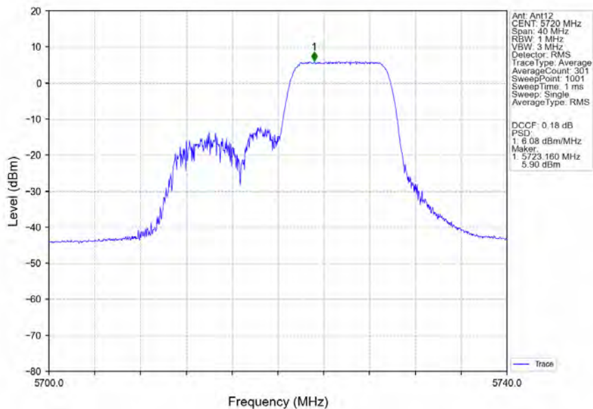
802.11ax(HEW20)_HCH_5720MHz_RU106_Right_Ant12_NTNV
