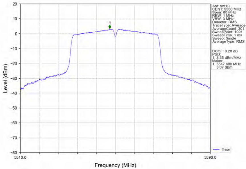
802.11n(HT40)_MCH_5550MHz_MIMO_NTNV
