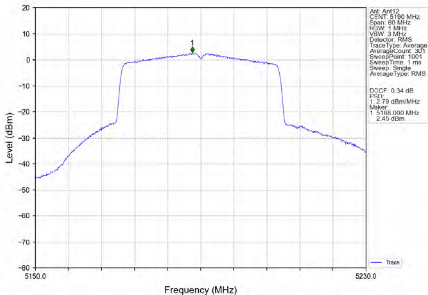
802.11ax(HEW40)_LCH_5190MHz_RU484_Left_Ant12_NTNV
