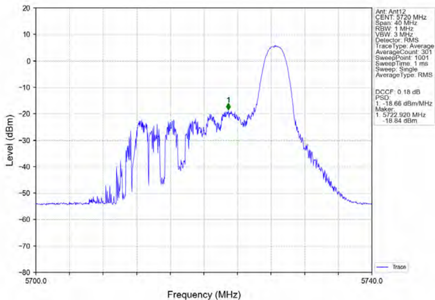
802.11ax(HEW20)_HCH_5720MHz_RU26_Right_Ant12_NTNV
