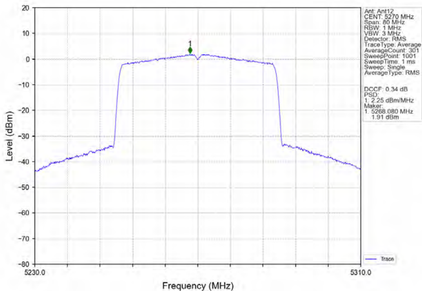
802.11ax(HEW40)_LCH_5270MHz_RU484_Left_Ant12_NTNV
