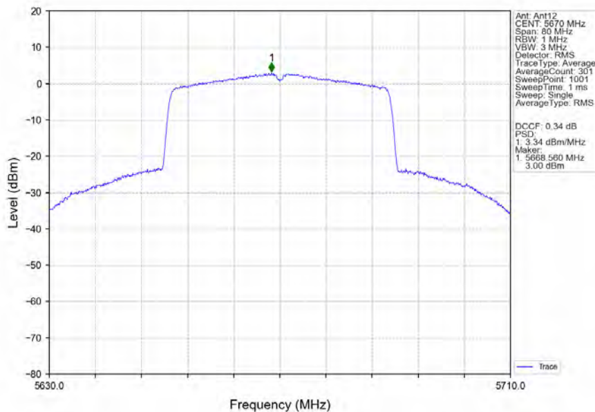
802.11ax(HEW40)_HCH_5670MHz_RU484_Left_Ant12_NTNV
