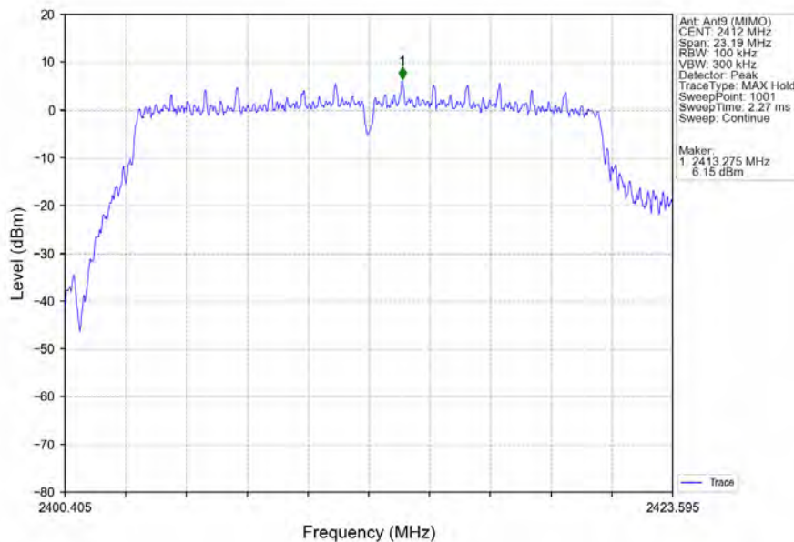
802.11n(HT20)_LCH_2412MHz_Ant9 (MIMO)_NTNV
