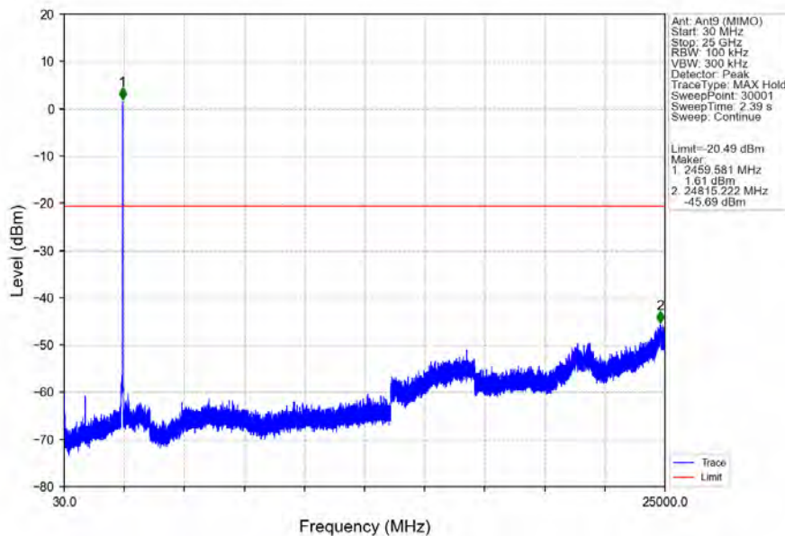
802.11n(HT20)_HCH_2462MHz_Ant9 (MIMO)_NTNV
