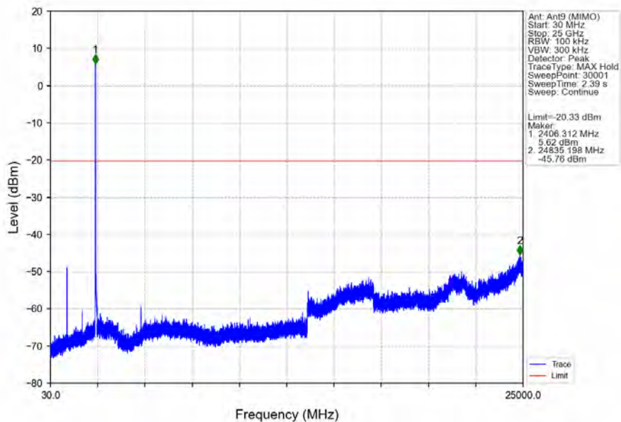
802.11ax(HEW20)_LCH_2412MHz_RU52_Left_Ant9 (MIMO)_NTNV
