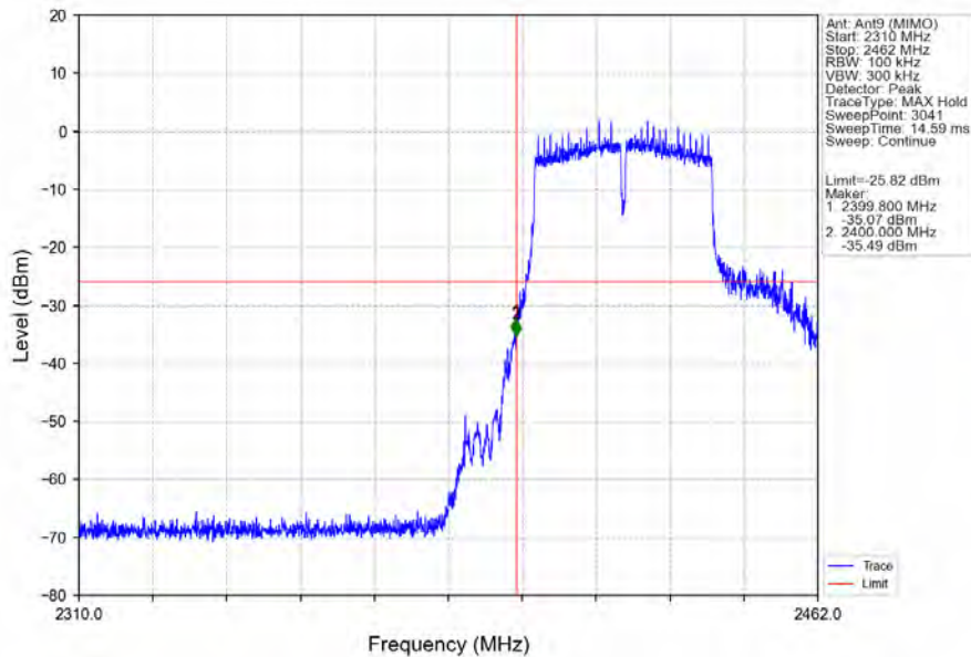
802.11n(HT40)_LCH_2422MHz_Ant9 (MIMO)_NTNV
