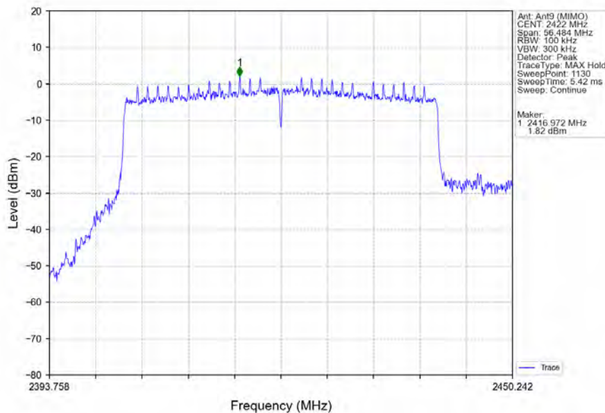
802.11ax(HEW40)_LCH_2422MHz_RU484_Left_Ant9 (MIMO)_NTNV
