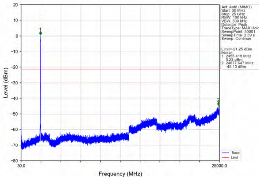
802.11n(HT20)_HCH_2462MHz_Ant8 (MIMO)_NTNV
