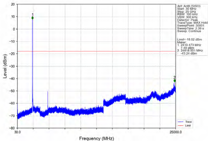
802.11b_LCH_2412MHz_Ant8 (SISO)_NTNV
