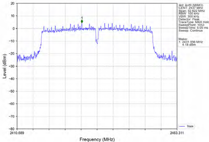
802.11n(HT40)_MCH_2437MHz_Ant9 (MIMO)_NTNV
