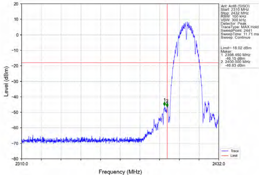
802.11b_LCH_2412MHz_Ant8 (SISO)_NTNV
