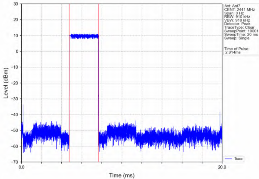
8DPSK_3DH5_HOPP_Ant7_NTNV
