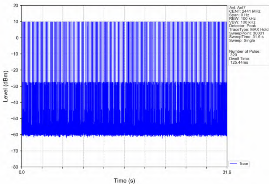
8DPSK_3DH1_HOPP_Ant7_NTNV
