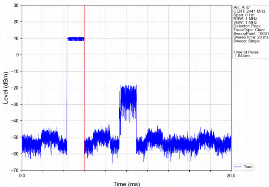
Pi/4DQPSK_2DH3_HOPP_Ant7_NTNV
