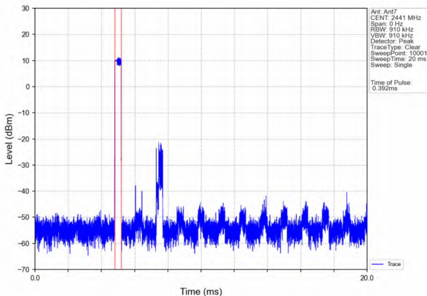
8DPSK_3DH1_HOPP_Ant7_NTNV
