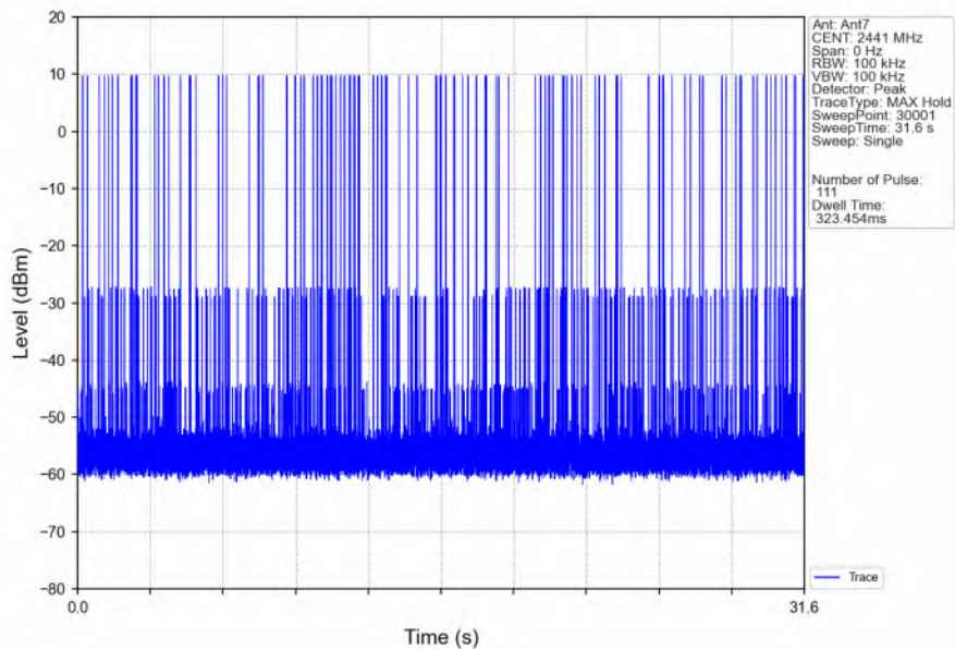
8DPSK_3DH5_HOPP_Ant7_NTNV
