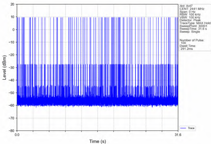
Pi/4DQPSK_2DH5_HOPP_Ant7_NTNV
