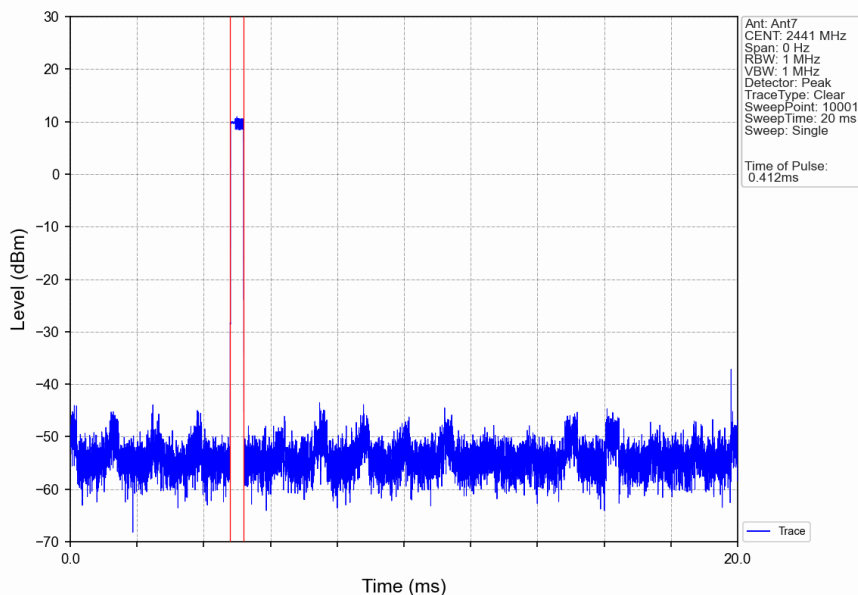
Pi/4DQPSK_2DH1_HOPP_Ant7_NTNV
