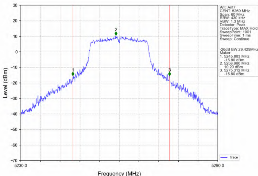
802.11n(HT20)_LCH_5260MHz_Ant7_NTNV
