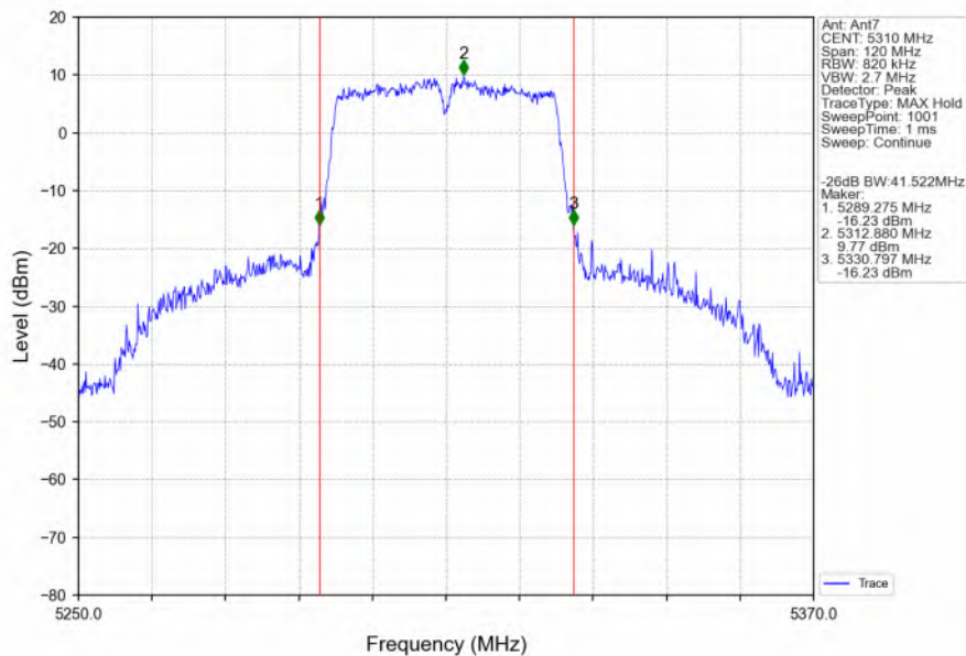
802.11n(HT40)_HCH_5310MHz_Ant7_NTNV
