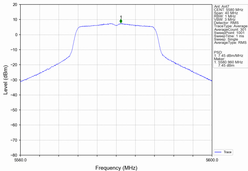
802.11a_MCH_5580MHz_Ant7_NTNV
