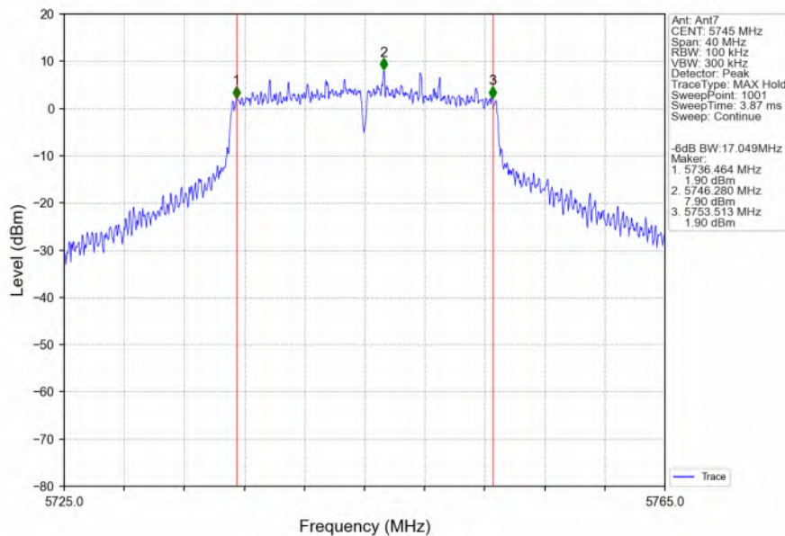
802.11n(HT20)_LCH_5745MHz_Ant7_NTNV
