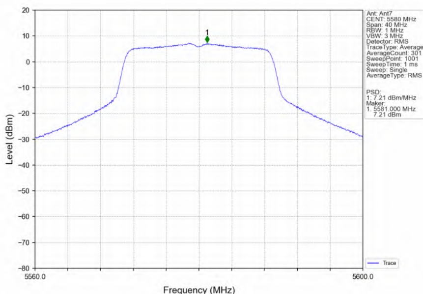
802.11n(HT20)_MCH_5580MHz_Ant7_NTNV
