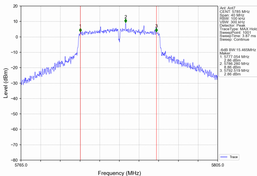
802.11a_MCH_5785MHz_Ant7_NTNV
