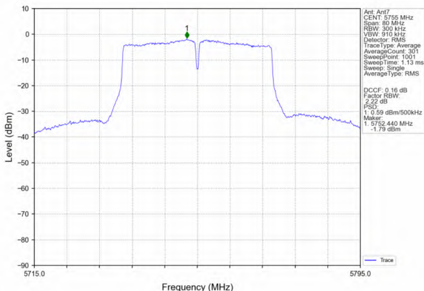
802.11ac(VHT40)_LCH_5755MHz_Ant7_NTNV
