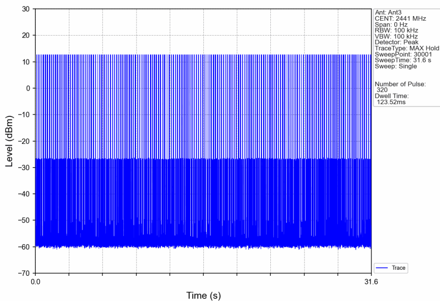
Pi/4DQPSK_2DH1_HOPP_Ant3_NTNV
