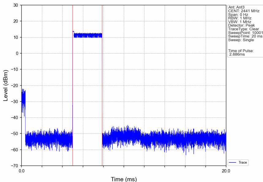
Pi/4DQPSK_2DH5_HOPP_Ant3_NTNV
