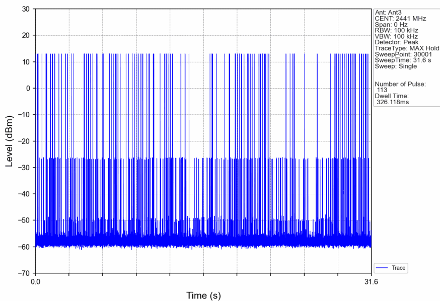
Pi/4DQPSK_2DH5_HOPP_Ant3_NTNV
