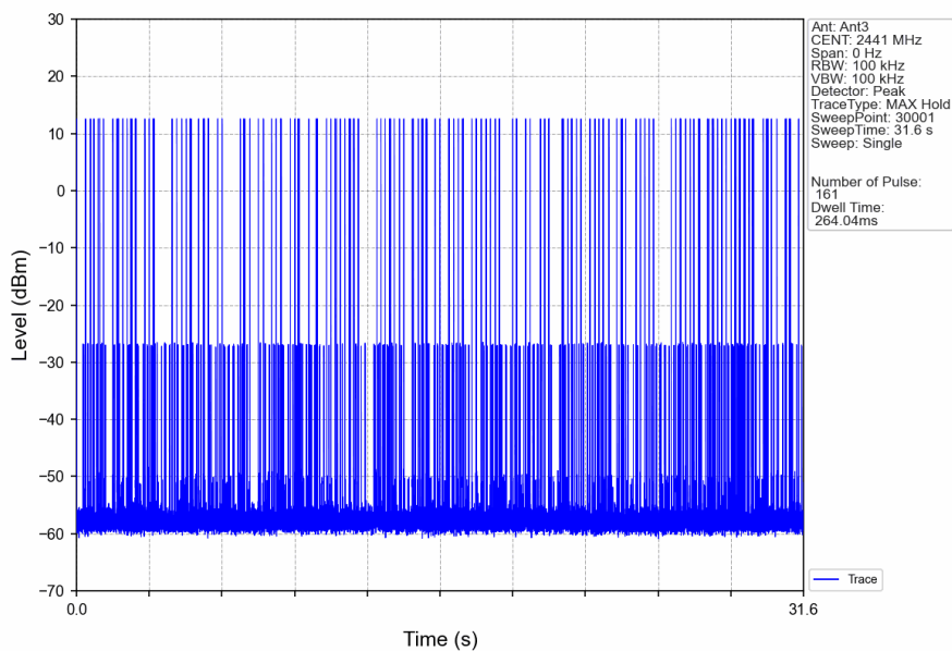
Pi/4DQPSK_2DH3_HOPP_Ant3_NTNV
