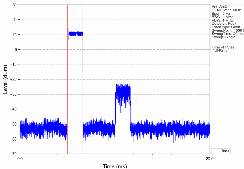
Pi/4DQPSK_2DH3_HOPP_Ant3_NTNV
