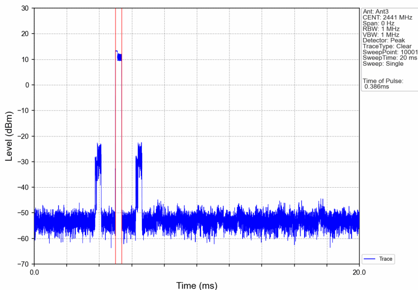
Pi/4DQPSK_2DH1_HOPP_Ant3_NTNV
