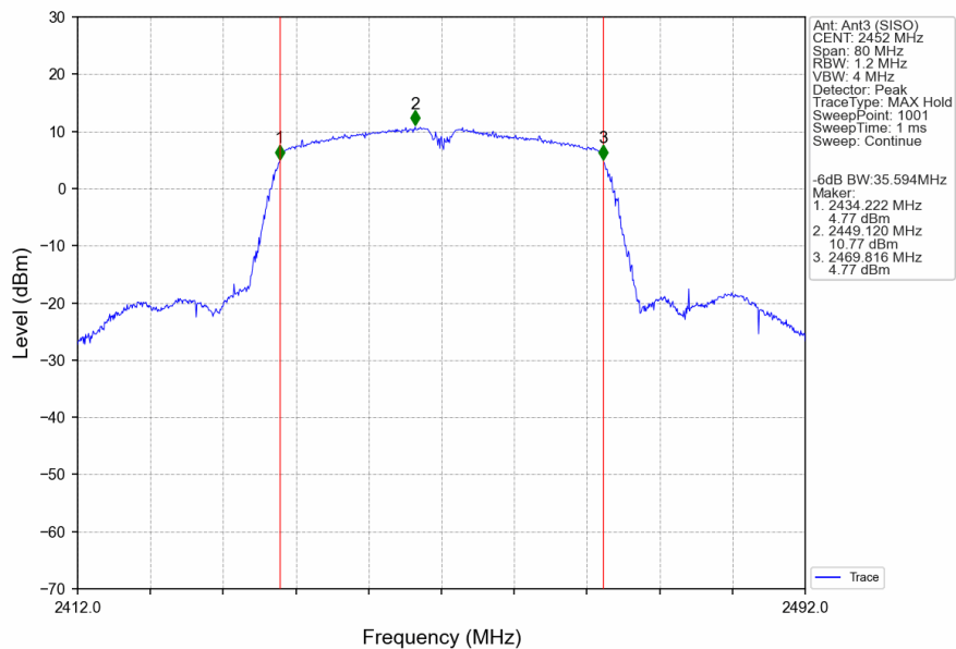
802.11n(HT40)_HCH_2452MHz_Ant3 (SISO)_NTNV
