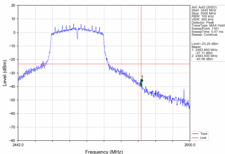
802.11n(HT20)_HCH_2462MHz_Ant3 (SISO)_NTNV
