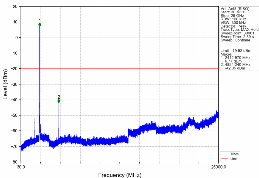
802.11b_LCH_2412MHz_Ant3 (SISO)_NTNV
