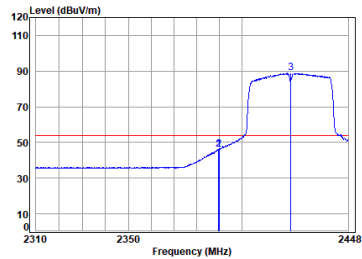
11n_HT(40M)_TX_CH_03_Horizontal-Avg
