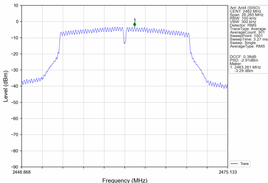
802.11g_HCH_2462MHz_Ant4 (SISO)_NTNV
