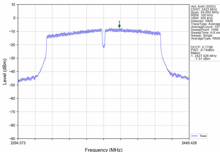
802.11n(HT40)_LCH_2422MHz_Ant4 (SISO)_NTNV
