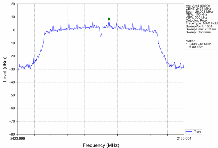
802.11n(HT20)_MCH_2437MHz_Ant4 (SISO)_NTNV
