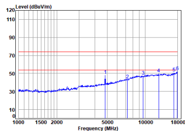
11n_20M_TX_CH_01_Vertical
