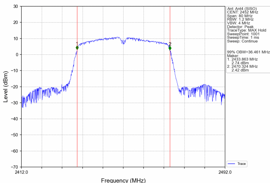
802.11n(HT40)_HCH_2452MHz_Ant4 (SISO)_NTNV
