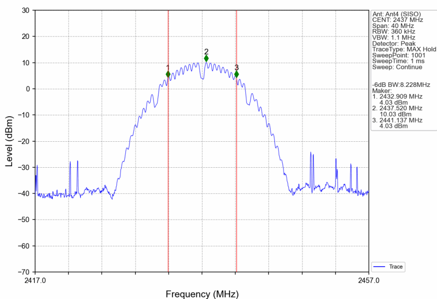
802.11b_MCH_2437MHz_Ant4 (SISO)_NTNV
