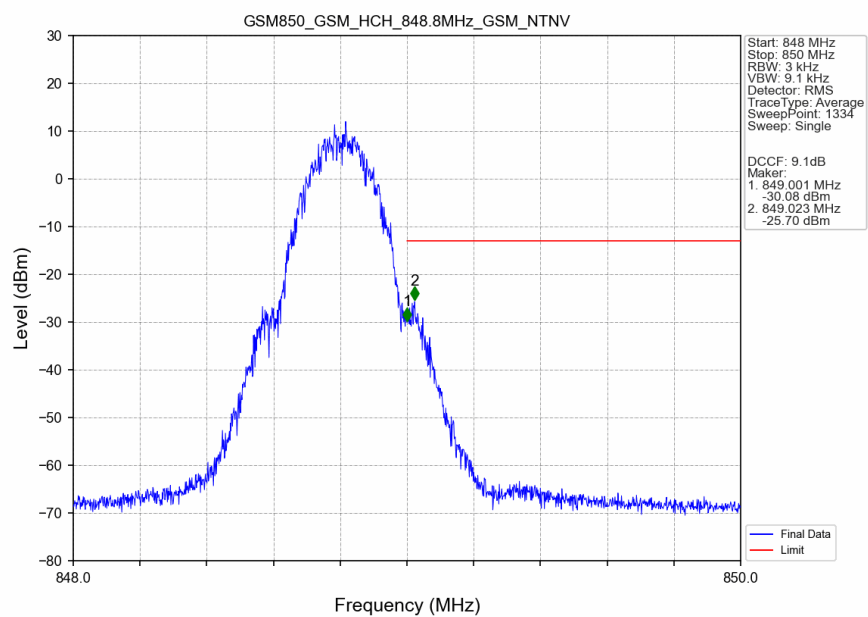
GSM850_GSM_HCH_848.8MHz_GSM_NTNV
