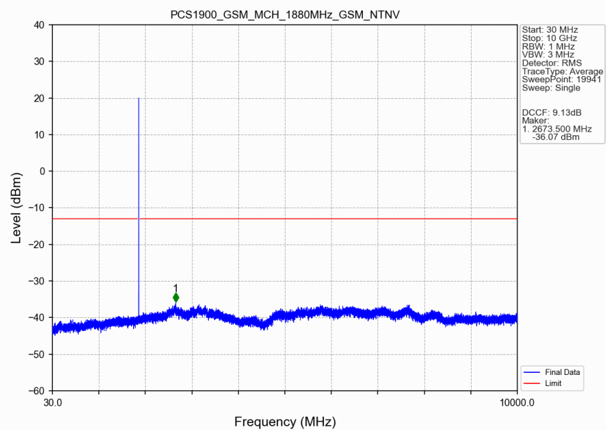
PCS1900_GSM_MCH_1880MHz_GSM_NTNV
