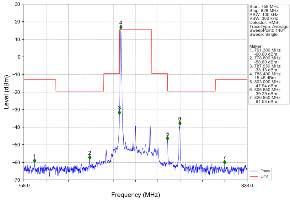
n14_15kHz_SISO_NTNV_10MHz_CP-OFDM_256_QAM_793MHz_Edge_1RB_Left_Ant0
