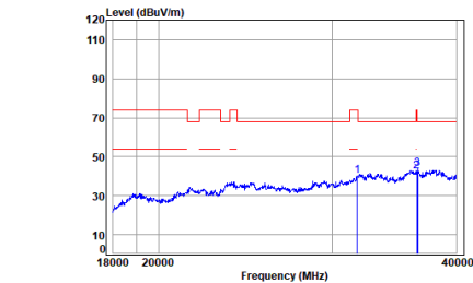
11a_Straddle_TX_CH_144_Horizontal
