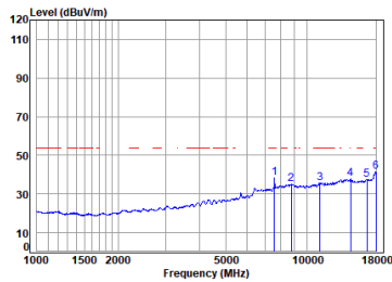
11ac_80M_Straddle_TX_CH_138_Vertical-Avg
