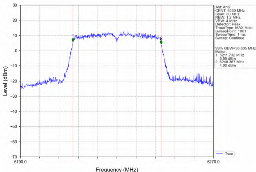
802.11n(HT40)_HCH_5230MHz_Ant7_NTNV
