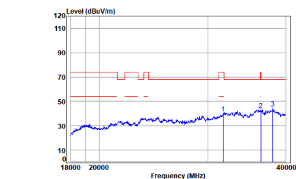
11a_TX_CH_52_Horizontal.gif
