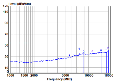
11ac_80M_Straddle_TX_CH_138_Horizontal-Avg
