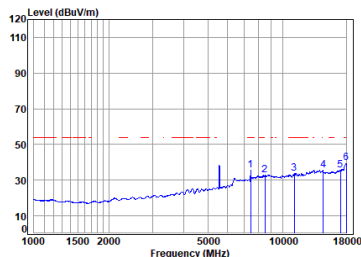
11a_TX_CH_116_Horizontal-Avg
