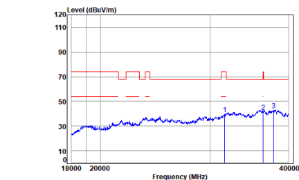
11a_TX_CH_157_Horizontal
