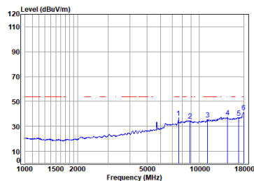
11ac_40M_Straddle_TX_CH_142_Vertical-Avg
