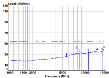
11a_Straddle_TX_CH_144_Horizontal-Avg
