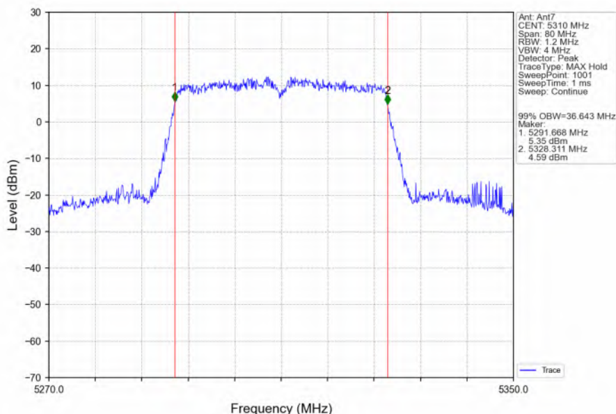
802.11n(HT40)_HCH_5310MHz_Ant7_NTNV
