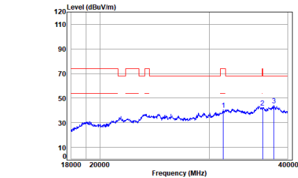
11a_TX_CH_36_Horizontal.gif
