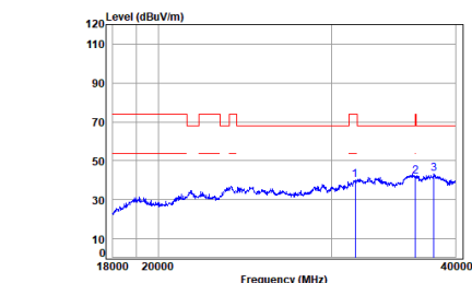
11a_TX_CH_48_Horizontal.gif
