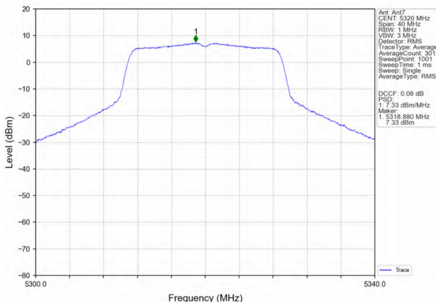
802.11n(HT20)_HCH_5320MHz_Ant7_NTNV
