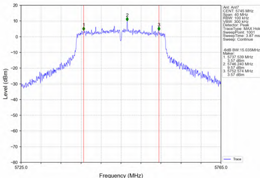
802.11n(HT20)_LCH_5745MHz_Ant7_NTNV
