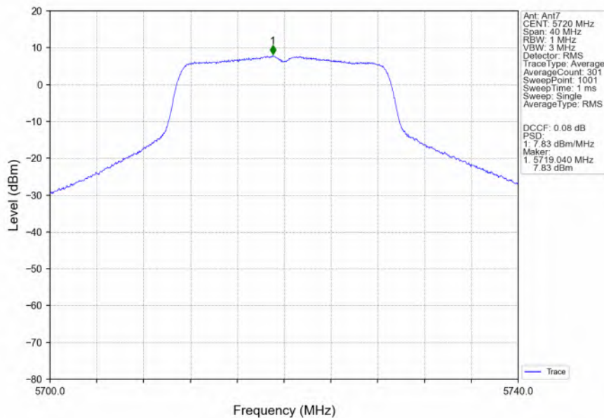
802.11a_HCH_5720MHz_Ant7_NTNV
