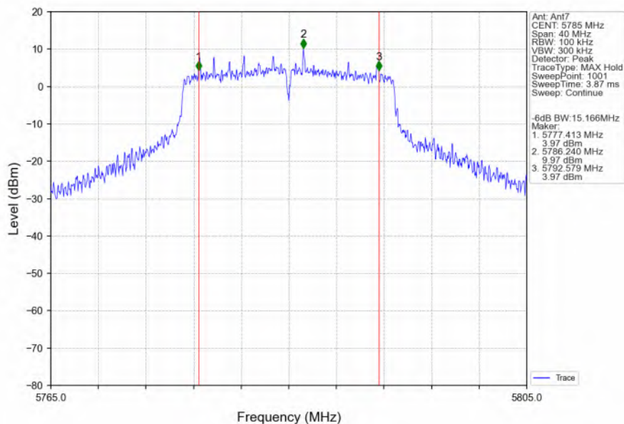
802.11a_MCH_5785MHz_Ant7_NTNV
