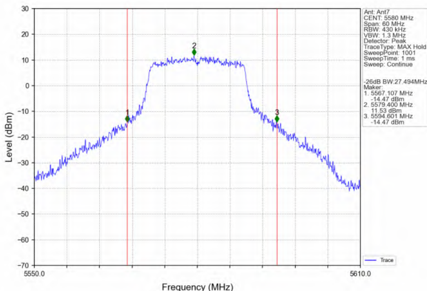
802.11a_MCH_5580MHz_Ant7_NTNV
