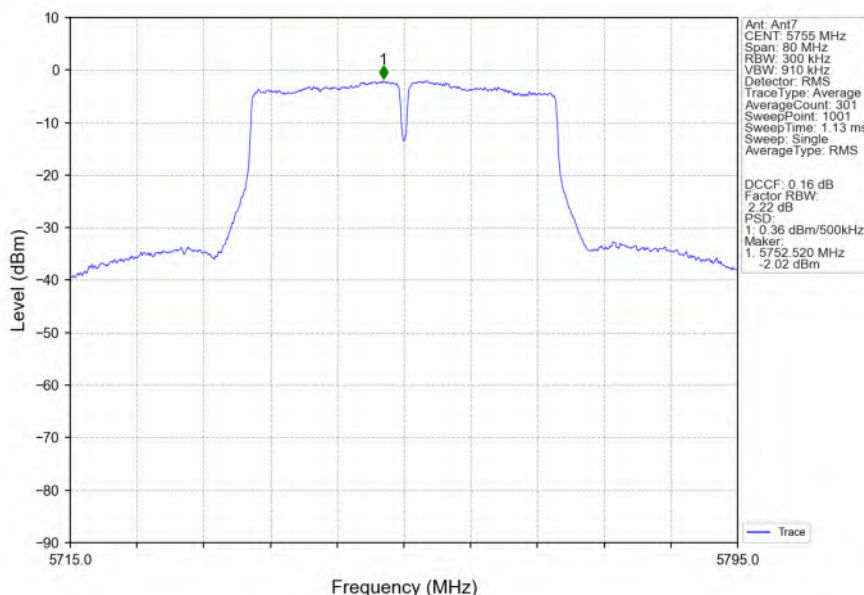
802.11ac(VHT40)_LCH_5755MHz_Ant7_NTNV
