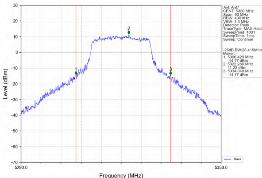
802.11n(HT20)_HCH_5320MHz_Ant7_NTNV
