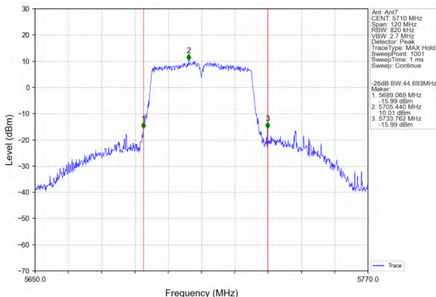
802.11n(HT40)_HCH_5710MHz_Ant7_NTNV
