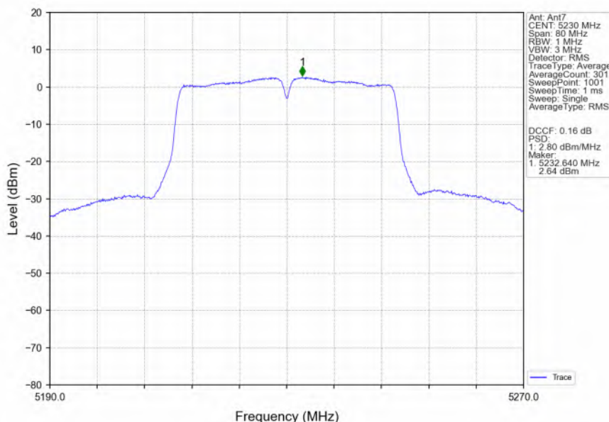
802.11n(HT40)_HCH_5230MHz_Ant7_NTNV
