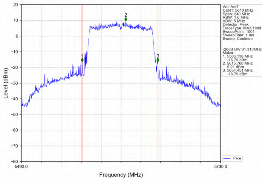
802.11ac(VHT80)_HCH_5610MHz_Ant7_NTNV
