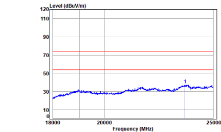
BT_DH5_TX_CH_39_Horizontal
