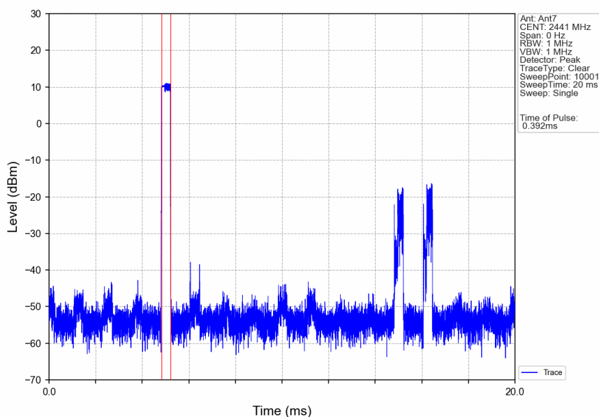
Pi/4DQPSK_2DH1_HOPP_Ant7_NTNV
