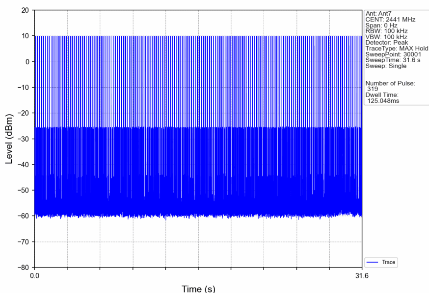
Pi/4DQPSK_2DH1_HOPP_Ant7_NTNV
