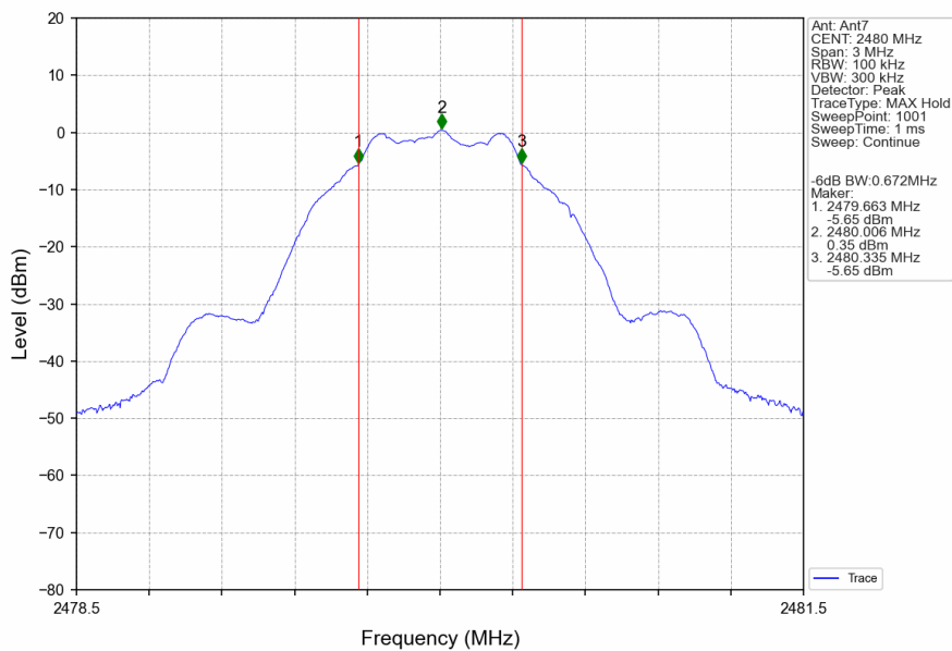
1M_HCH_2480MHz_Ant7_NTNV
