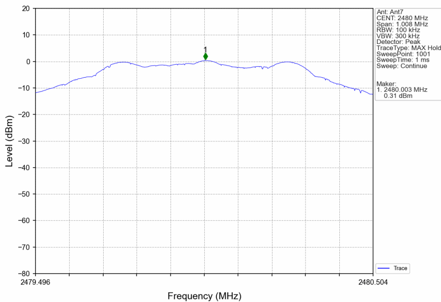
1M_HCH_2480MHz_Ant7_NTNV
