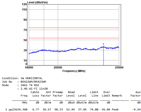
11n_20M_TX_CH_11_Horizontal
