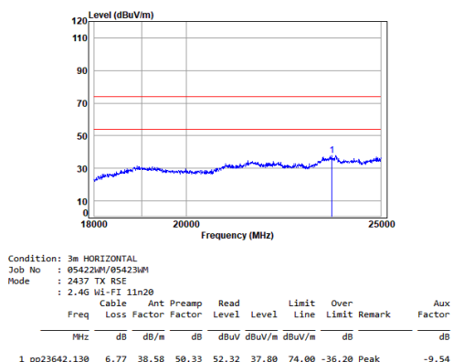
11n_20M_TX_CH_06_Horizontal
