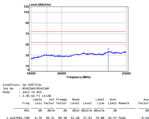
11n_20M_TX_CH_01_Vertical
