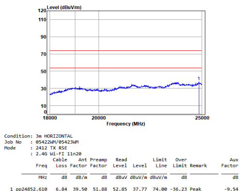
11n_20M_TX_CH_01_Horizontal
