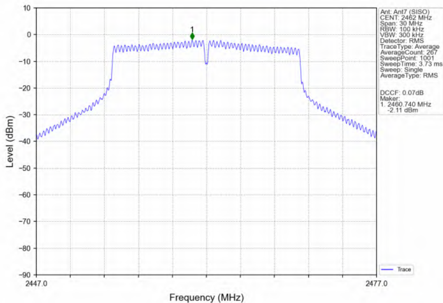
802.11g_HCH_2462MHz_Ant7 (SISO)_NTNV
