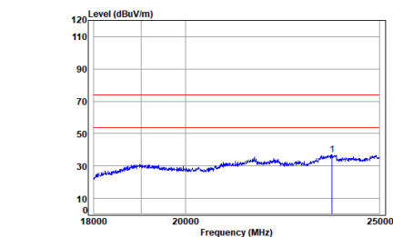
11g_TX_CH_06_Horizontal
