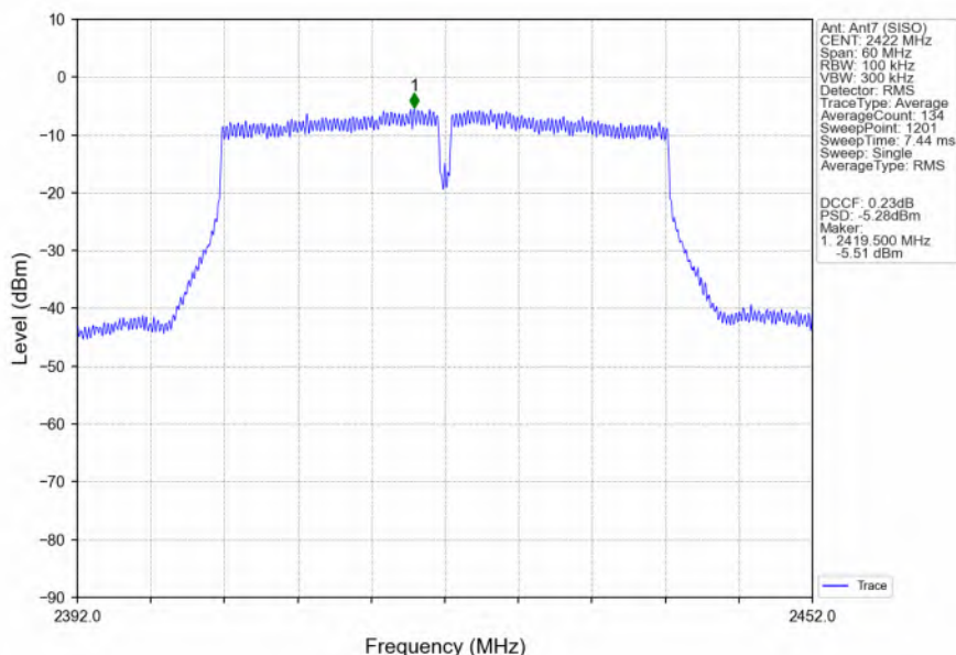
802.11n(HT40)_LCH_2422MHz_Ant7 (SISO)_NTNV
