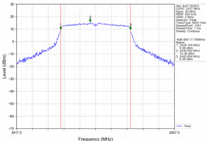
802.11n(HT20)_MCH_2437MHz_Ant7 (SISO)_NTNV
