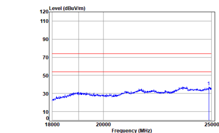
11g_TX_CH_11_Horizontal
