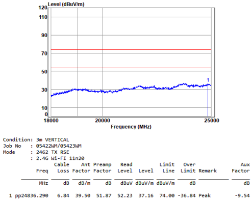
11n_20M_TX_CH_11_Vertical
