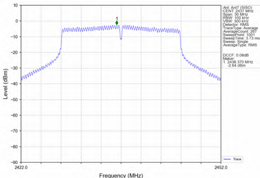
802.11n(HT20)_MCH_2437MHz_Ant7 (SISO)_NTNV
