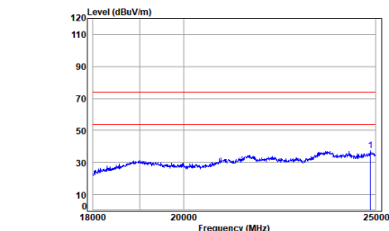
11b_TX_CH_11_Horizontal
