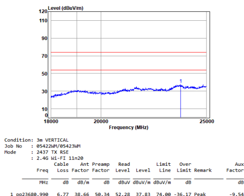
11n_20M_TX_CH_06_Vertical
