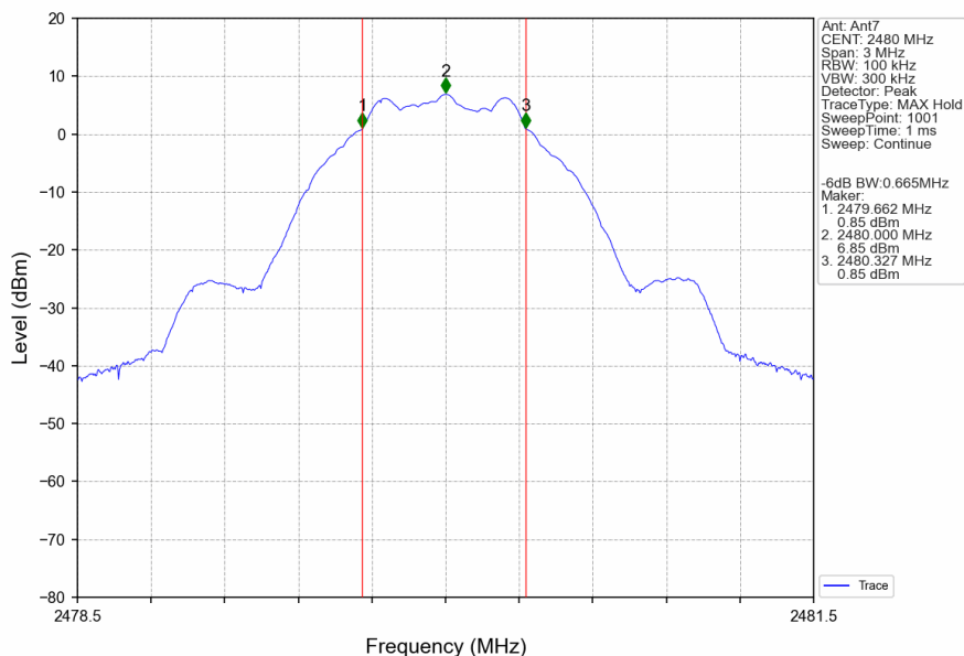
1M_HCH_2480MHz_Ant7_NTNV
