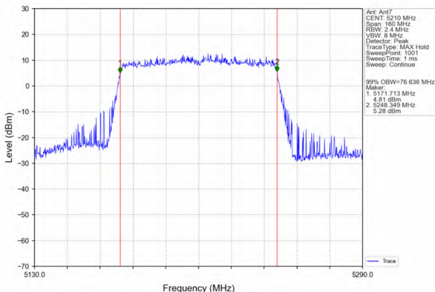
802.11ac(VHT80)_MCH_5210MHz_Ant7_NTNV
