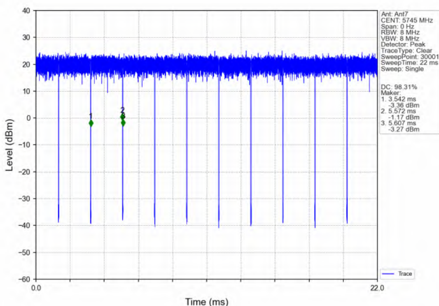
802.11a_LCH_5745MHz_Ant7_NTNV
