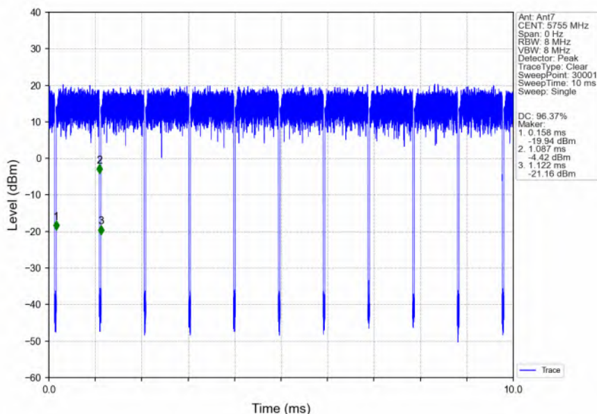
802.11n(HT40)_LCH_5755MHz_Ant7_NTNV
