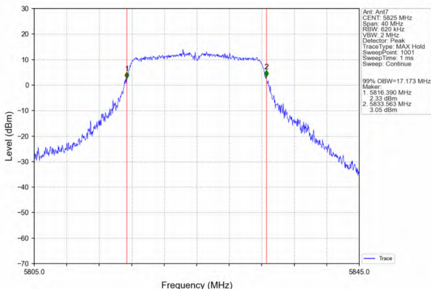
802.11a_HCH_5825MHz_Ant7_NTNV
