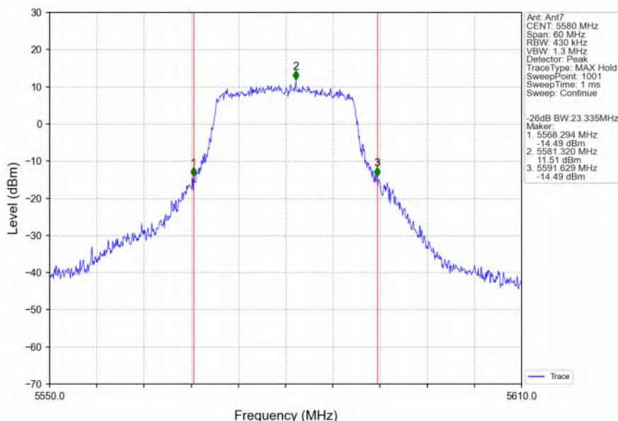
802.11n(HT20)_MCH_5580MHz_Ant7_NTNV
