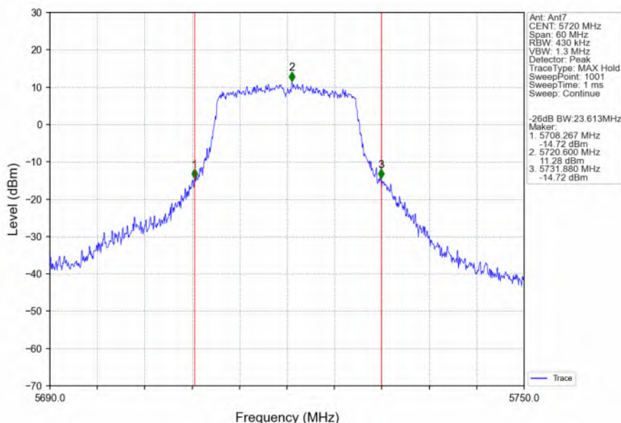
802.11n(HT20)_HCH_5720MHz_Ant7_NTNV
