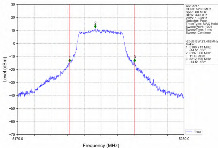
802.11a_MCH_5200MHz_Ant7_NTNV
