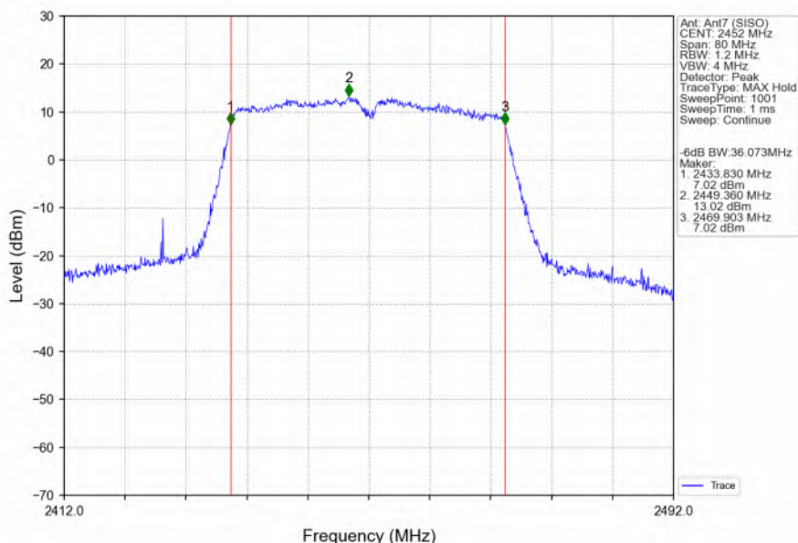
802.11n(HT40)_HCH_2452MHz_Ant7 (SISO)_NTNV
