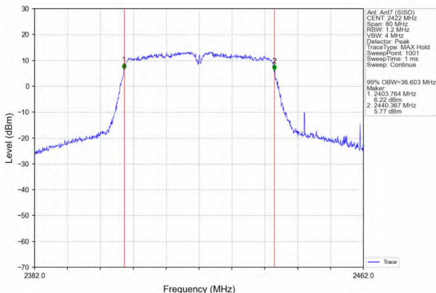
802.11n(HT40)_LCH_2422MHz_Ant7 (SISO)_NTNV
