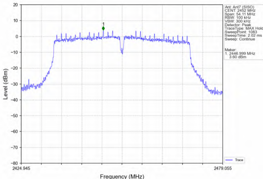
802.11n(HT40)_HCH_2452MHz_Ant7 (SISO)_NTNV
