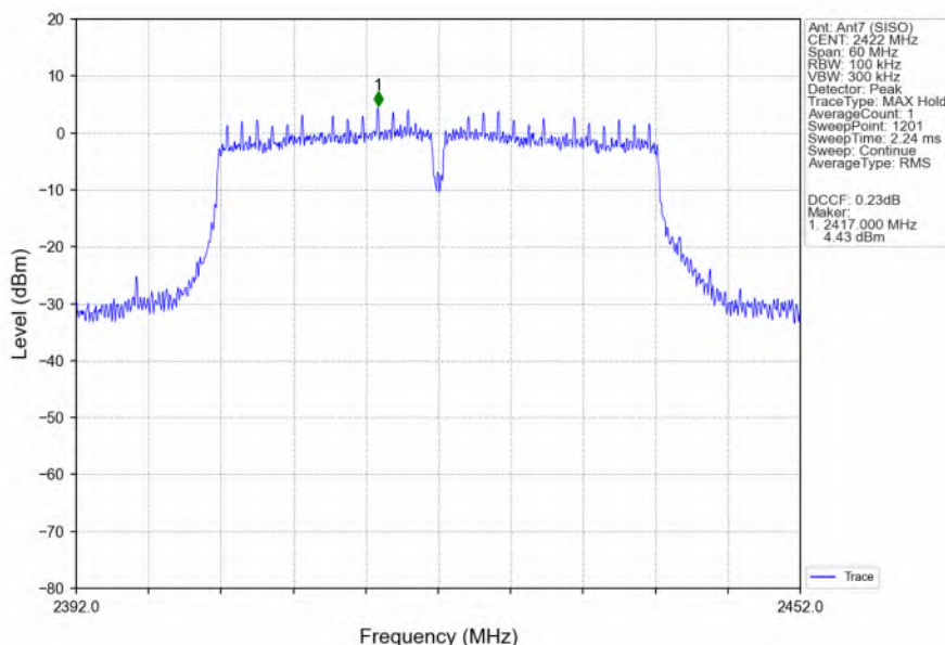
802.11n(HT40)_LCH_2422MHz_Ant7 (SISO)_NTNV
