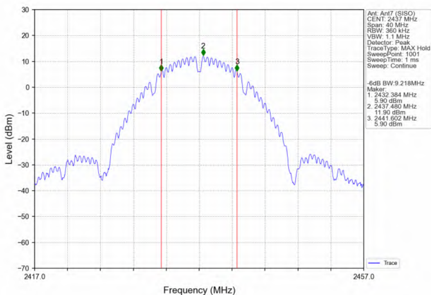
802.11b_MCH_2437MHz_Ant7 (SISO)_NTNV
