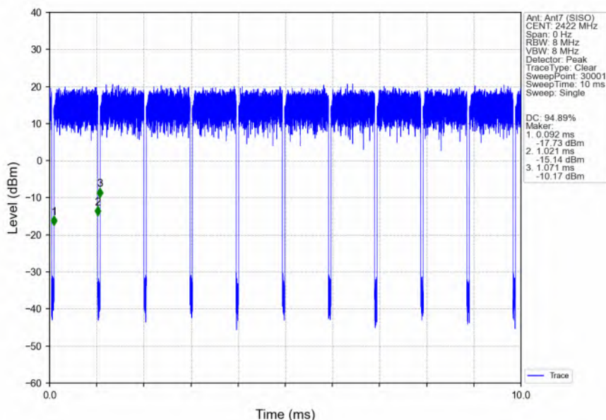
802.11n(HT40)_LCH_2422MHz_Ant7 (SISO)_NTNV
