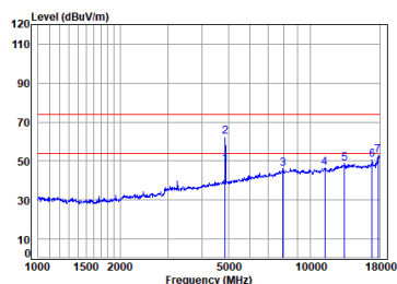
11g_TX_CH_06_Horizontal
