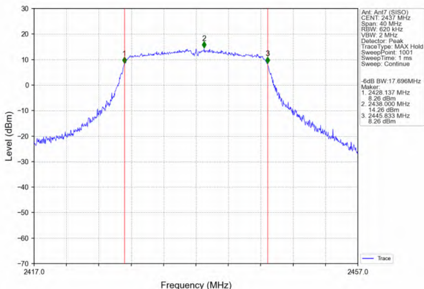
802.11n(HT20)_MCH_2437MHz_Ant7 (SISO)_NTNV
