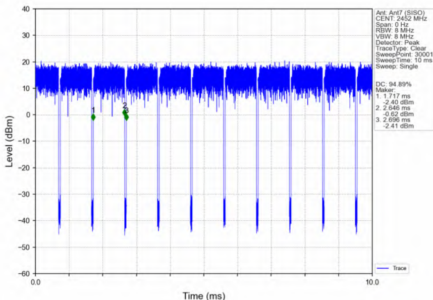
802.11n(HT40)_HCH_2452MHz_Ant7 (SISO)_NTNV
