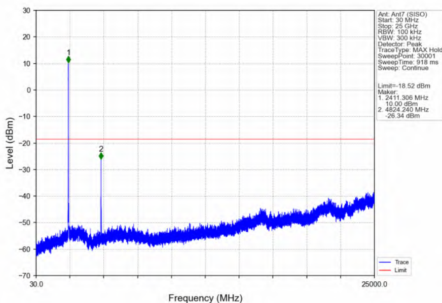
802.11b_LCH_2412MHz_Ant7 (SISO)_NTNV
