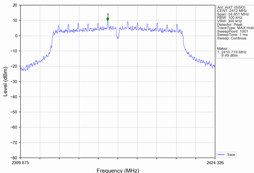
802.11g_LCH_2412MHz_Ant7 (SISO)_NTNV
