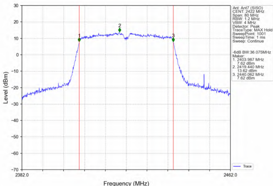
802.11n(HT40)_LCH_2422MHz_Ant7 (SISO)_NTNV
