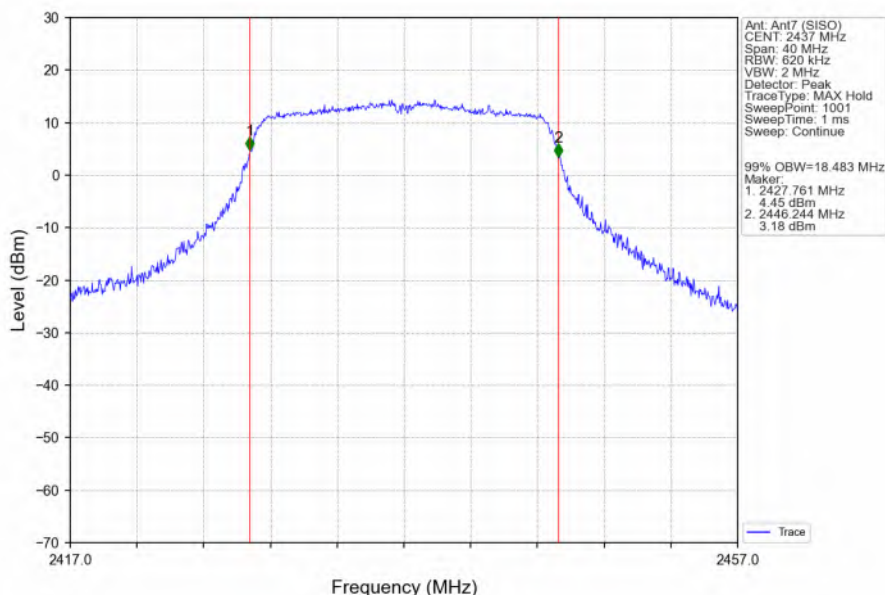
802.11n(HT20)_MCH_2437MHz_Ant7 (SISO)_NTNV
