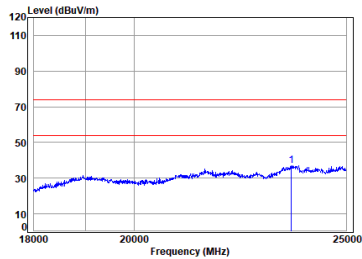
BT_DH5_TX_CH_39_Horizontal
