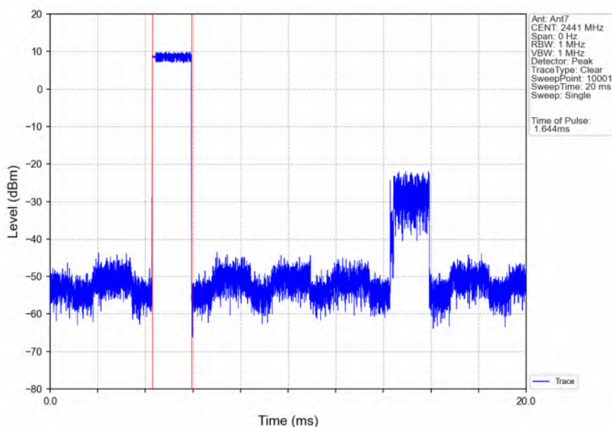
Pi/4DQPSK_2DH3_HOPP_Ant7_NTNV
