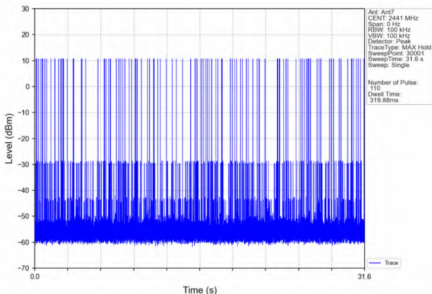
GFSK_DH5_HOPP_Ant7_NTNV
