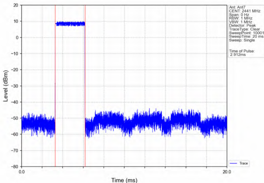
Pi/4DQPSK_2DH5_HOPP_Ant7_NTNV
