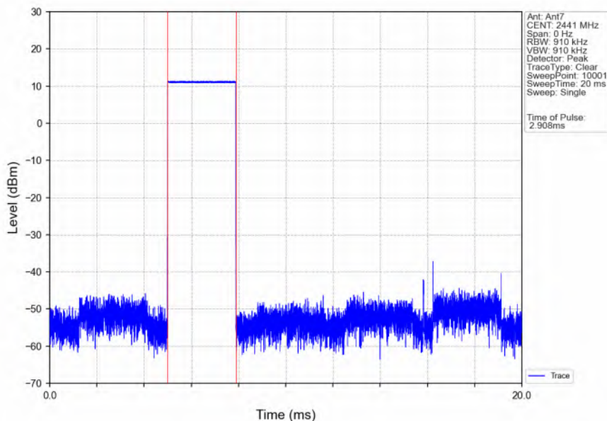
GFSK_DH5_HOPP_Ant7_NTNV
