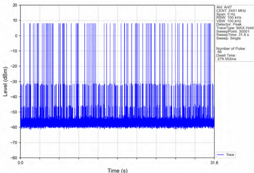
Pi/4DQPSK_2DH5_HOPP_Ant7_NTNV
