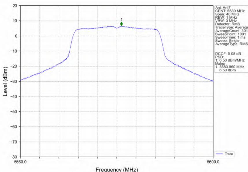
802.11n(HT20) MCH 5580MHz Ant7 NTN
