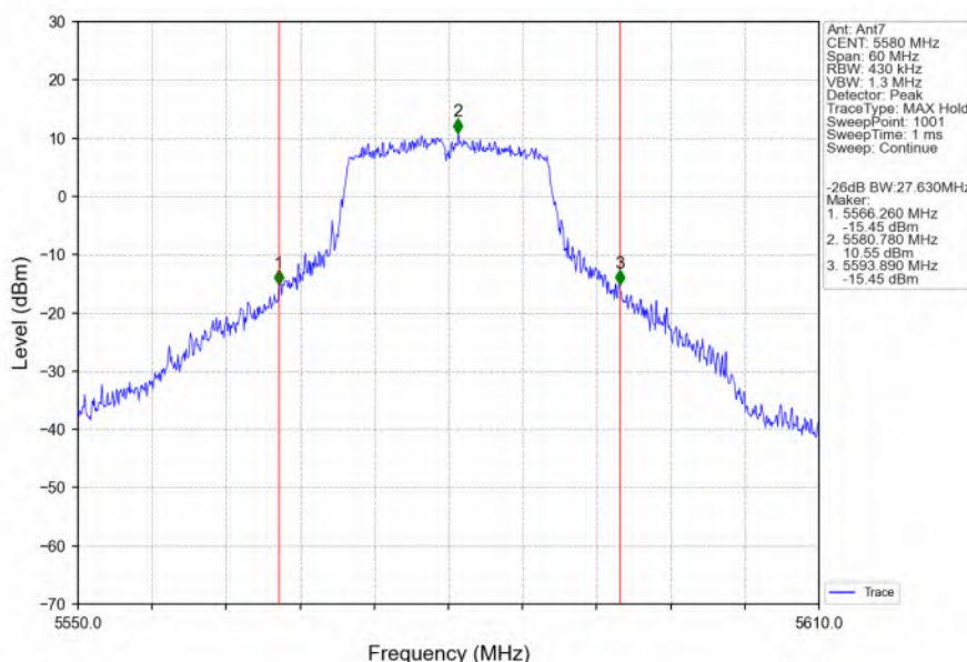
802.11a_MCH_5580MHz_Ant7_NTNV
