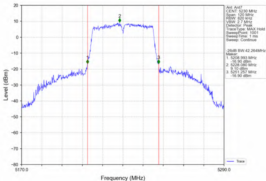
802.11ac(VHT40) HCH 5230MHz Ant7 NTN
