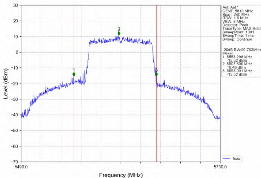
802.11ac(VHT80) HCH 5610MHz Ant7 NTN
