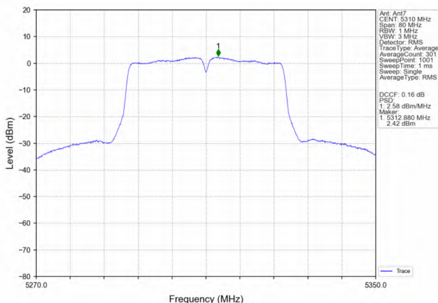
802.11ac(VHT40) HCH 5310MHz Ant7 NTN
