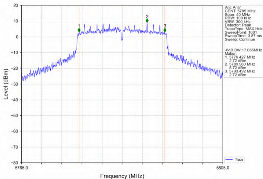
802.11ac(VHT20) MCH 5785MHz Ant7 NTN
