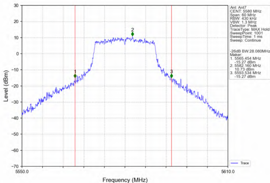
802.11n(HT20) MCH 5580MHz Ant7 NTN
