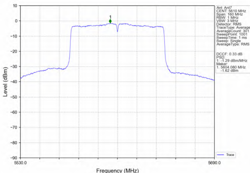
802.11ac(VHT80) HCH 5610MHz Ant7 NTN
