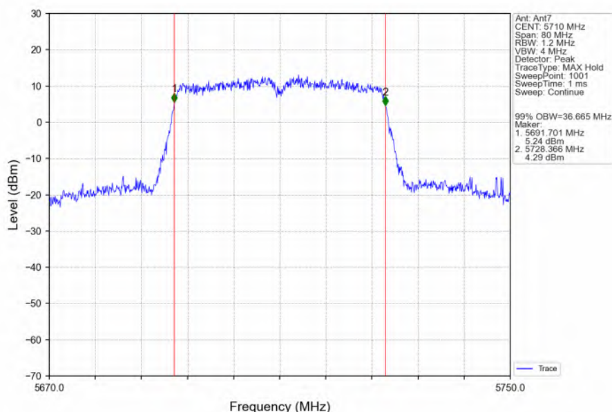
802.11n(HT40)_HCH_5710MHz_Ant7_NTNV
