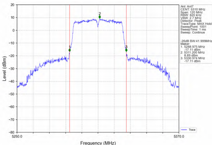
802.11n(HT40) HCH 5310MHz_Ant7_NTNV
