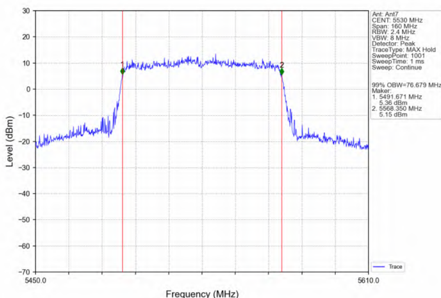
802.11ac(VHT80)_LCH_5530MHz_Ant7_NTNV
