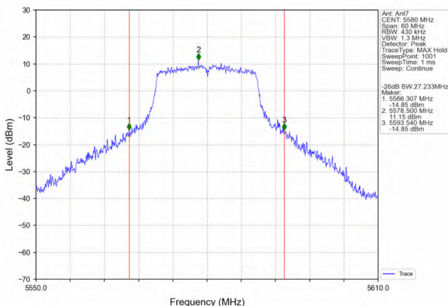
802.11ac(VHT20) MCH 5580MHz Ant7 NTN
