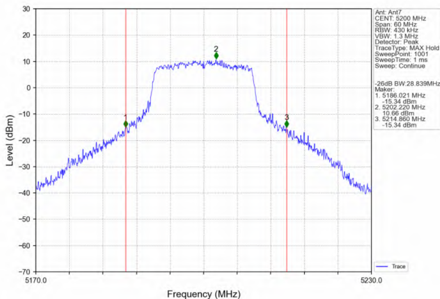
802.11n(HT20) MCH 5200MHz_Ant7_NTNV
