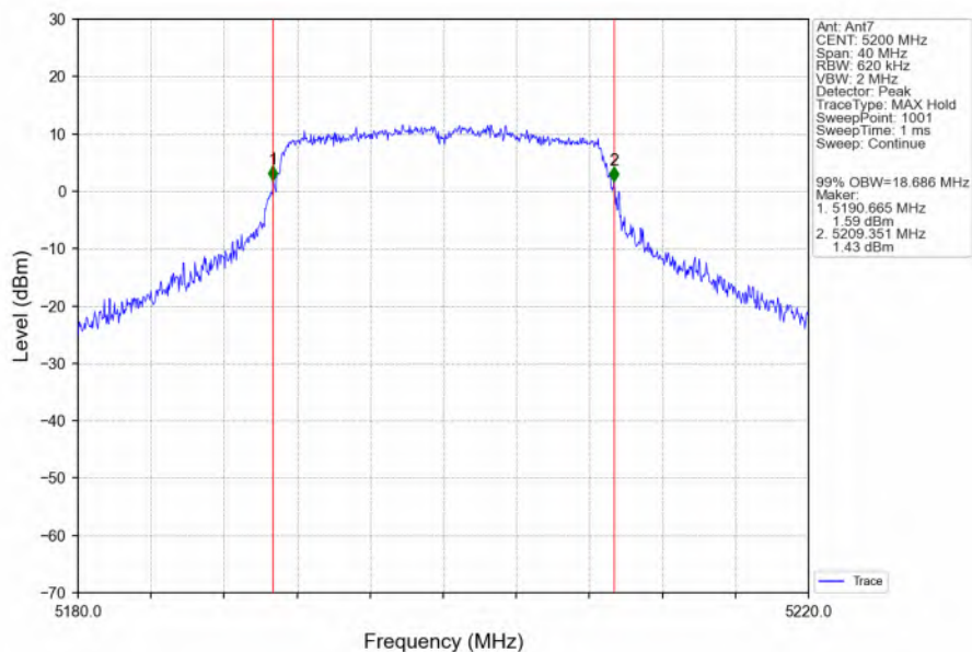
802.11ac(VHT20) MCH 5200MHz Ant7 NTN
