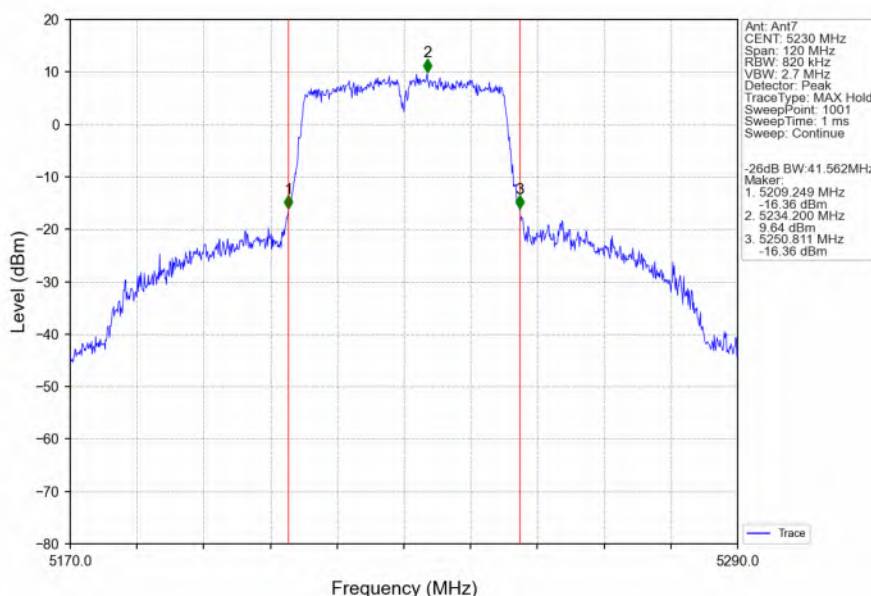
802.11n(HT40) HCH 5230MHz_Ant7_NTNV
