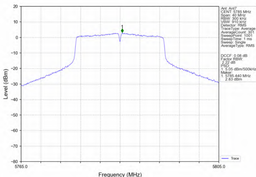
802.11n(HT20) MCH 5785MHz Ant7 NTN
