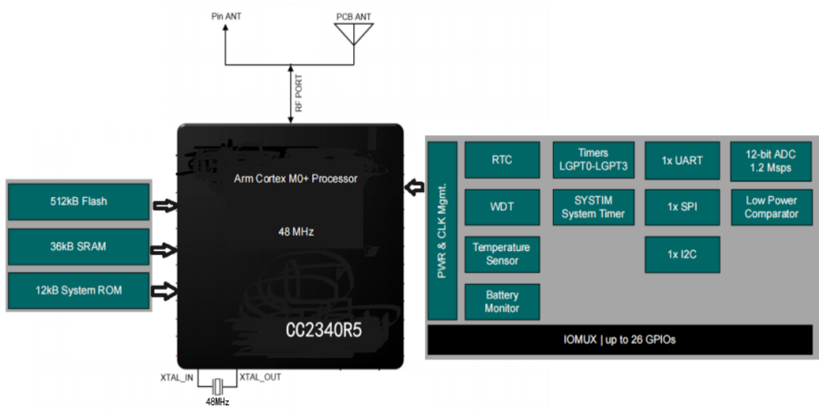
Figure1 : Block Digrm
