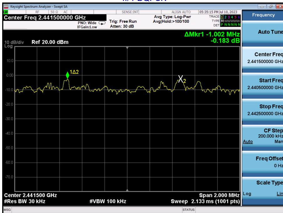
\pi/4 -DQPSK
