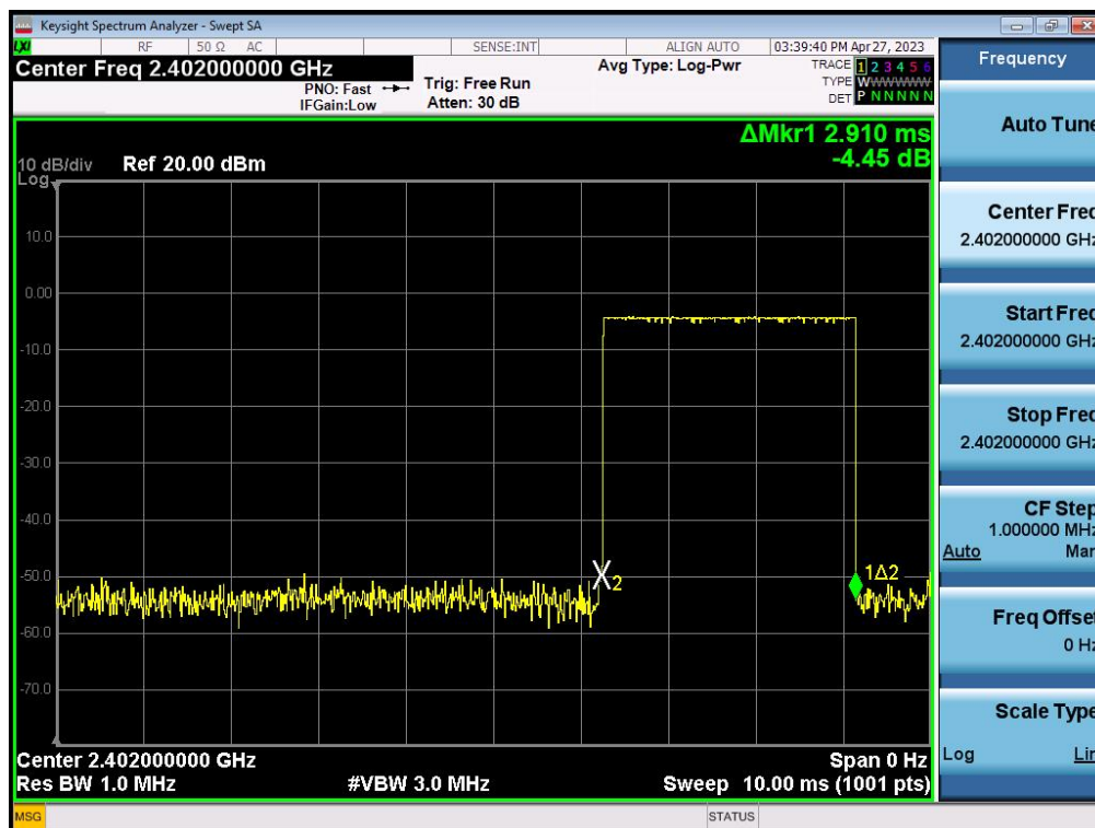
GFSK 2402MHz
