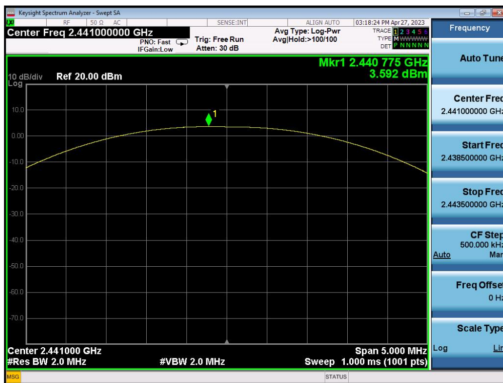
GFSK 2441MHz
