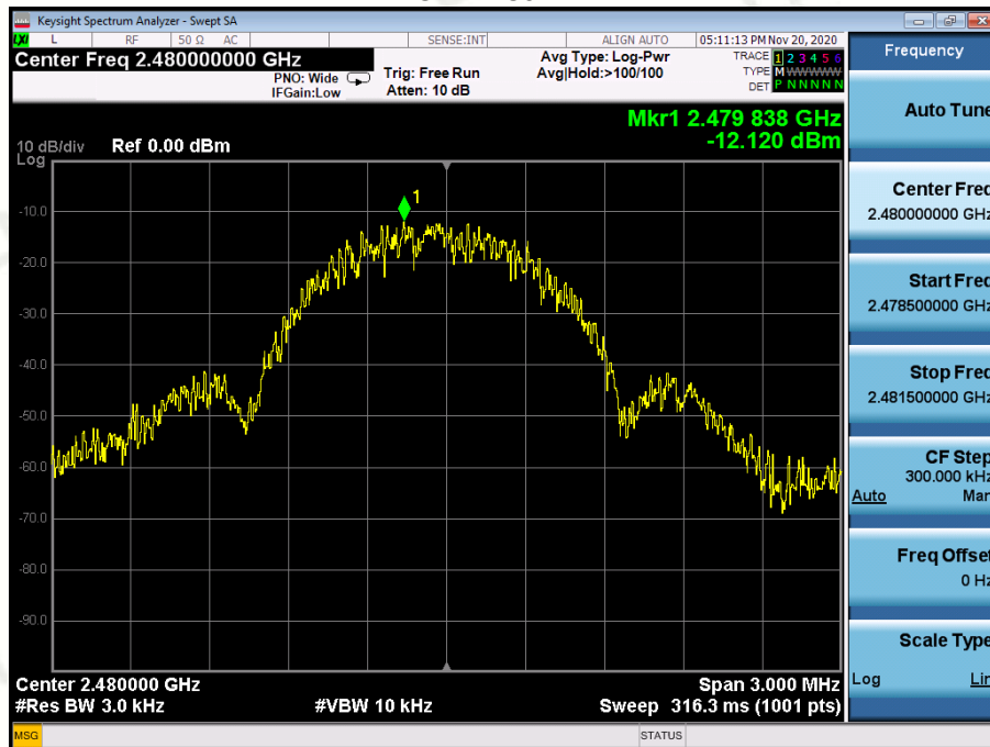
CH: 2480MHz
