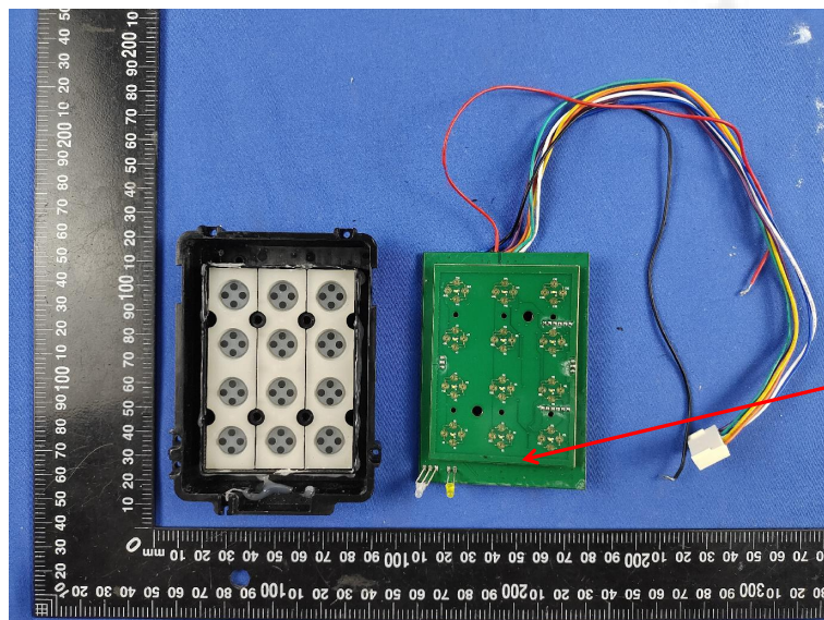
RFID Antenna
