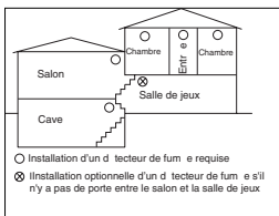
Fig 5. Installation dans une maison
