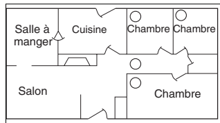
Fig 2. Emplacement des détecteurs dans des maisons ayant une seule chambre à coucher sur un étage
