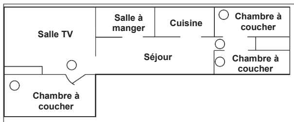
Figure 6 - Emplacement des détecteurs dans les habitations comportant plusieurs ensembles de chambres à coucher ou plusieurs chambres à coucher sur plusieurs étages
