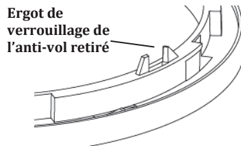
Figure 17 - Ergot de verrouillage de l'anti-vol retiré
