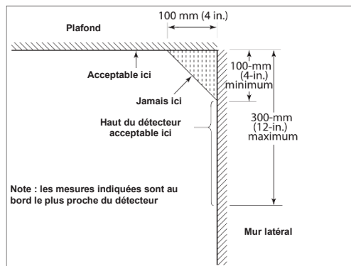
Figure 9 - Exemple de montage correct des détecteurs
