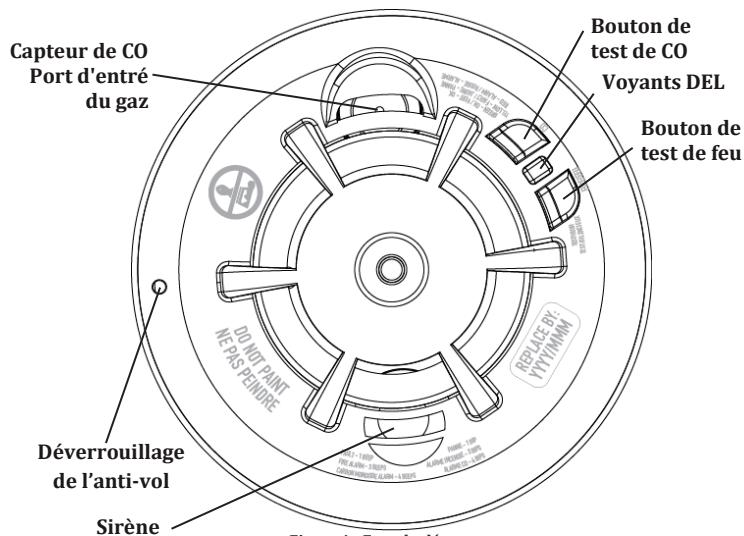
Figure 1 - Face du détecteur
