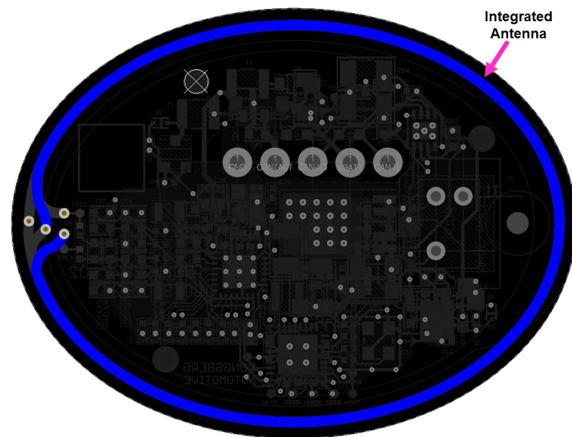
Bottom Layer
