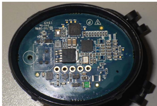
Bottom PCB
