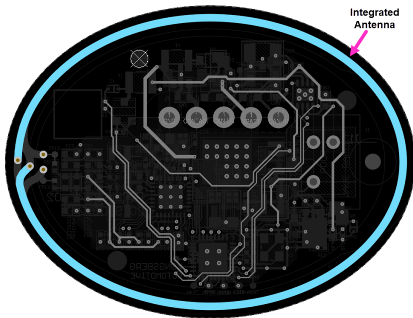
Inner Layer 2
