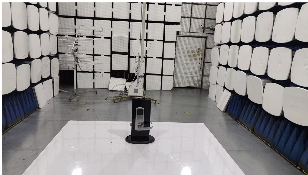
Fig. 2 (30MHz~1GHz)
