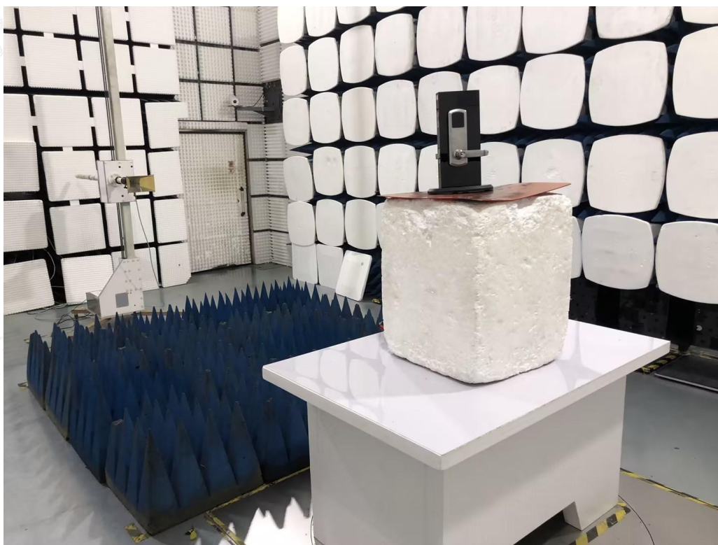
Fig. 2 (Above 1GHz)
