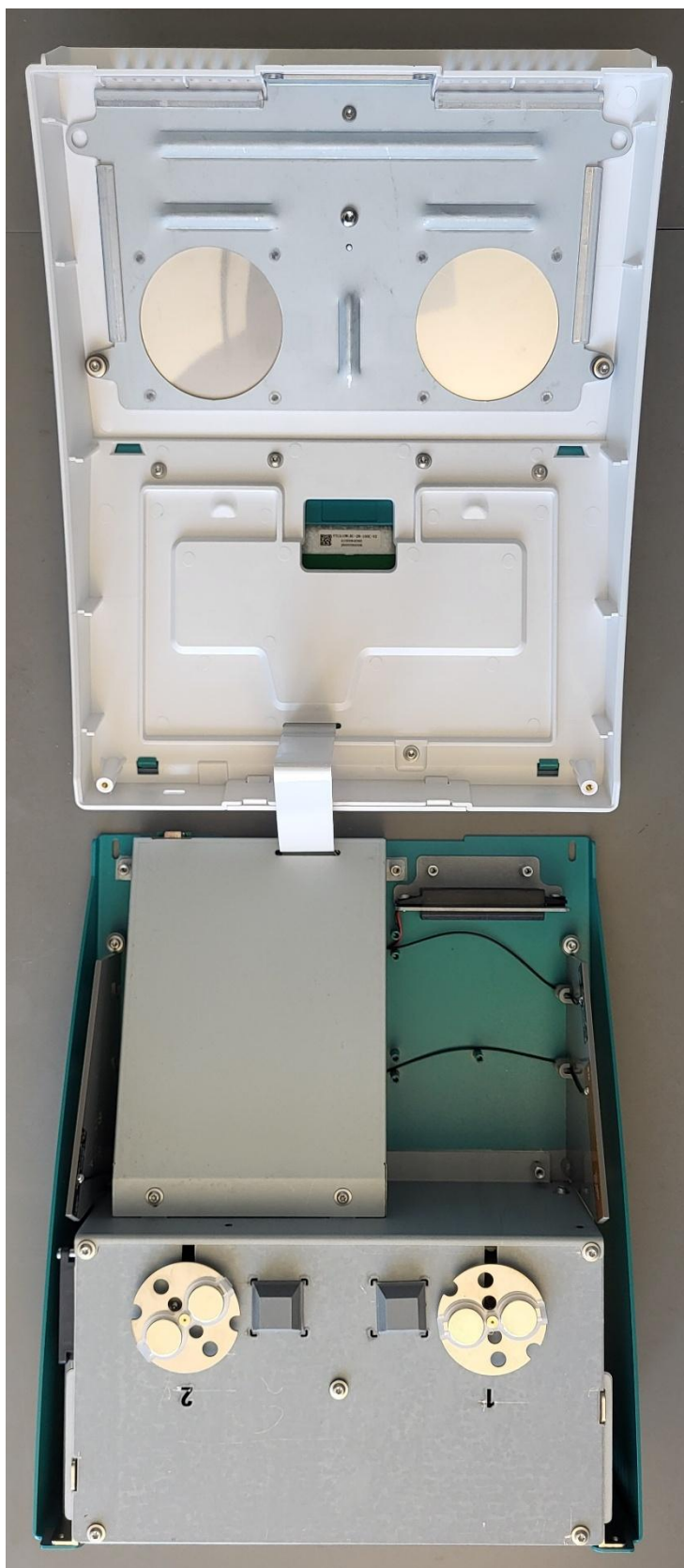
IONIC Titrator (top view)
