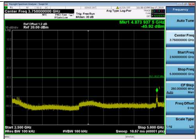
802.11g,2437MHz,Ant0,Plot 4,2500MHz~5000MHz
