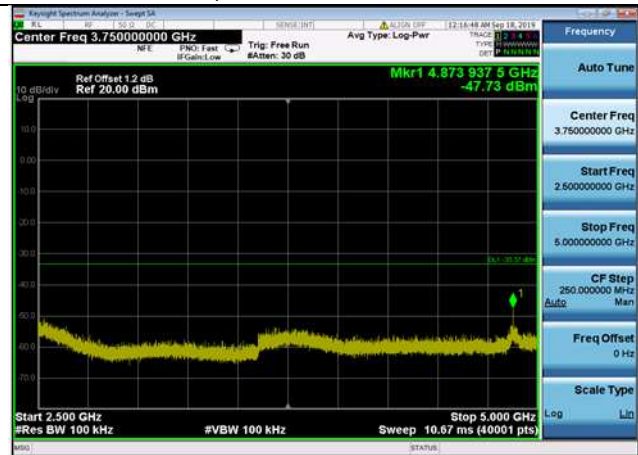
802.11n(HT40),2437MHz,Ant0,Plot 4,2500MHz~5000MHz
