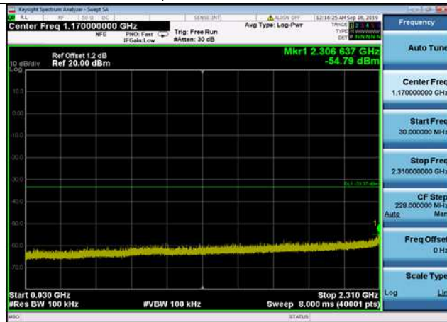
802.11n(HT40),2437MHz,Ant0,Plot 3,30MHz~2310MHz
