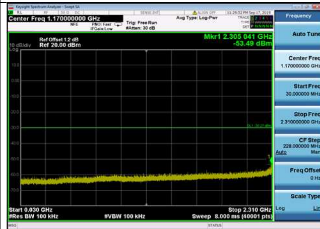
802.11g,2437MHz,Ant0,Plot 3,30MHz~2310MHz
