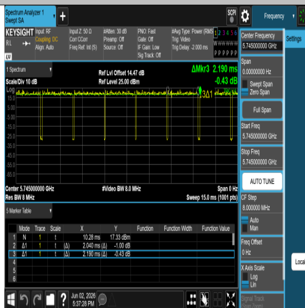
NTNV-11A-Ant1-5745
