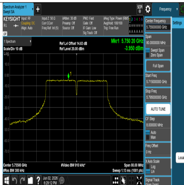
11N40ISO-Ant1-5755-PASS
