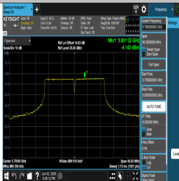
11N40ISO-Ant1-5795-PASS
